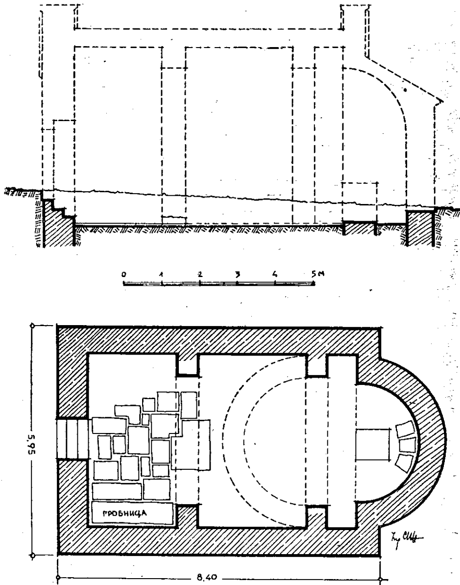
Сл. 111. — Основа и подужни пресек цркве св. Јована Претече у Студеници
