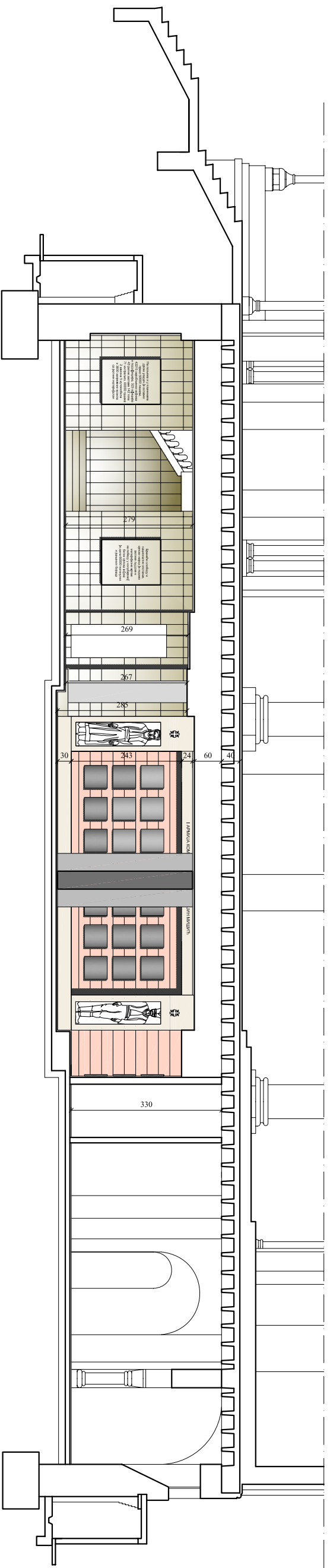
Попречни пресек 2-2 Р 1: 100
