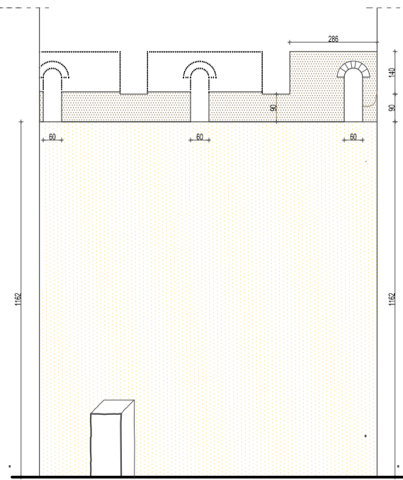
УНУТРАШЊИ ИЗГЛЕД БЕДЕМА
