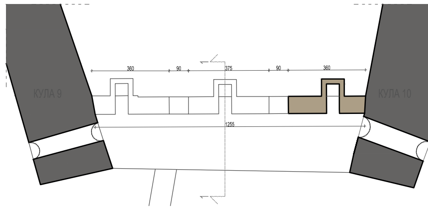
УНУТРАШЊИ ИЗГЛЕД БЕДЕМА
