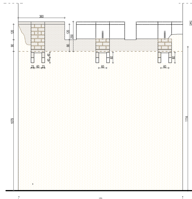
СПОЉАШЊИ ИЗГЛЕД БЕДЕМА
