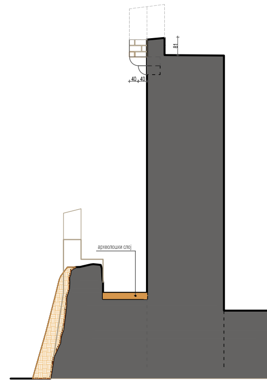
ПРЕСЕК 1 - 1
