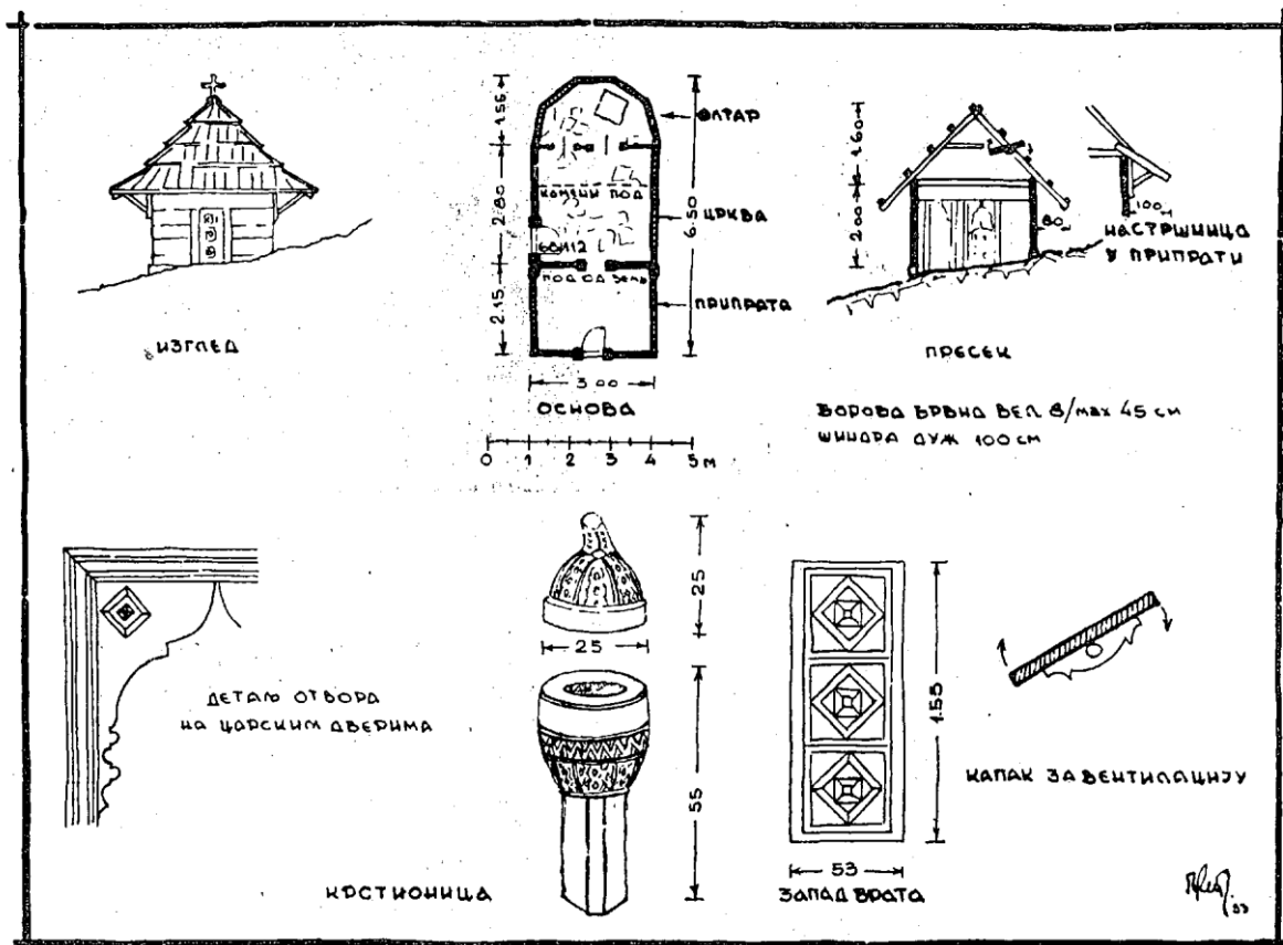
Изглед, пресеци и детаљи цркве брвнаре у Кућанима
