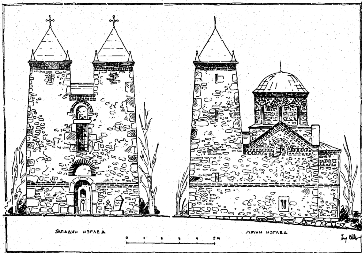
Сл. 8. — Пројект за рестаурацију Доње Каменице
