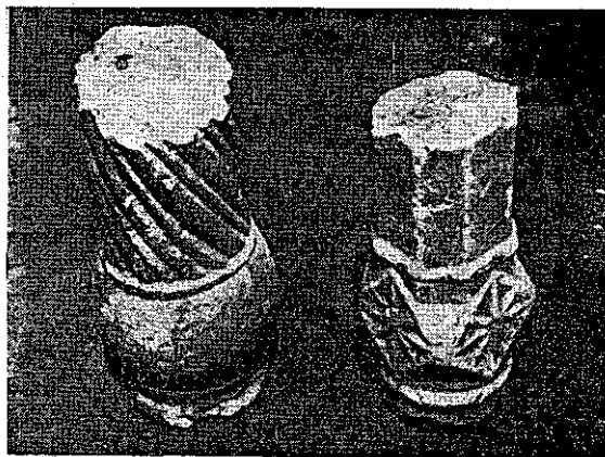
Сл. 72. — Два дела стубова чирака
