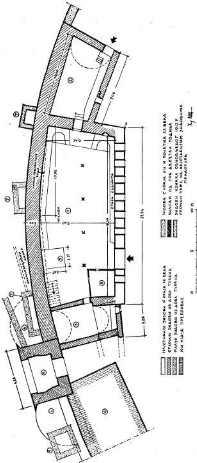
Сл. 87. — Основа трпезарије у Студеници пре почетка радова: 1 — Сала за обед, 2 — Подрум, 3 — Пушница, 4 — Места где су се налазиле полукружне куле, 5 — Основа четвртасте куле која почива на полукружним кулама, 6 — Конак з XIX века, обновљен 1912 године, 7 — Остаци порушених клозета, 8 — Магацин — одељење саграђено пре десетак година, 9 — Нова зидана већ, порушена приликом реставрације
