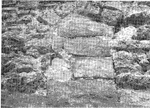
Сл. 10. Зазидана ниша на кубету после обијања малтера. — Fig. 10. Niche murée de la coupole après l'enlèvement du mortier.
