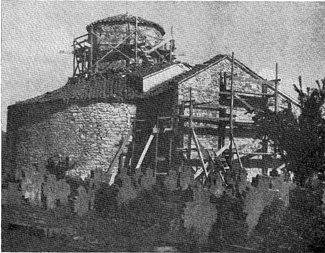
Сл. 8. Северозападни део у току радова. — Fig. 8. Face nord-ouest au cours des travaux.
