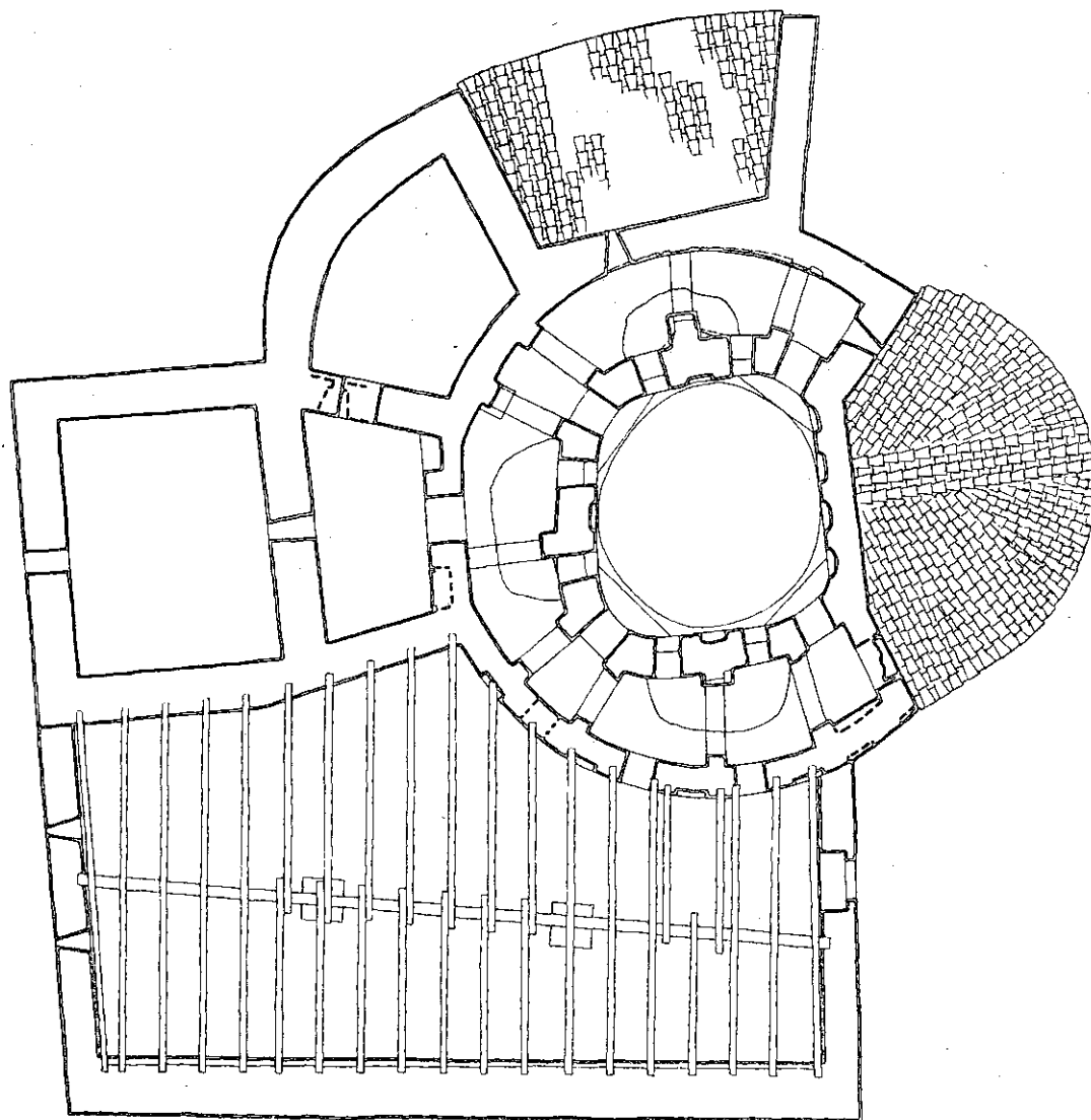
Сл. 2. Основа у висини галерије после конзервације. Нише и отвори на галерији били су зазидани, а на једној страни галерије нису постојали попречни луци пре конзервације. — Fig. 2. Plan à la hauteur de la galerie. Les niches et les baies de la galerie avaient été murées, et d'un côté de la galerie les arcs transversaux n'existaient pas avant la conservation.
