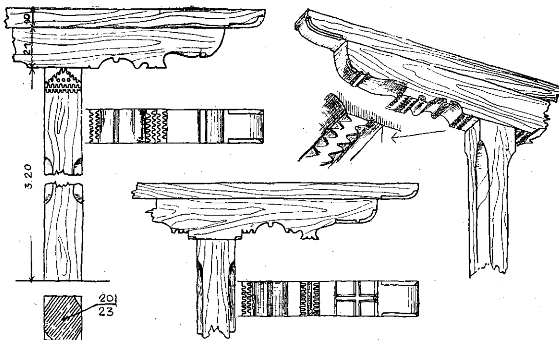
Сл. 9. Дрвени ступци и јастуци из 19. века, део кровне конструкције јужног дозиданог простора. — Fig. 9. Piliers et coussinets en bois datant du XIX e siècle, une partie de la toiture surmontant la construction ajoutée du côté du sud.
