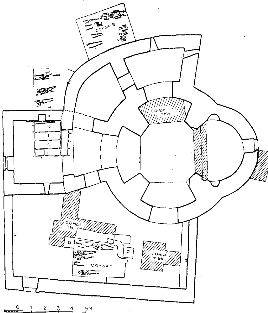
Сл. 1. Основа цркве и положај сонди. Сонде I и II су из 1957 године, а сонда III из 1958. год. Остале сонде су из 1956. год. — Fig. 1. Plan de l'église et emplacements des sondes. Les sondes I et II furent pratiquées en 1957 et la sonde III en 1958; toutes les autres en 1956.
