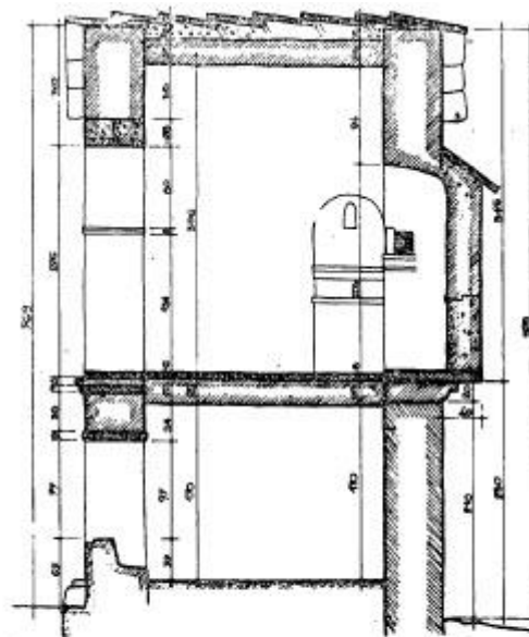
5. Долац, изнад Студенице, црква св. Богородице, подужни пресек 5. Dolac, au-dessus de Studenica, église de la Sainte-Vierge, la coupe longitudinale
