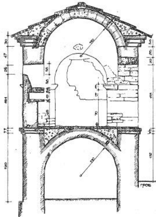
3. Долац, изнад Студенице, црква св. Богородице, попречни пресек 3. Dolac, au-dessus de Studenica, église de la Sainte-Vierge, la coupe transversale.
