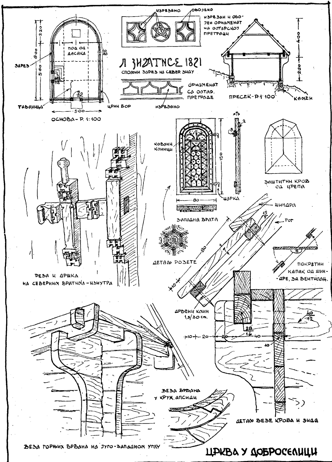
113. Eglise de «Dobroselica»: Plan; Details: ornaments, inscriptions; Coupe; Chevillette; Porte d'entrée; Schème de la toiture; Détails de la charpente.
