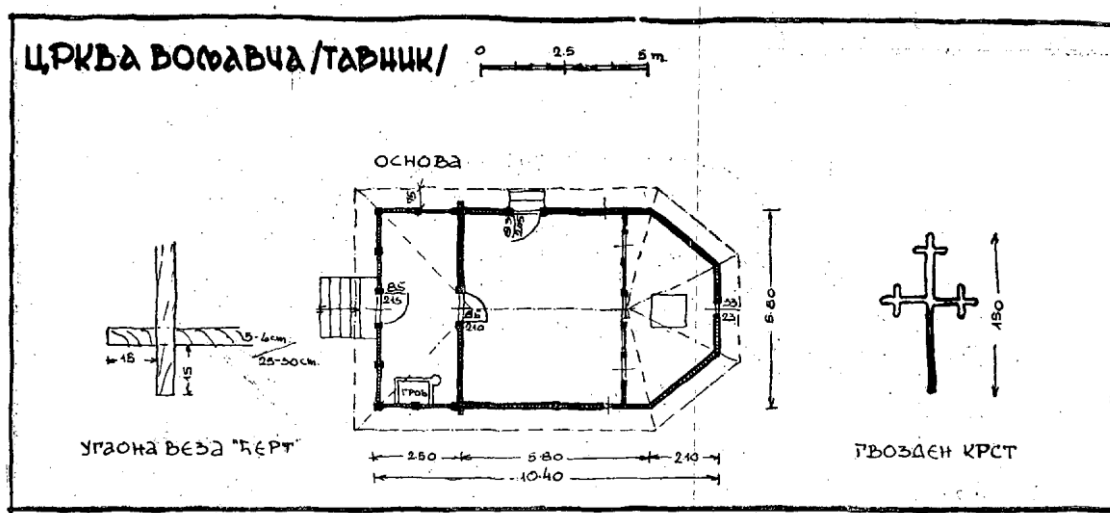
104. »Voljavča«, église de »Tavnik«: Jointurje; Plan; Croix en fer forgé.
