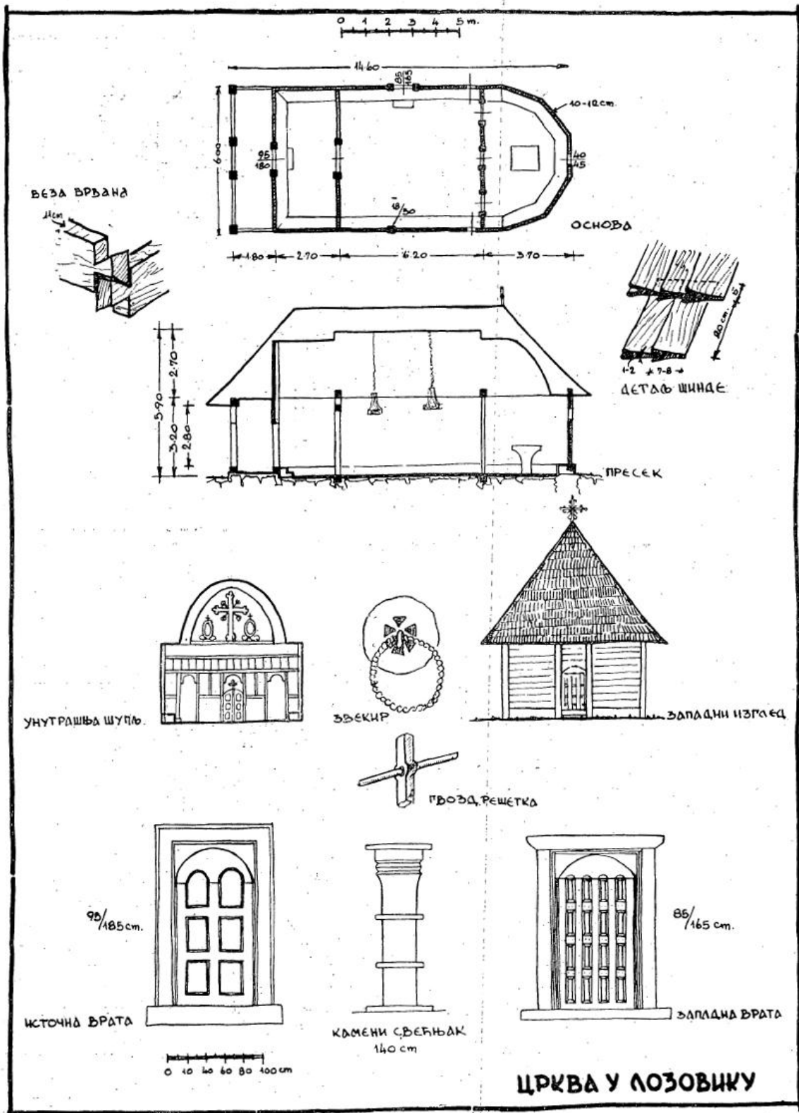
122. Eglise de «Lozovik»: Plan; Coupes; Schème de l'iconostase; Façade; Portes d'entrée; Jointures; Echantôles; Fer forgé; Chandelier de pierre.
