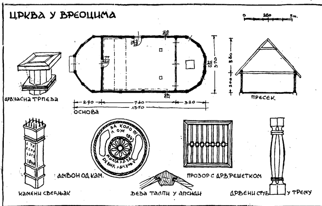
107. Eglise de »Vreoci«: Autel de bois; Plan; Coupe; Chandelier et ambon de pierre; Fenêtre à grille de bois; Jointure de madriers; Pilier de bois.
