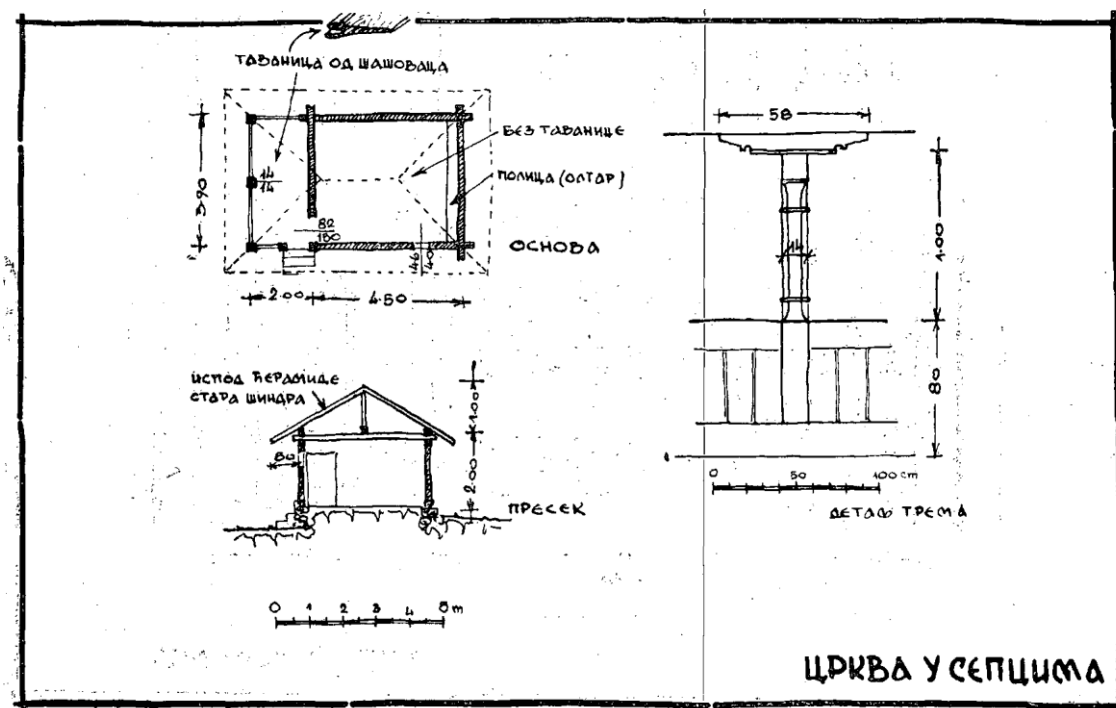
140. Eglise de »Sepci«: Plan; Coupe; Pilier du portique.
