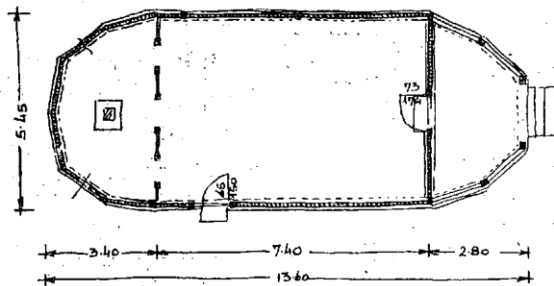
ОСНОВА
