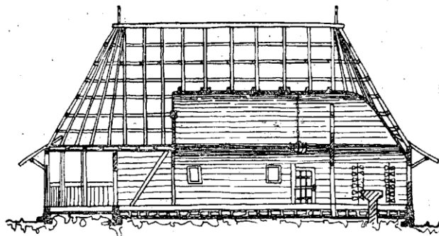
ПОДУЖНИ ПРЕСЕК
