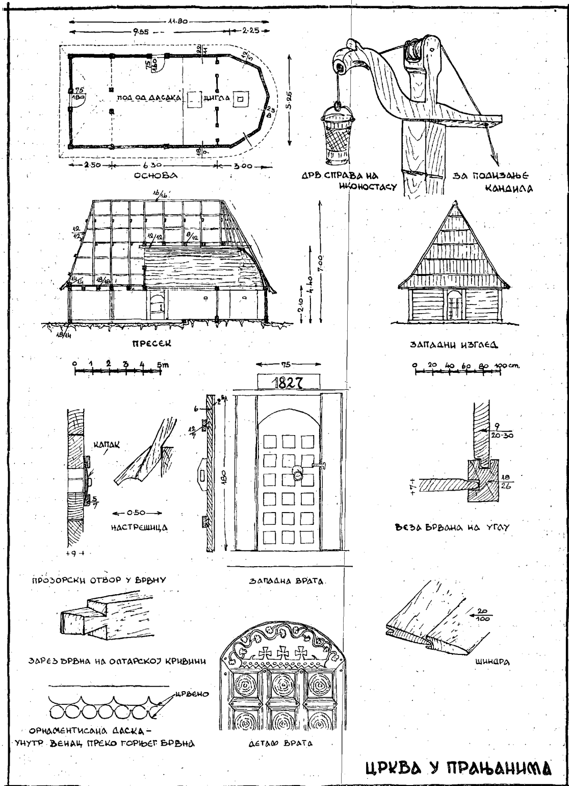
134. Eglise de «Pranjani»: Plan; Suspension à poulie pour veilleuse; Coupe; Façade; Détail de charpente; Porte d'entrée; Jointure; Latte ornementée; Détail de la porte; Echandoles.
