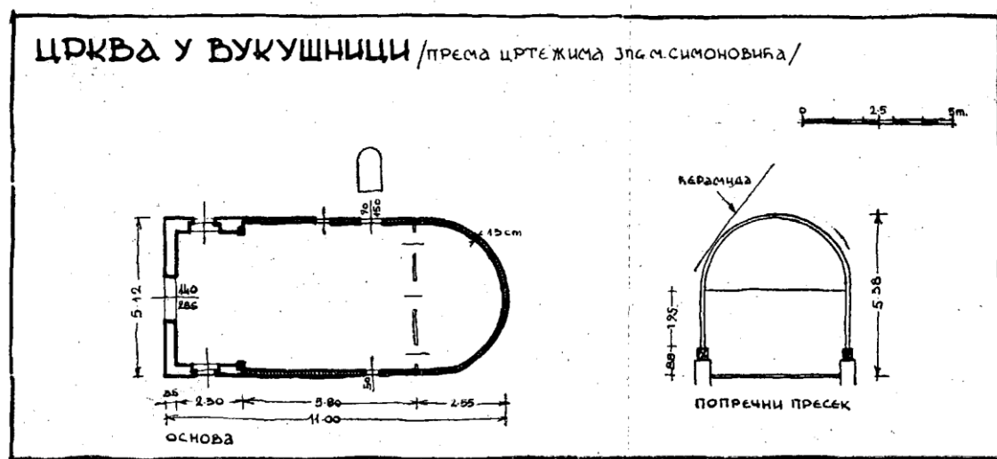
108. Eglise de »Vukušnica«, Plan; Coupe (D'après les esquisses de l'ing. M. Simonović).
