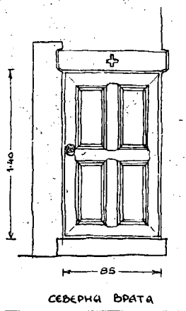
135. Eglise de »Radijevići«: Plan de l'église et de son sous-sol; Coupe; Façade; Porte d'entrée; Autel de pierre; Pilier de la cave; Fenêtre.
