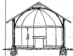
ПОПРЕЧНИ ПРЕСЕК
