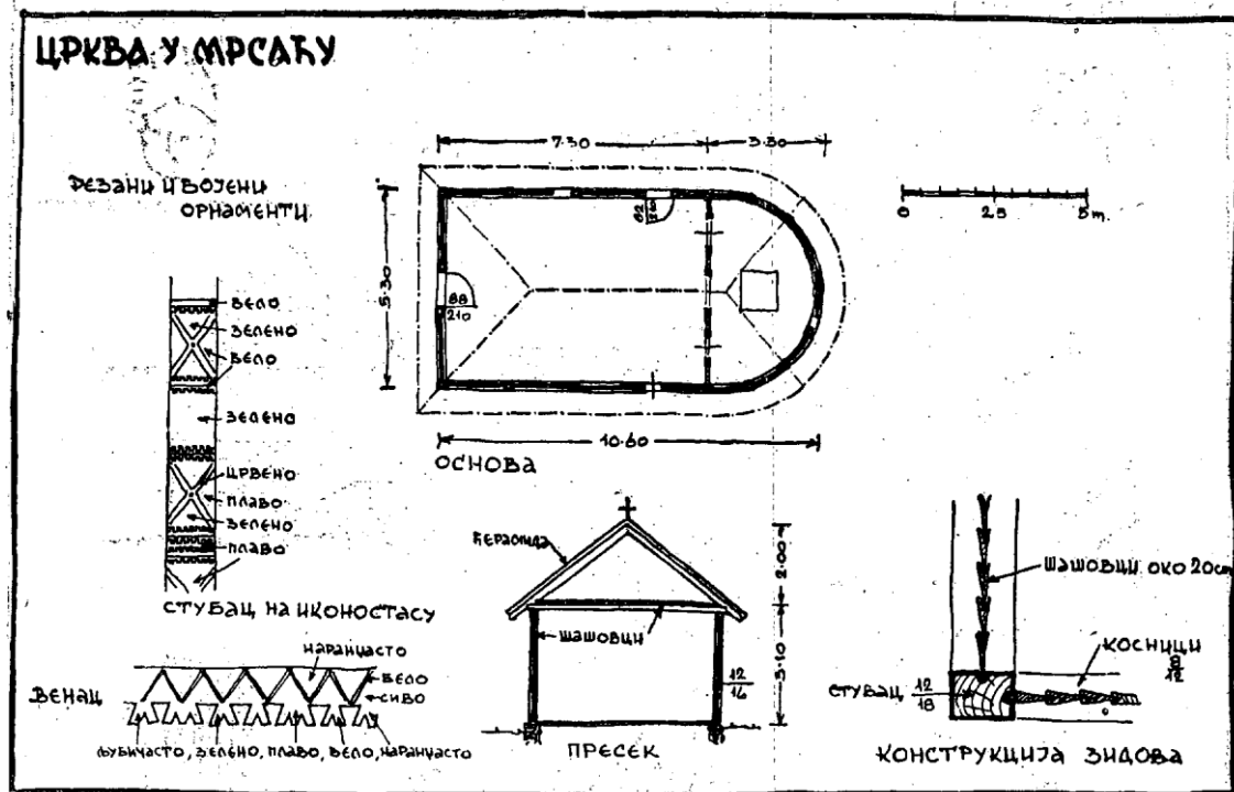
126. Eglise de «Mrsac»: Plan; Coupe; Ornementation colorée; Jointure d'angle.
