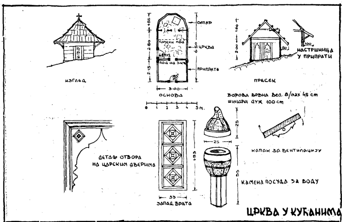
121. Eglise de «Kučani»: Façade; Plan; Co upre; Détail de la baie de l'iconostase; Porte d'entrée; Bénitier; Volet à ventilation.
