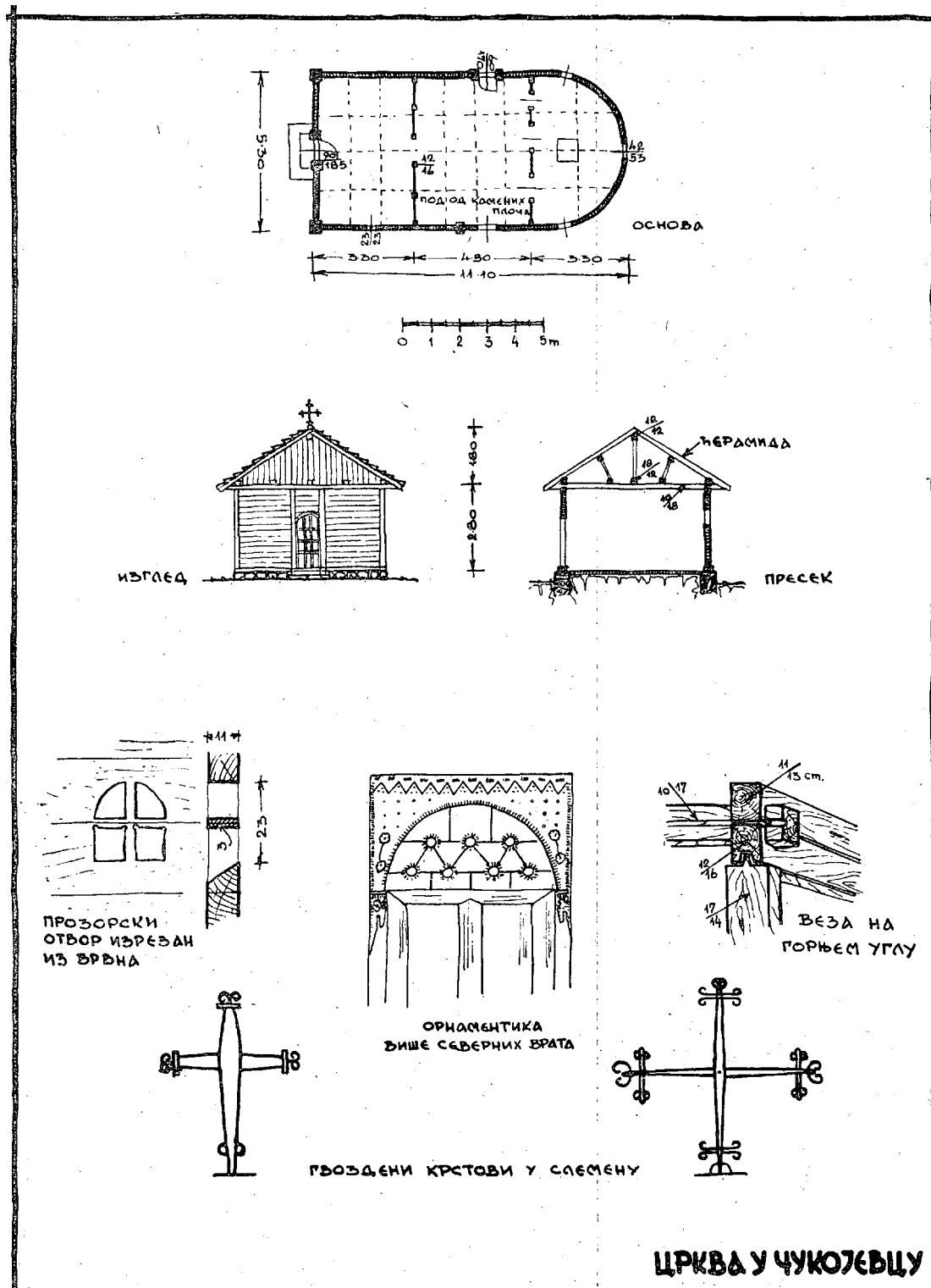
150. Eglise de «Cukojevac»: Plan; Façade; Co upe; Ouverture de fenêtre entaillée dans les madriers; Ornaments au-dessus de la porte d'entrée; Jointure; de l'entablement; Croix en fer forgé.
