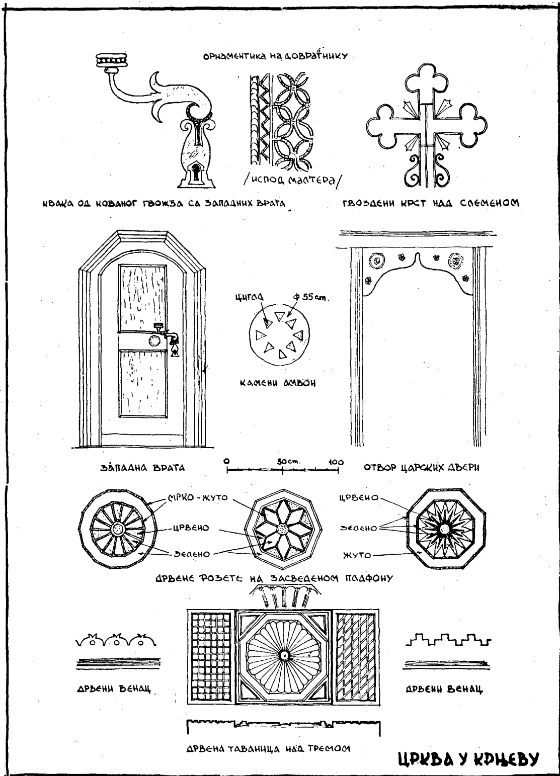
120. Eglise de «Krnjevo»: Poignée; Ornementation; Croix en fer forgé; Portes d'entrée; Ambon de pierre; Baie de la porte du sanctuaire; Boiseries du plafond.
