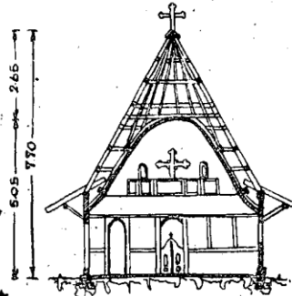
ПОПРЕЧНИ ПРЕСЕК
