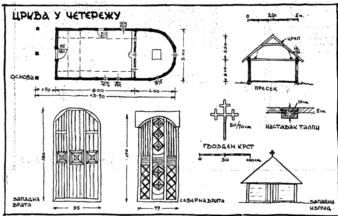
149. Eglise de «Cetereže»: Plan; Coupe; Porte d'entrée; Croix en fer forgé; Jointure de madriers; Façade.
