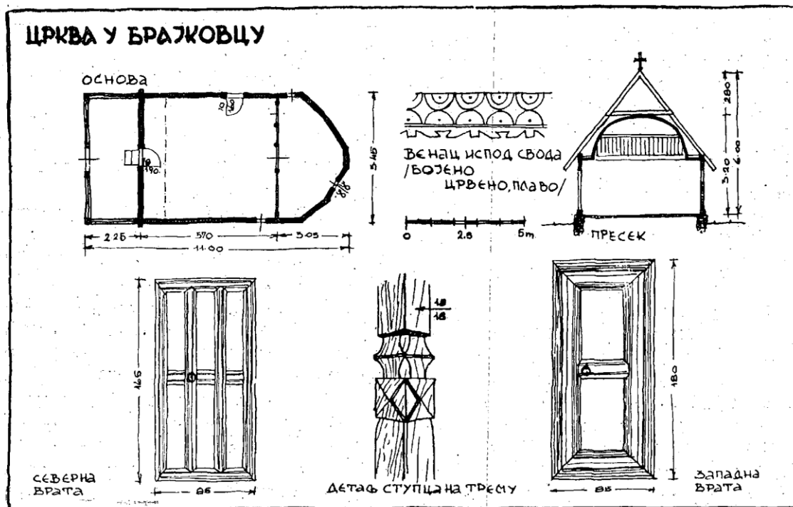
100. Eglise de «Brajkovac»: Plan; Coupe; Portes d'entrée; détails d'ornements.
