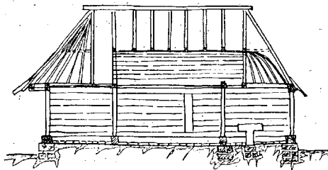
ПОДУЖНИ ПРЕСЕК
