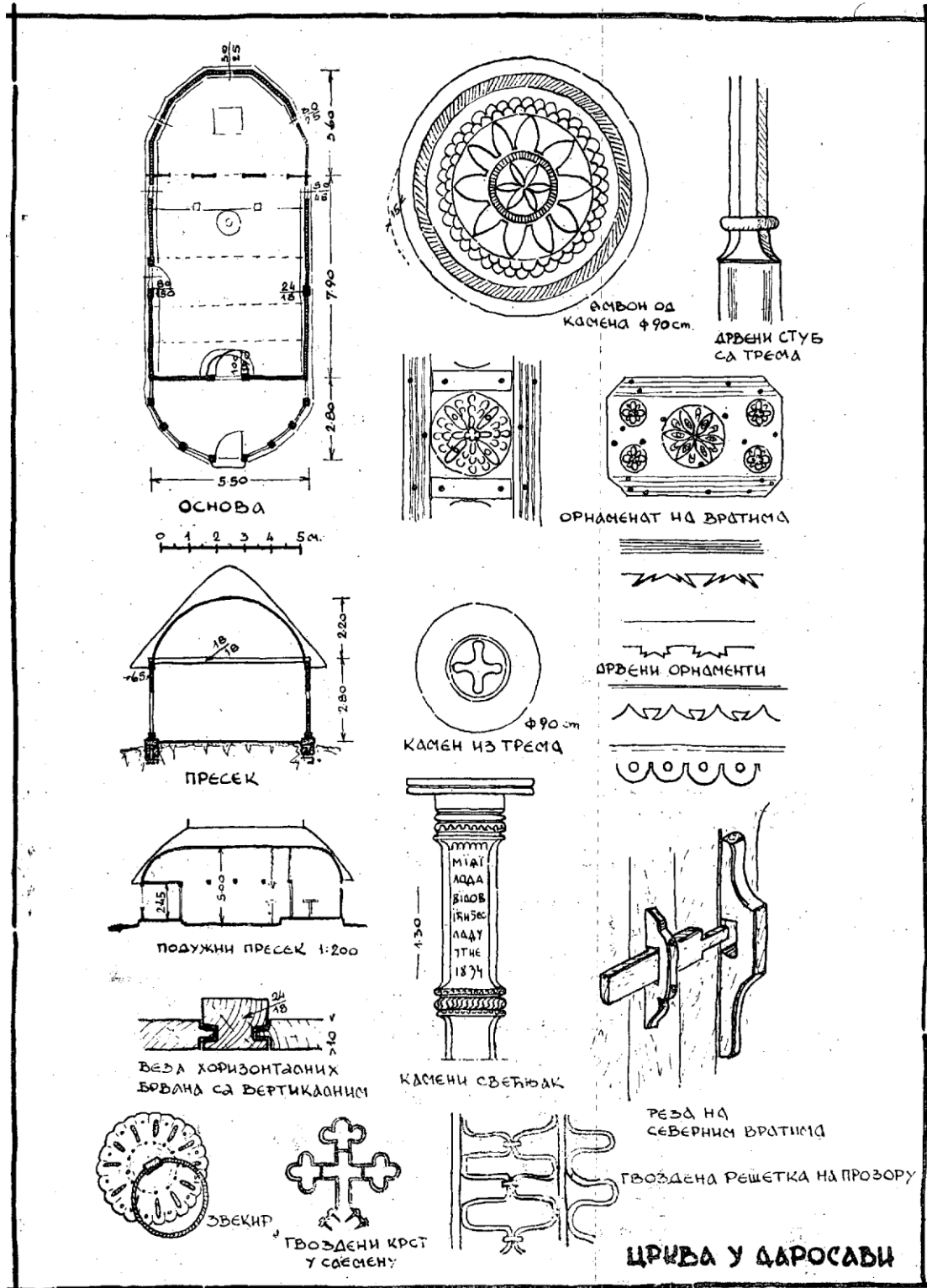
112. Eglise de «Darosava»: Plan; Coupes; Ambons et chandelier de pierre; Pilier en bois du portique; Ornementation en bois; Chevillette; Fer forgé.
