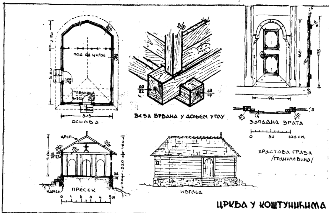
118. église de »Koštunići«: Plan; e; Jointure d'angle; Façade; Porte d'entrée.
