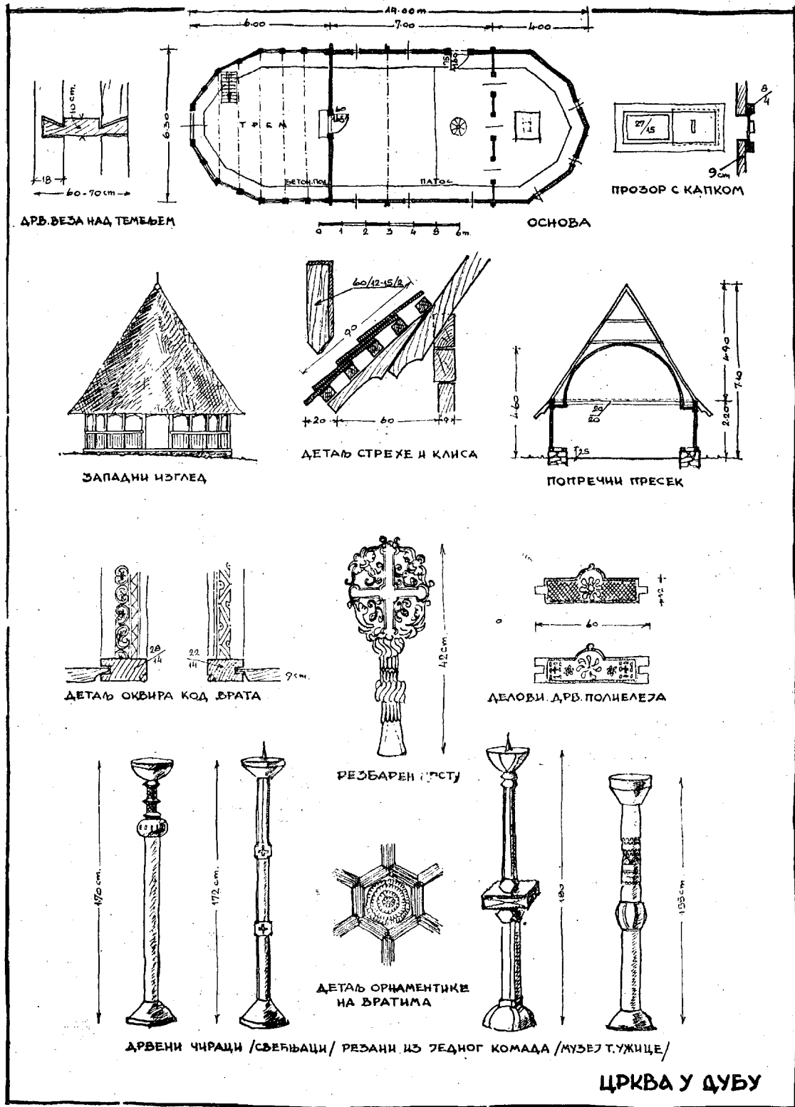
116. Eglise de «Dub»: Plan; Façade; Coupe; Détails: jointure, toiture, fenêtre à coulisse, ornements; Croix et chandeliers de bois.
