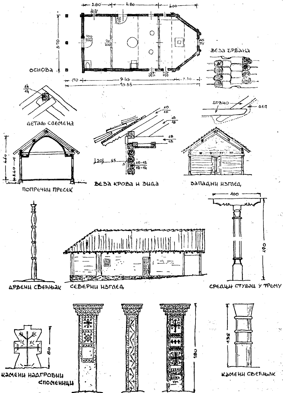
109. Eglise de «Glogovica»: plan; Détails du toit et des murs en madriers; Coupe; Façades; Chandeliers en bois et en pierre; Pilier de bois; Tom beaux de pierre.
