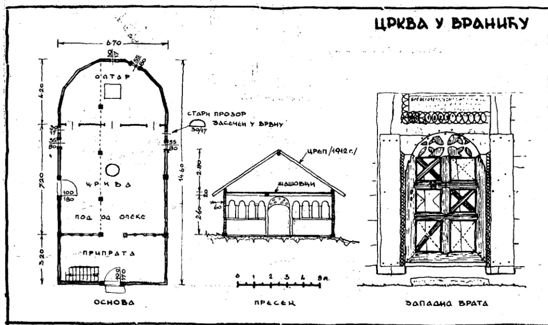
105. Eglise de «Vranić»: Plan; Co; Porte d'entrée.
