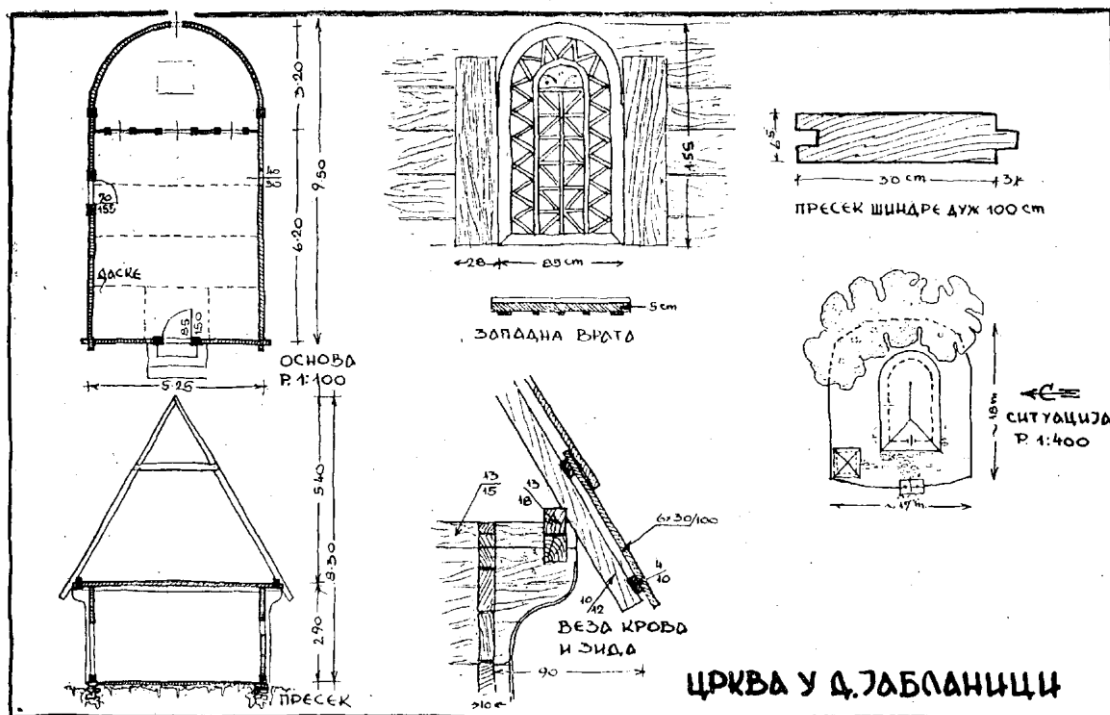
114. Eglise de «Donja Jablanica»: Plan; Coupe; Porte d'entrée; Détails de la charpente; Coupe d'une échandole; Situation.
