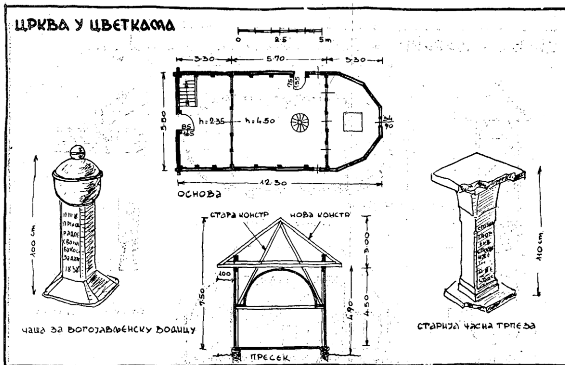
148. Eglise de «Cvetke»: Plan; Coupe; Bé nitier et autel, en pierre.
