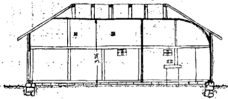
ПОДУЖНИ ПРЕСЕК
