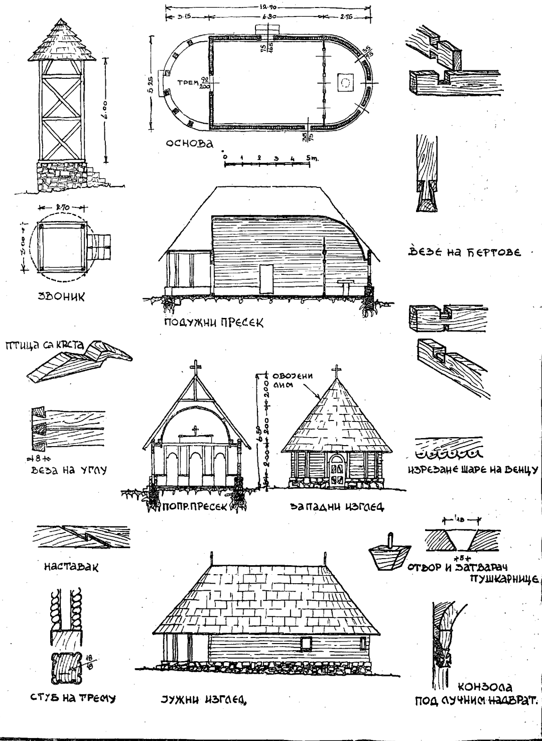
147. Eglise de «Carina»: Clocher: façade, plan; Eglise: plan, coupe, façade, différentes jointures de madriers, ornementation en bois sculpté (D'après les esquisses du Dr arch. D Tadić du Dr M. Corović et R. Ljubinković).
