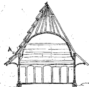
ПОПРЕЧНИ ПРЕСЕК
