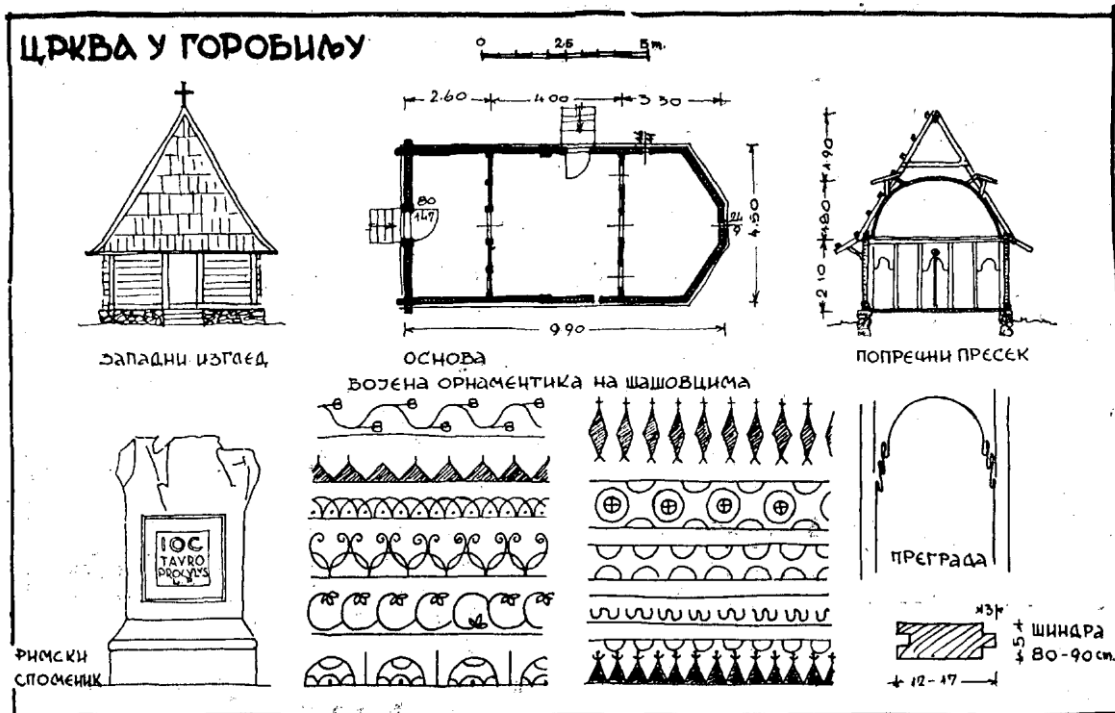
111. Eglise de «Gorobilje»: Façade; Plan; Coupe; Restes d'un monument romain à côté de l'église; Ornaments peints sur la voûte en bardeaux; Cloison; Echandole.
