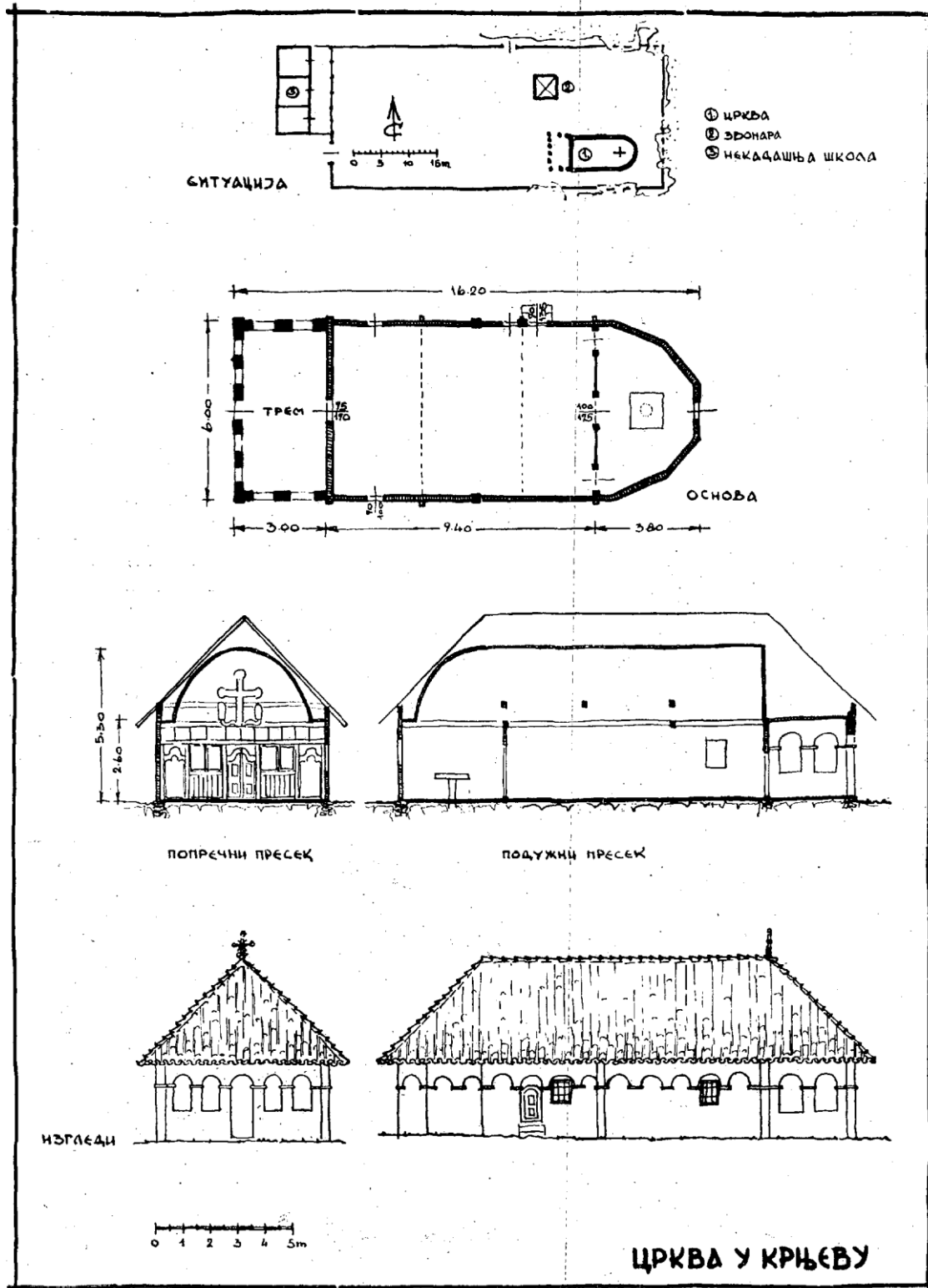
119. Eglise de »Krnjevo«: Situation; Plan; Coupes; Façades.
