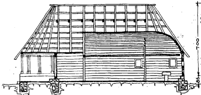
ПОДУЖИ ПРЕСЕК
