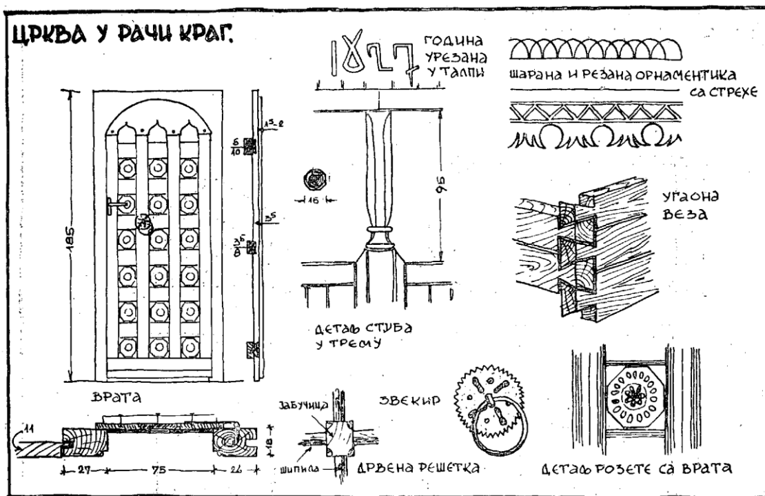
137. Eglise de »Rača Kragujevačka«: Porte d'entrée; Inscription (1827); Dentelure colorée du portique; Pilier du portique; Jointure d'angle; Détails: jointure des barreaux, décorations de porte.
