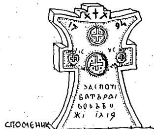
102. Eglise de »Brestovac«: Plan; Façade; Boiseries du plafond; Jointure des poutres murales; Lier de pierre; Pierre tombale; Chapiteau d'un pilier en bois (D'après les esquisses de: M. Jovanović, B. Živković, M. Ladević, S. Mandić).
