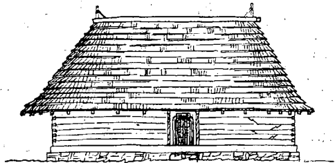
ЈУЖНИ ИЗГЛЕД
