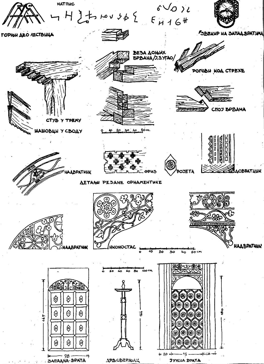
125. Eglise de «Miličinica»: Inscriptions; Détails de jointures et d'ornementations; Porte d'entrée; Chandelier en bois (D'après les esquisses du Dr arch. D.Tadić, du Dr M. Čorović et R. Ljubinković).
