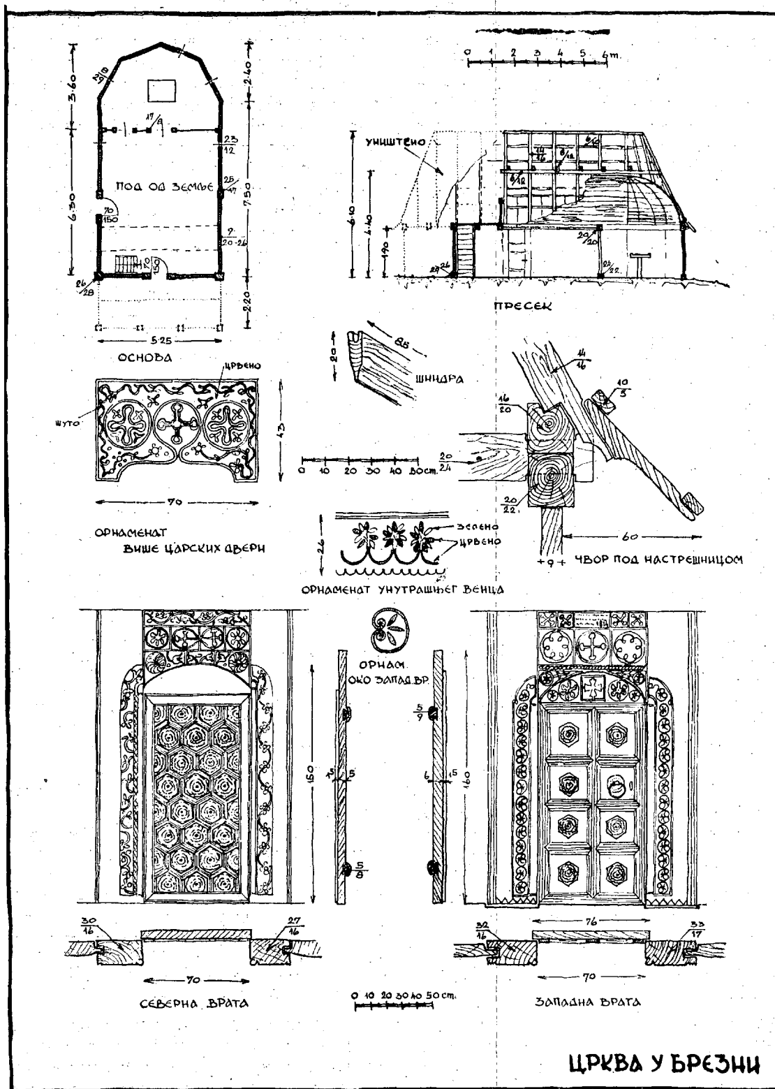
101. Eglise de »Brezna«: Plan; Coupe: Ornaments ; Jointures de poutres sous l'avent; Portes d'entrée.
