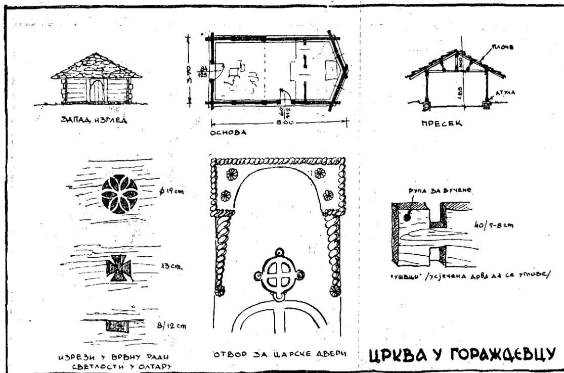
110. Eglise de »Gorazdevac«: Façade; Plan; Coupe; Rosace entaillée dans le bois, et autres ouvertures ménagées dans les madriers en guise de fenêtres; Ornementation surplombant la porté
