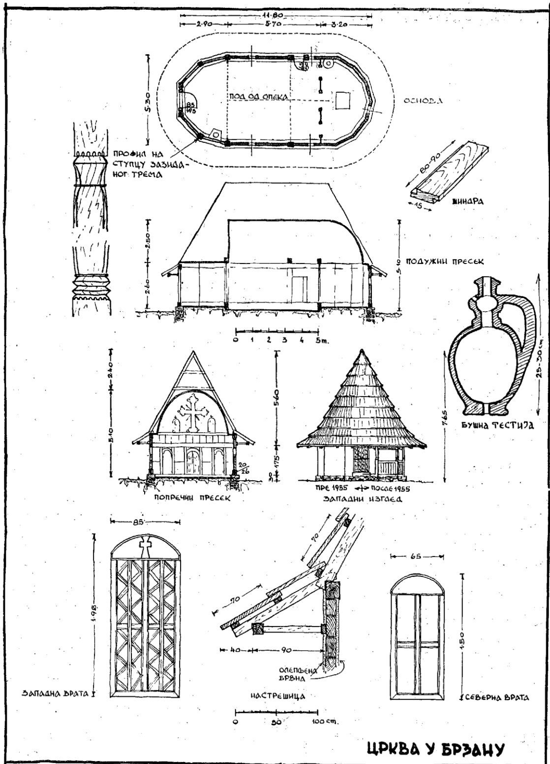
103. Eglise de »Brzan«: Plan; Coupes; Facade; Détails: pilier, échandole; Poterie acoustique; Portes d'entrée; Détail des éléments del'auvent.
