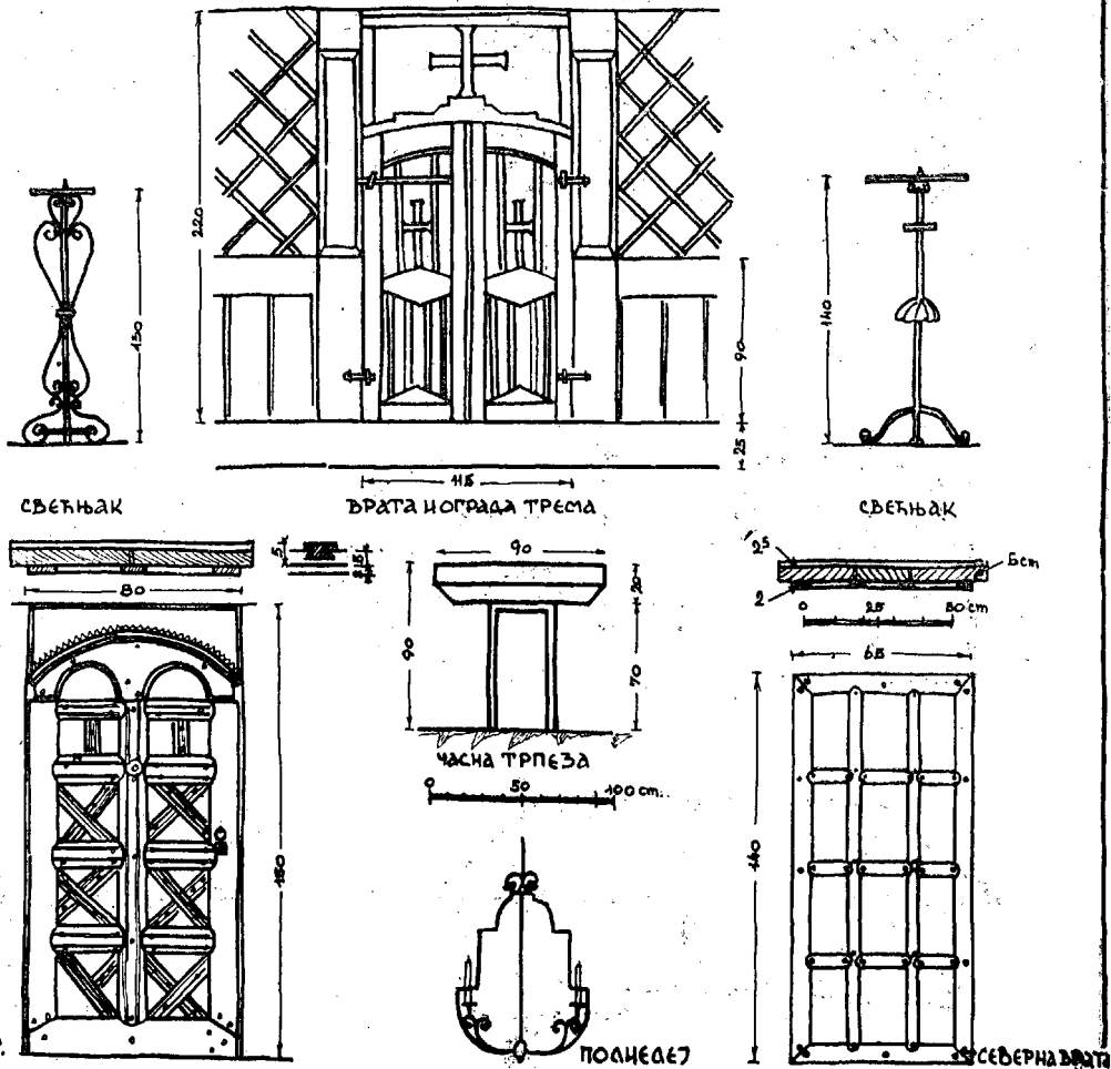
131. »Pokajnica« près »Velika Plana«: Détail de l'iconostase; Croix au faite du toit; Inscriptions (1818); Chandeliers en fer forgé; Détails du portique; Portes d'entrée: principale et latérale; Autel de pierre; Lustre.
