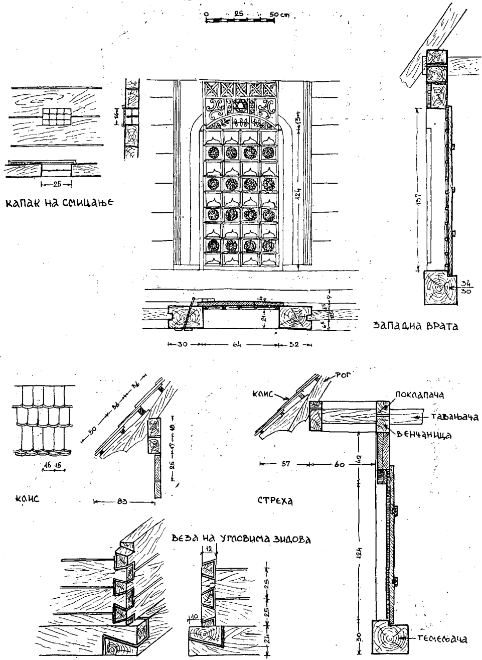
145. Eglise de «Takovo»: Couvercle à coulisse; Porte d'entrée; Toiture en bardeaux; Différentes jointures de madriers (D'après les dessins du prof. B. Kojić).
