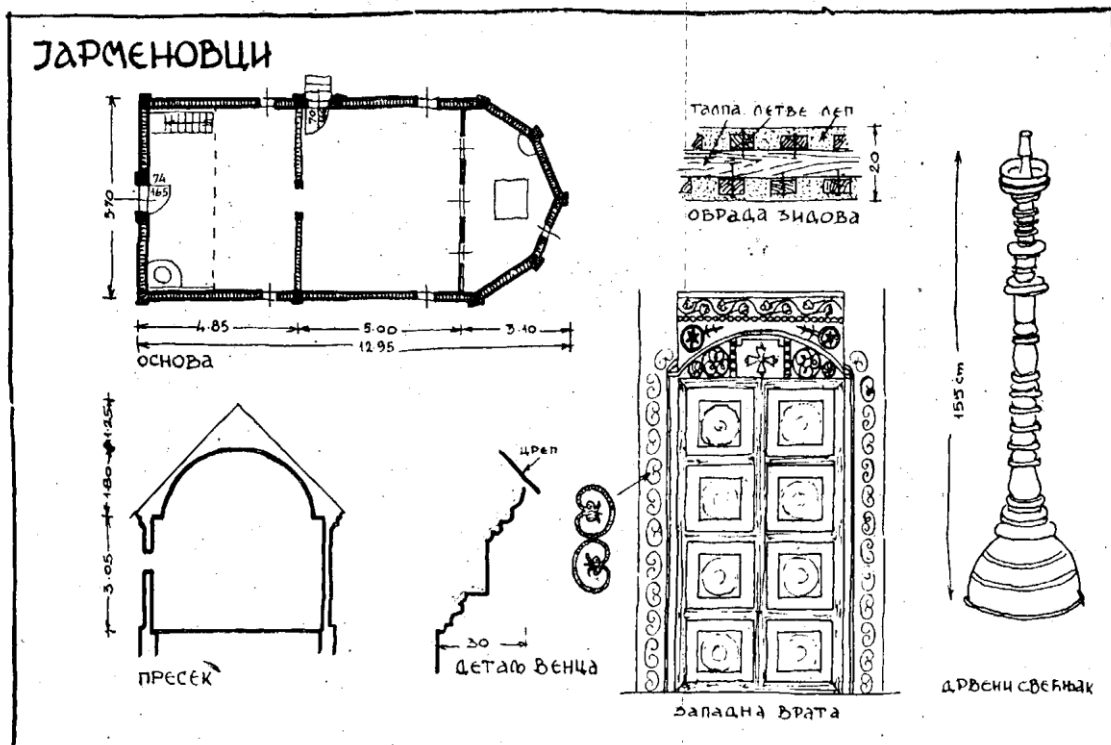
117. Eglise de «Jarmonovci»: Plan: Coupe: Détails du mur: Porte d'entrée: Chandelier en bois.
