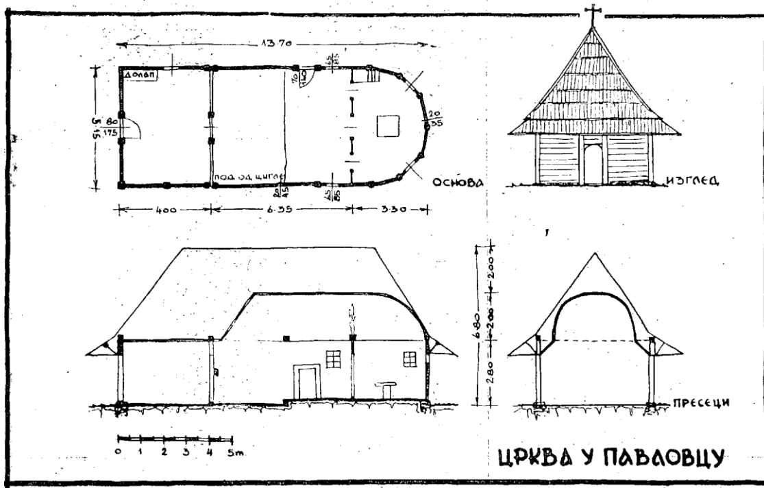
127. Eglise de «Pavlovac»: Plan; Façade; Coupes.
