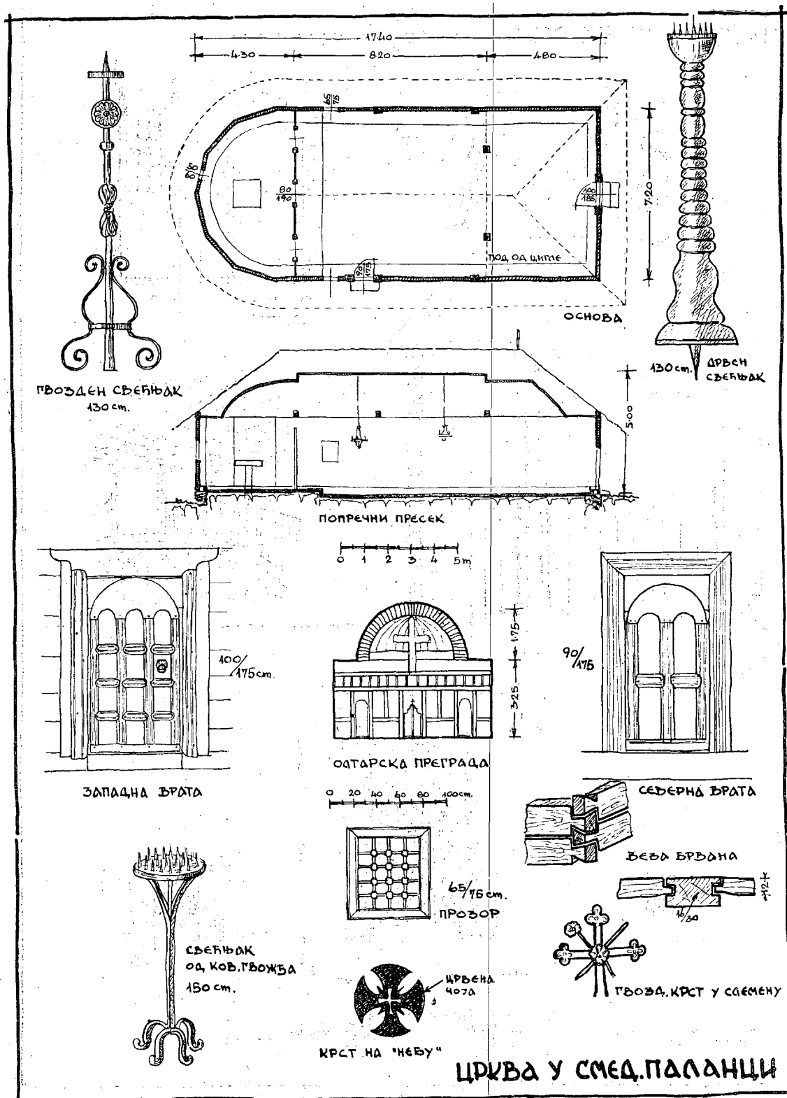
143. Eglise de »Smederevska Palanka«: Plan; Coupe; Chandeliers: en fer forgé, en bois; Fortes d'entrée; Schème de l'iconostase; Fenêtre; Jointures; Croix.
