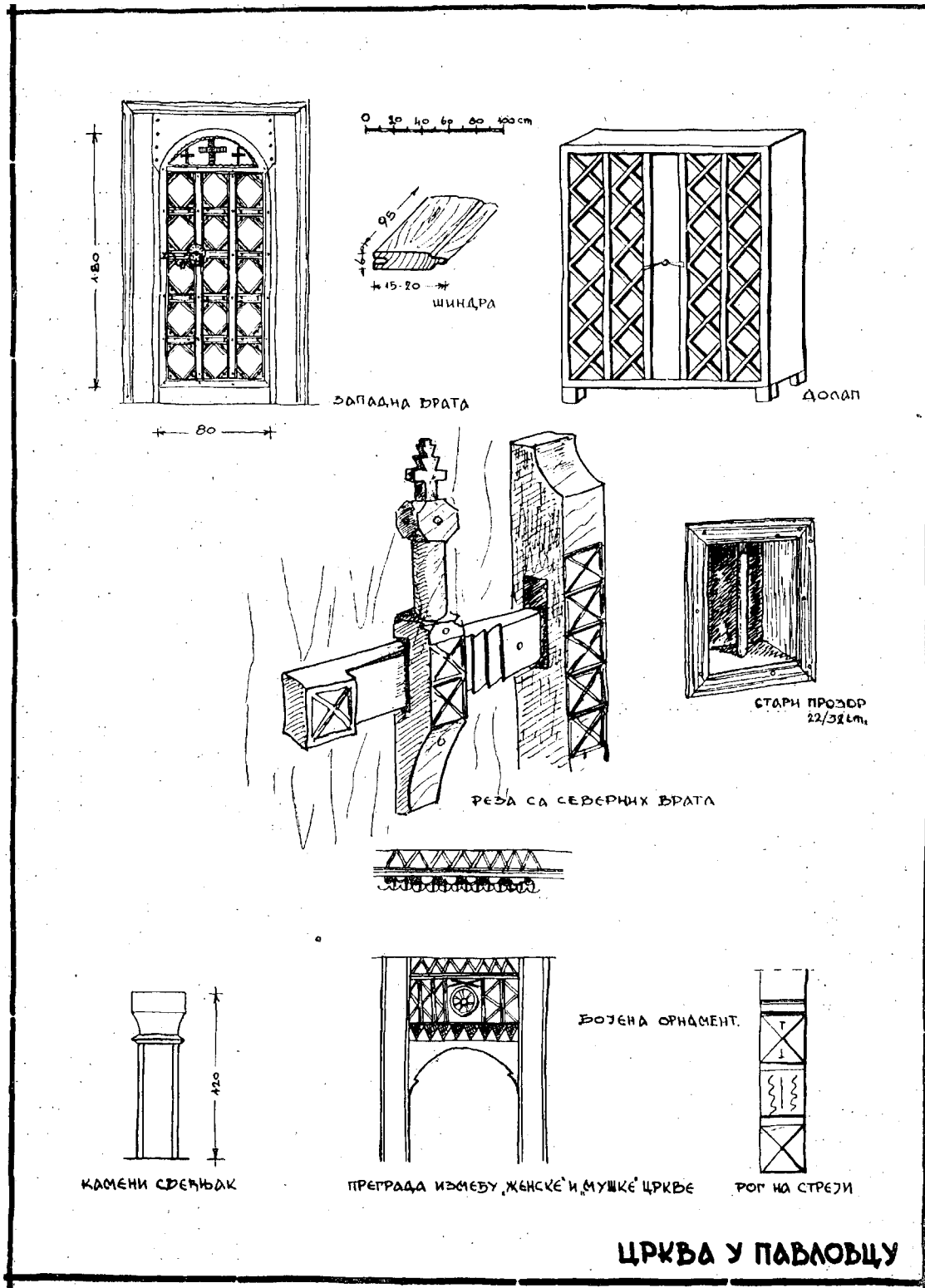
128. Eglise de «Pavlovac»: Porte d'entrée; Echandole; Armoire; Chevillette; Fenêtre; Chandelier de pierre; Décorations.
