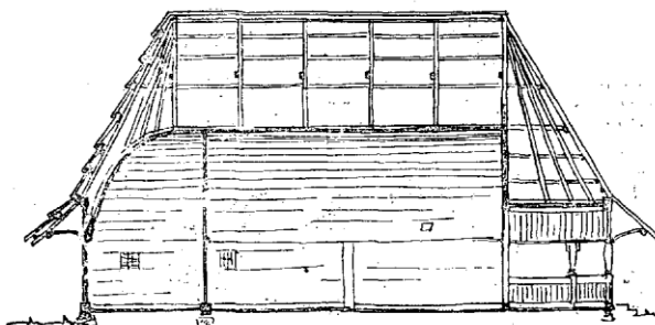
ПОДУЖНИ ПРЕСЕК
