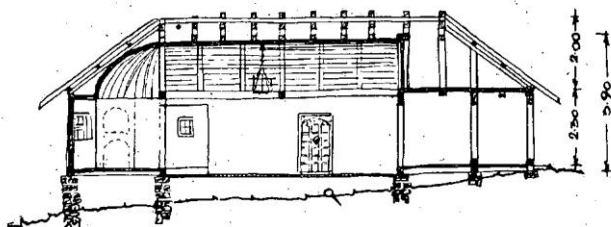
ПОДУЖНИ ПРЕСЕК
