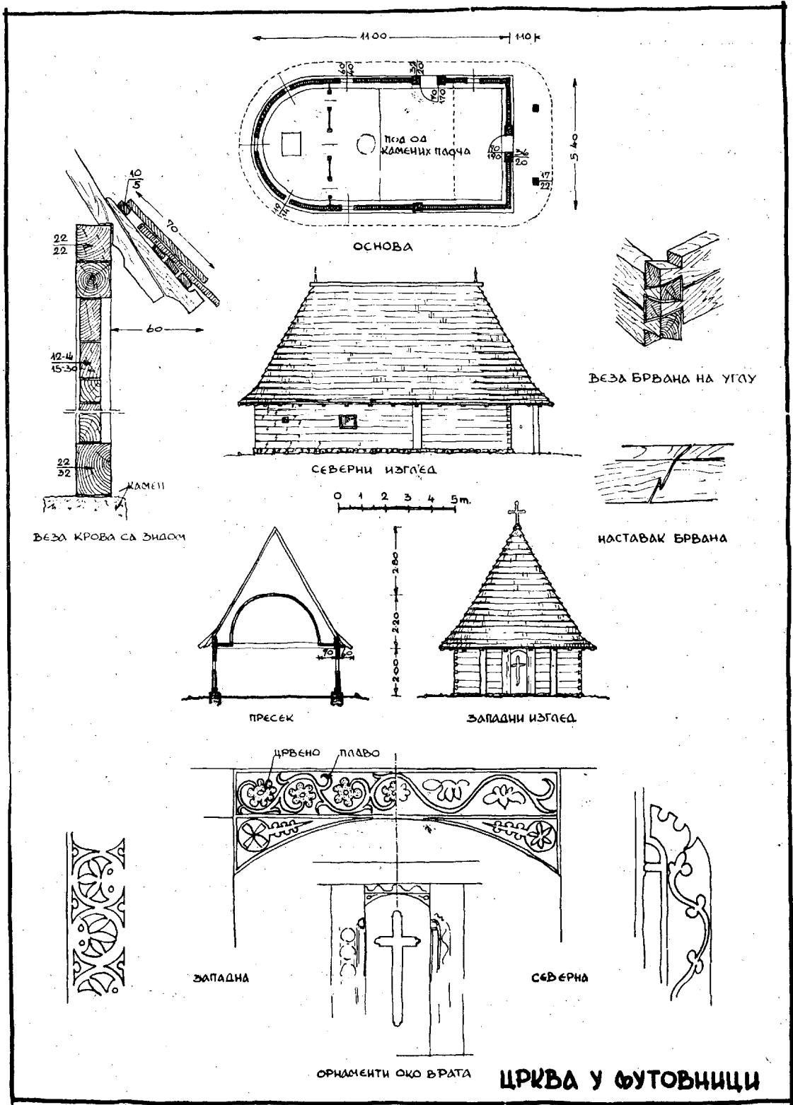
123. Eglise de «Ljutovnica»: Plan; Façades; Cou pe; Détails de la charpente; Décoration de la porte d'entrée.
