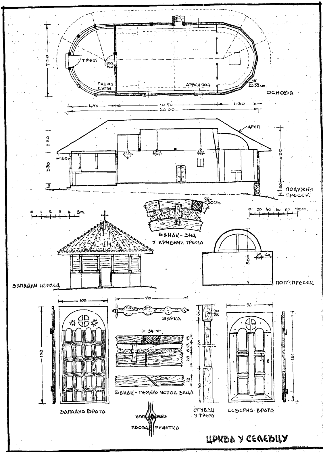
139. Eglise de «Selevac»: Plan; Coupes; Fa çade; Détails de soubassements dans la charpente; Portes d'entrée; Fer forgé; Pilier en bois.
