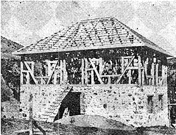
14. Пријепоље, конструкција и структура зграде најновијег порекла.
