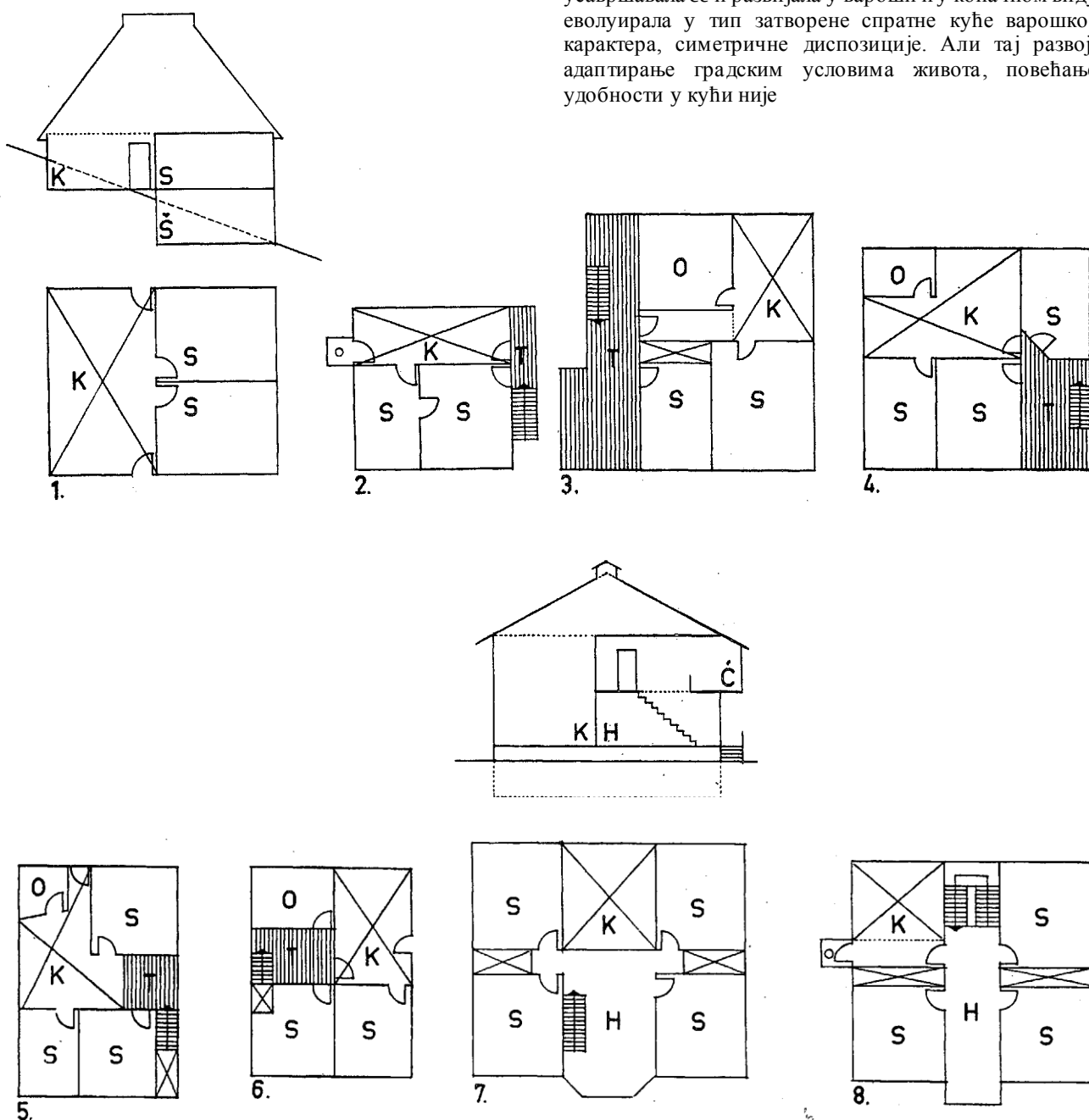
7. Пријепоље, претпостављена линија развоја схеме плана куће у вароши
