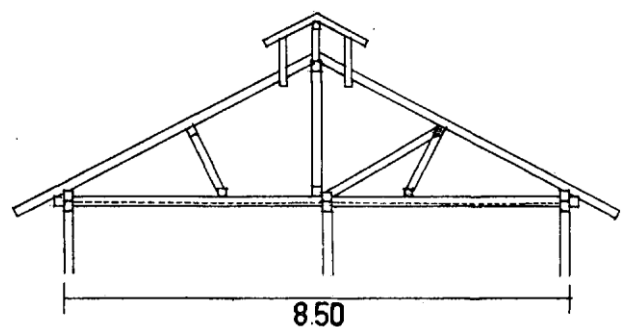
13. Пријеполје, кровна конструкција ћерамидног покривача старијих типова зграда у вароши
