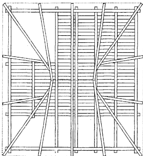
12. Пријеполје, конструкција крова и структура кровног покривача и саме зграде типа мале куће из Вакуфа
