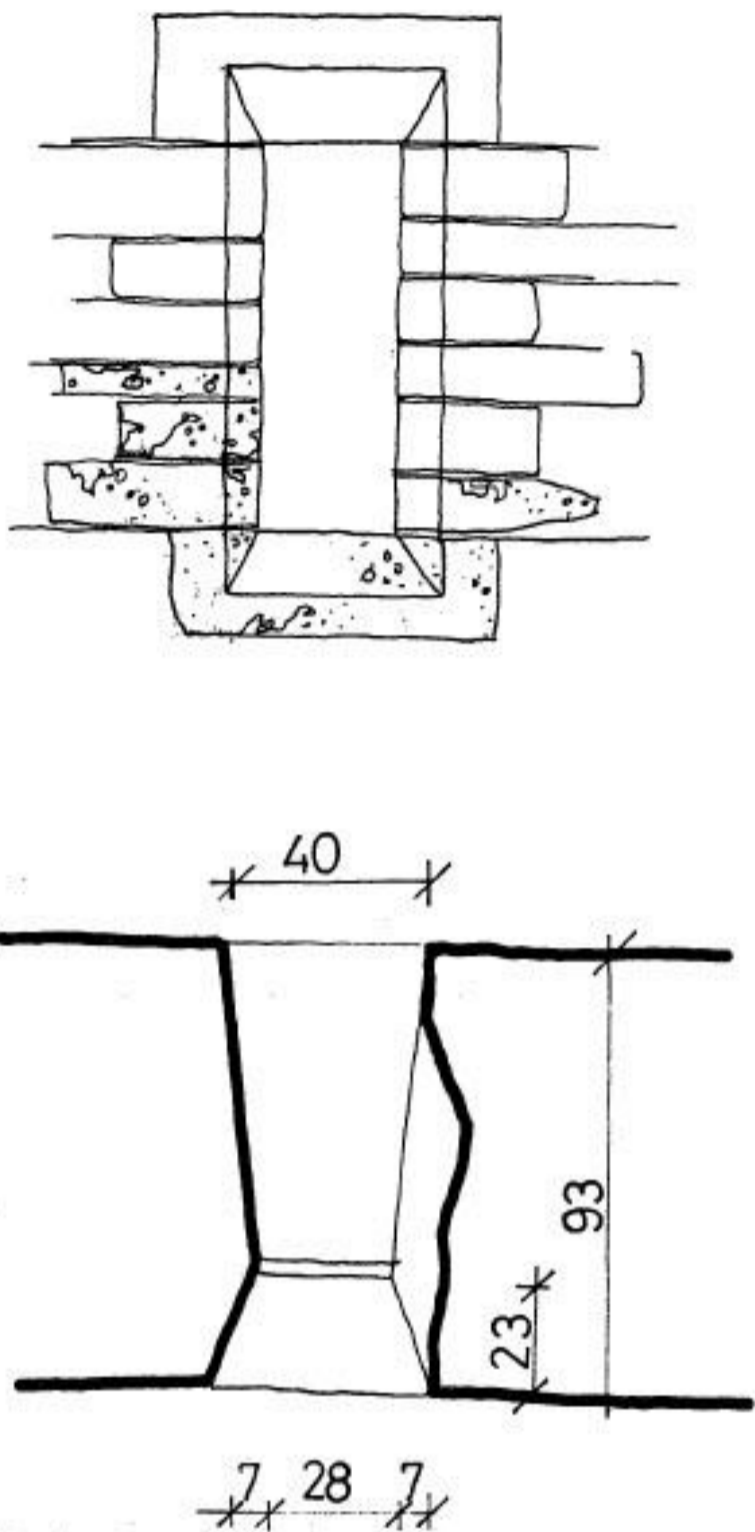
8. Прозор на јужном зиду источног травеја олтарског простора, идеална реконструкција.
