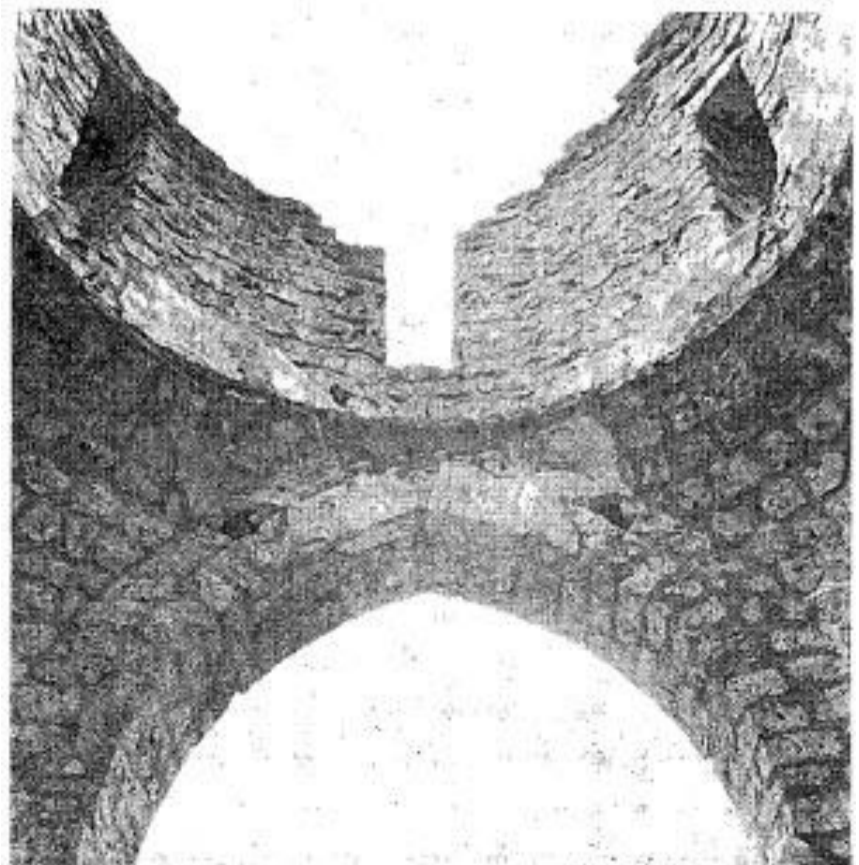
Fig. 10. Traitement et rangement des vousses dans l'espace central de l'église.
