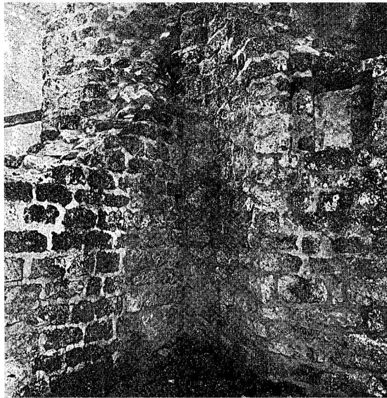
5. Спојница између средишног простора и апсиде северног параклиса.
