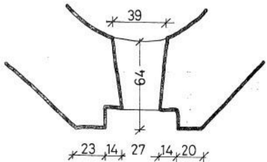
9. Прозор на апсиди северног параклиса, идеална реконструкција.
