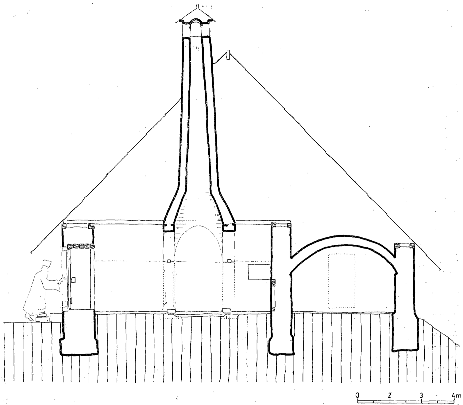
Сл. 19. Попречни пресек кроз кухињу (идеална реконструкција).
