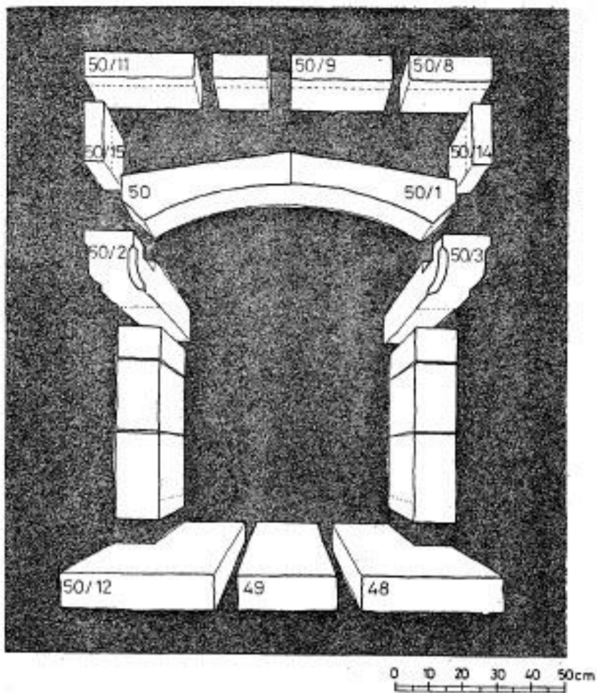
Сл. 12. а) Схема камина у расклопу — Трpezарија XV век.
