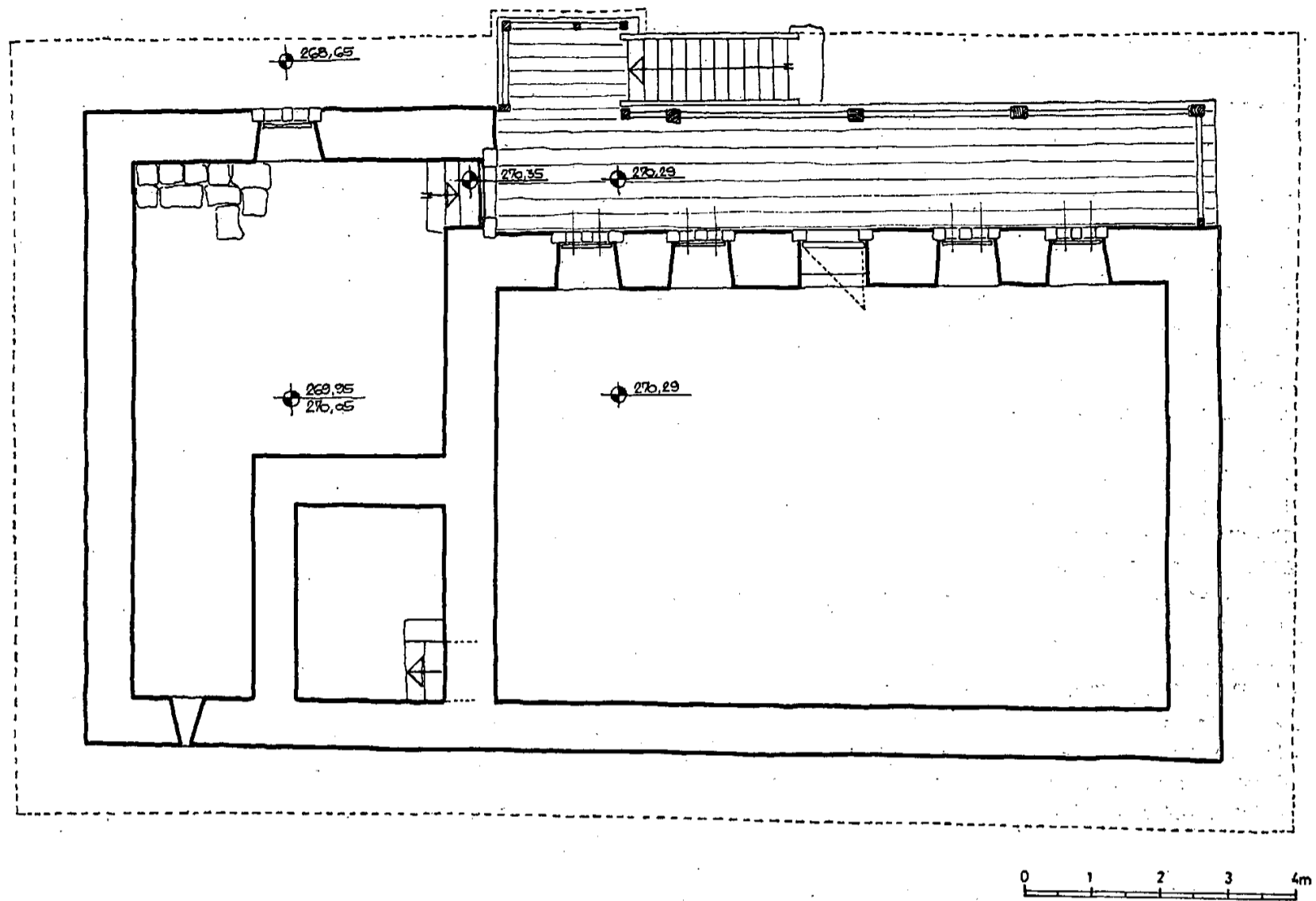
Сл. 6 Основа спрата стамбене грађевине (I) из XV века.
