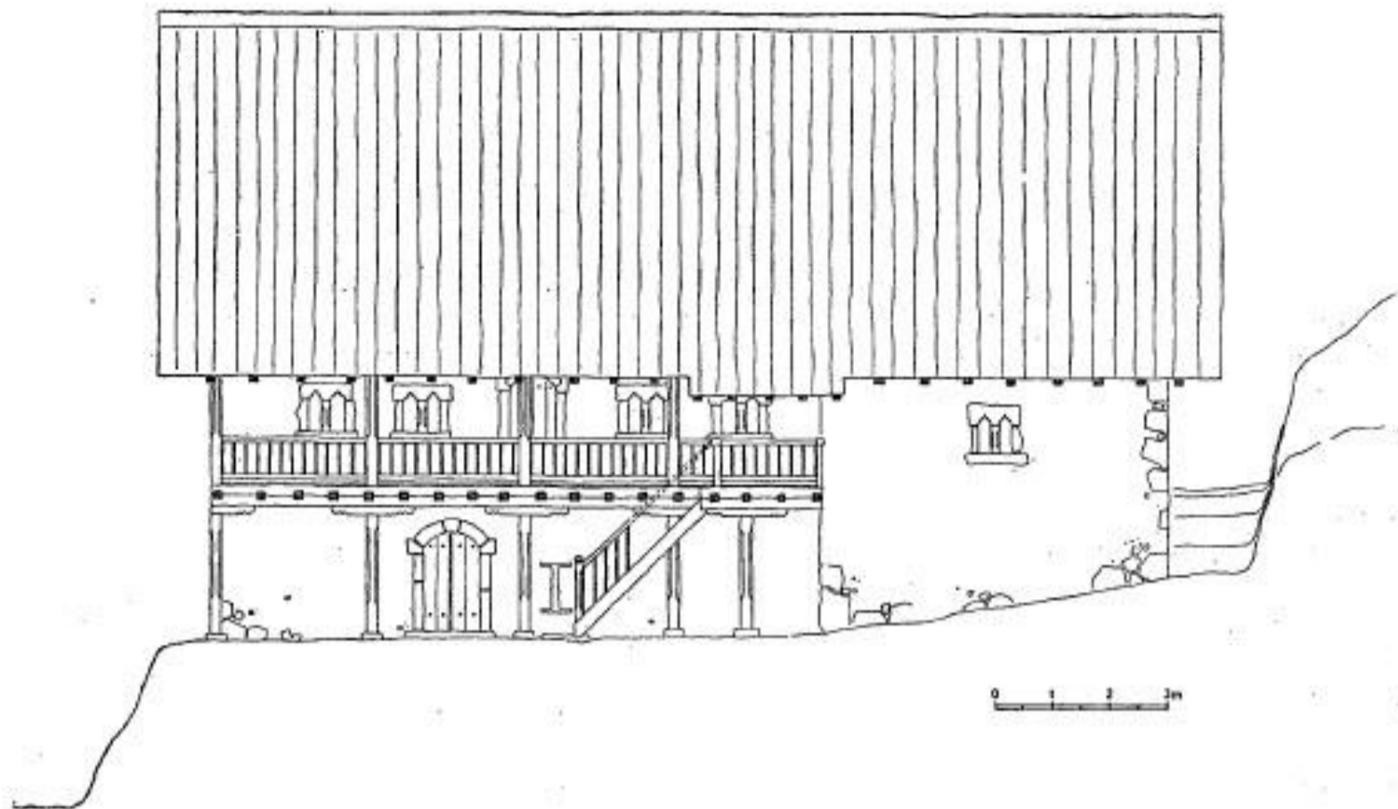
Fig. 10. Maison d'habitation du XV e siècle, — aspect sud, (reconstruction idéale).
