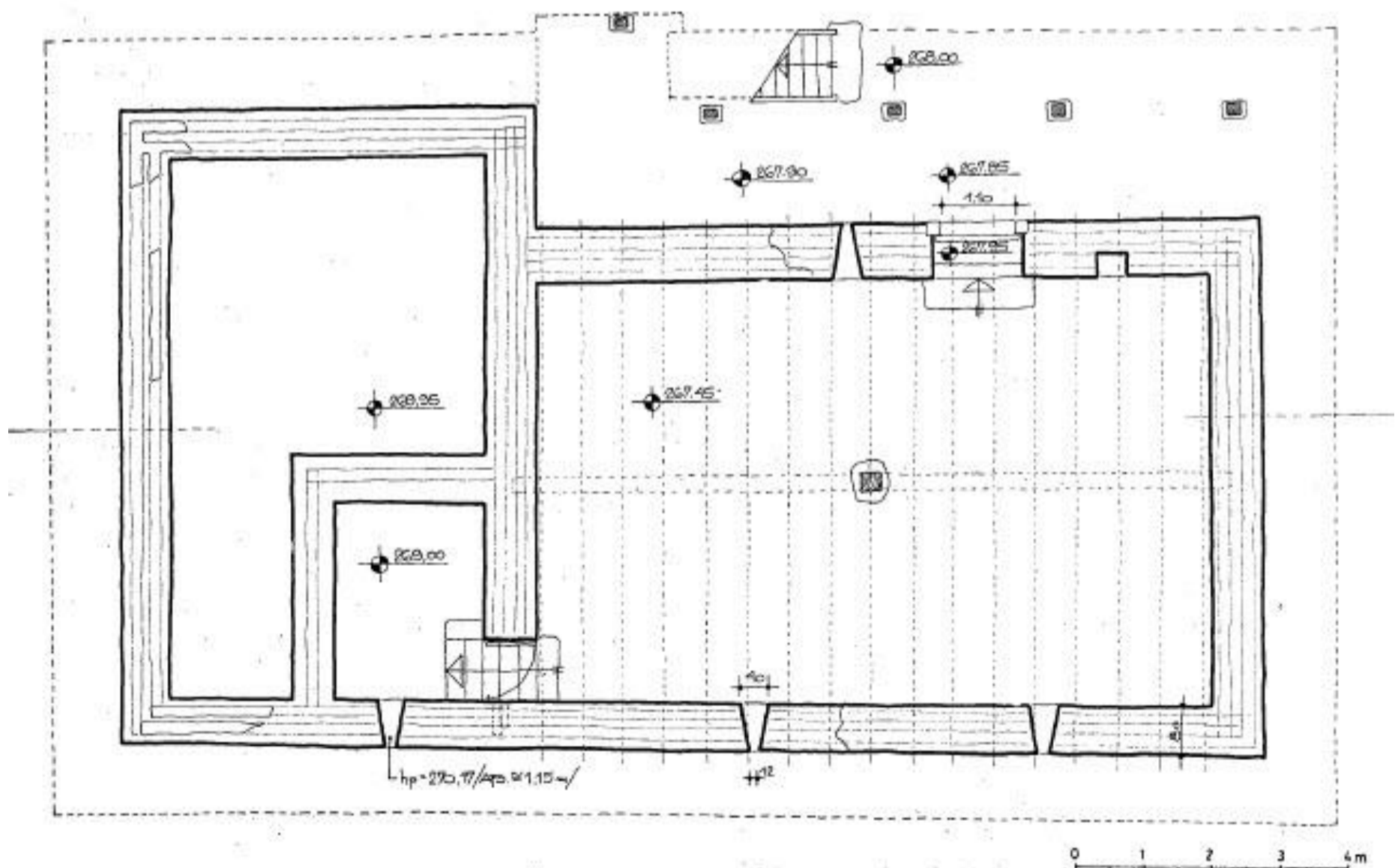
Fig. 5. Plan du rez-dechaussée de la maison d'habitation (I) du XV e siècle.
