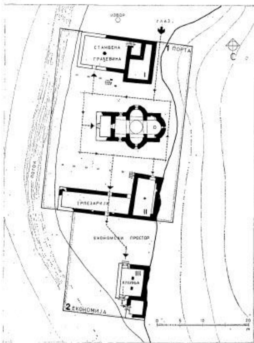
Сл. 2. Манастир у Павловцима — просторна анализа комплекса са схемом кретања.
