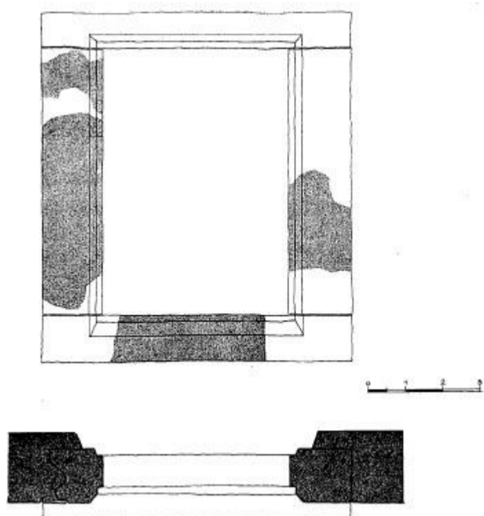
Сл. 15. Прозор Трпезарије XV век. Fig. 15. Fenêtre du réfectoire du XV e siècle.
