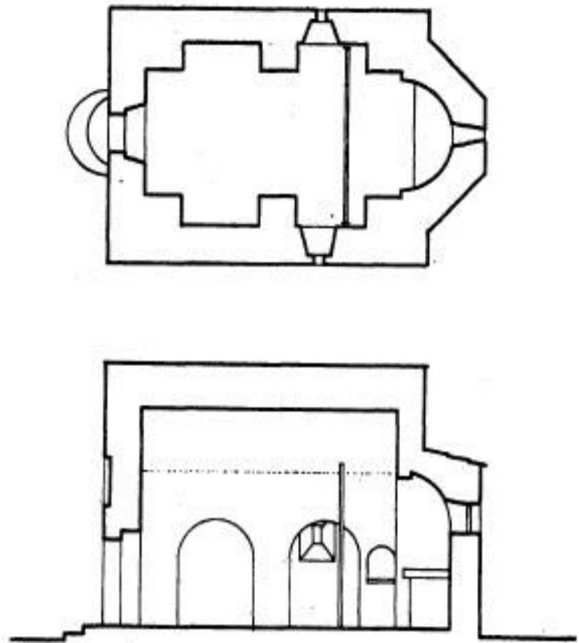
Сл. 3. Гребник, основа и пресек цркве Св. Јеремије (по теренском снимку арх. Р. Финдрика, 1956. године)
