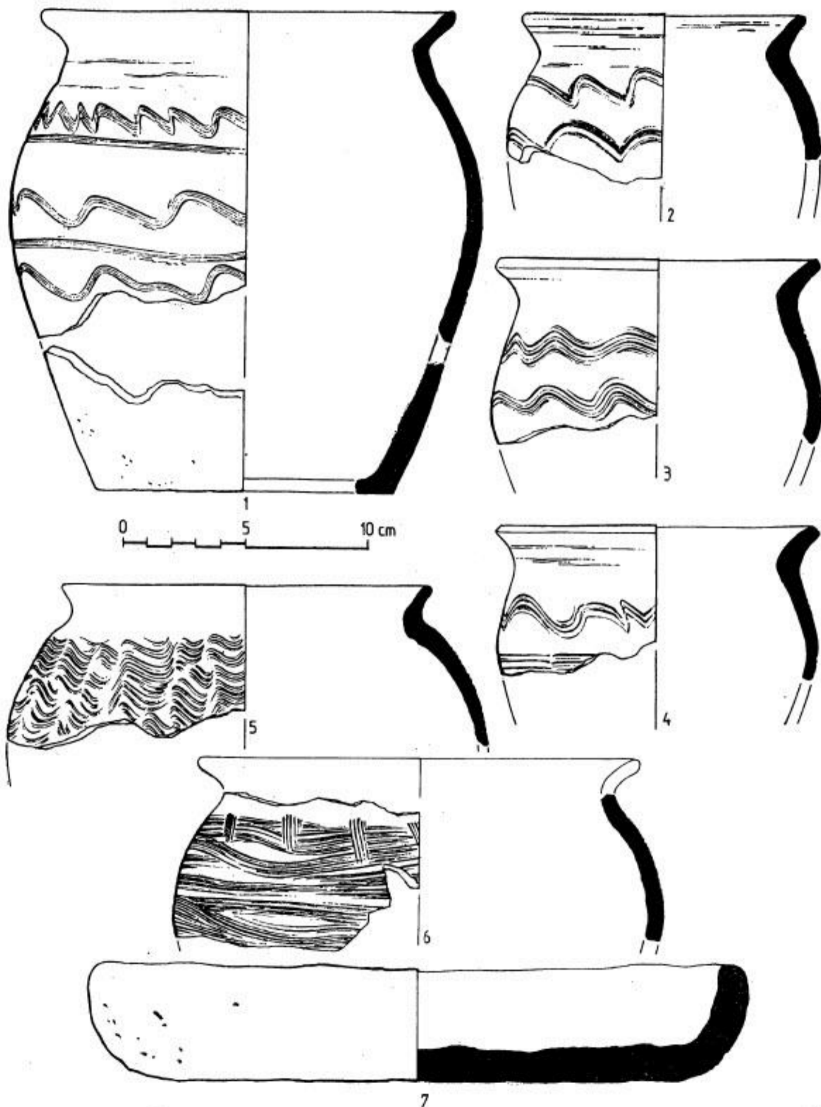
Сл. 7. Рас — Подграђе, керамика из средњовековног хоризонта — прва група (цртао Н. Степановић)
