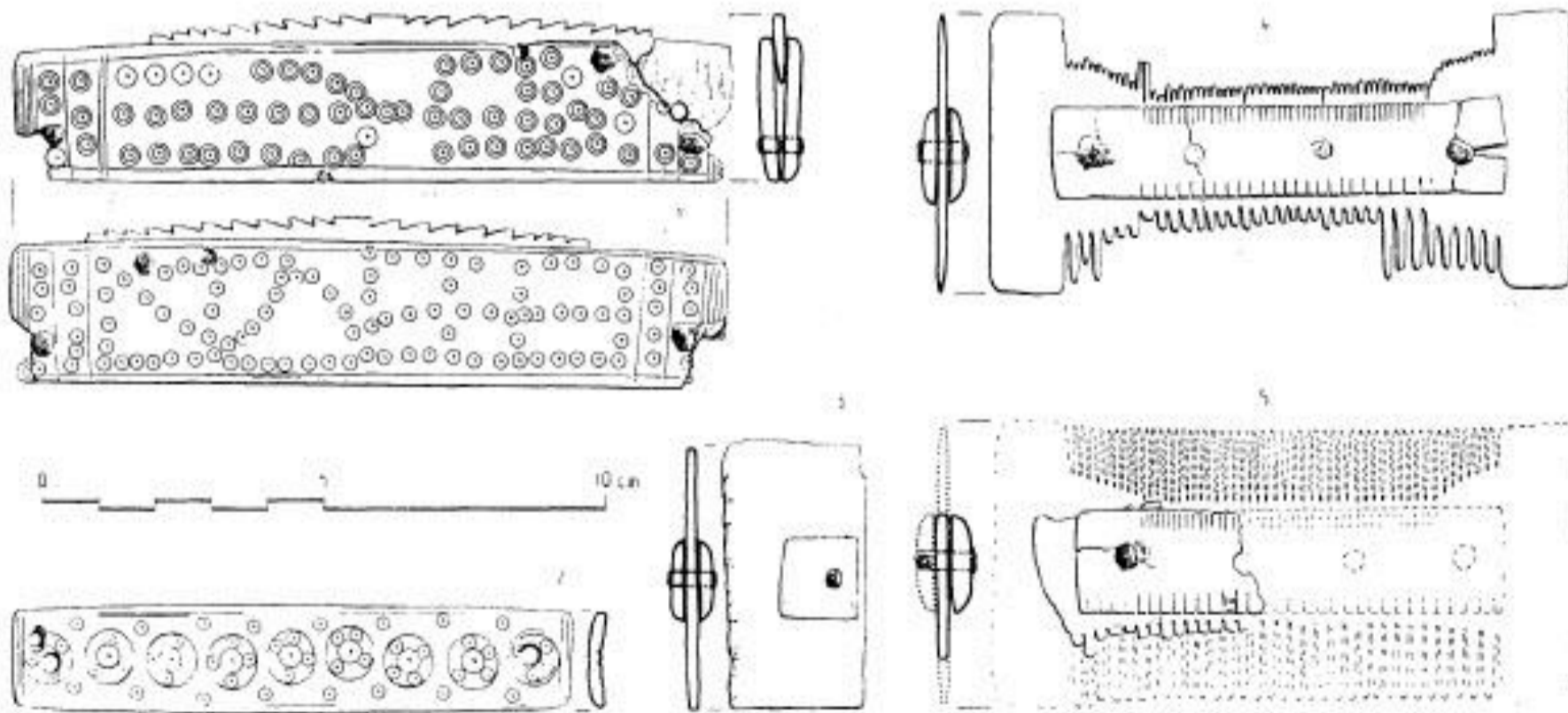
Сл. 6. Рас — Подграђе, коштани предмети из касноантичког хоризонта (цртао Н. Степановић)
