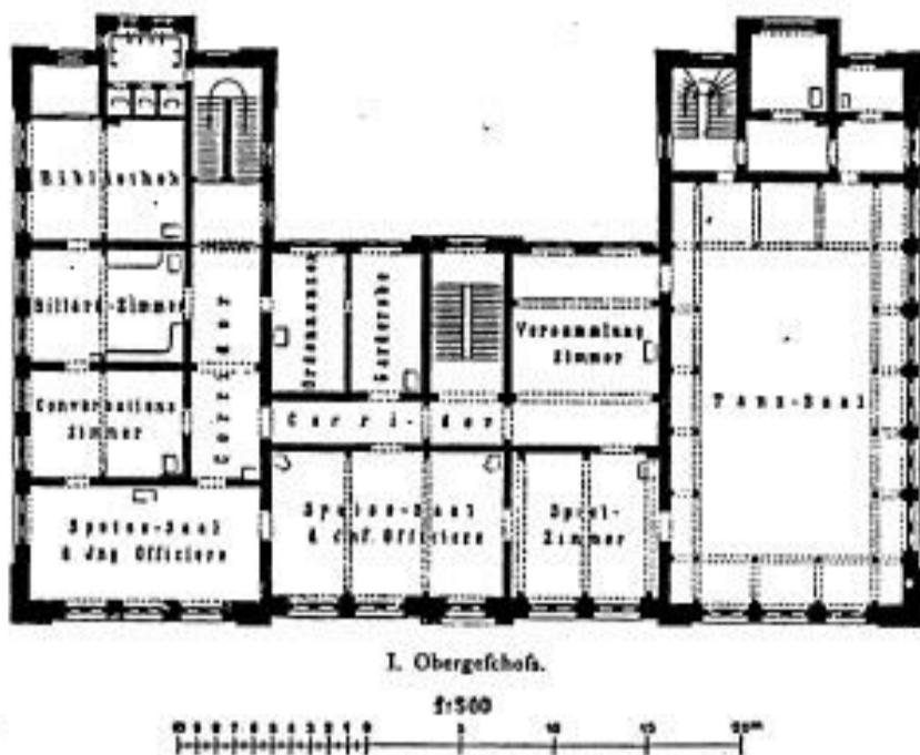
Сл. 10. Основа јавне грађевине са два крила у Шћећину (Пољска) из краја 19. века, Handbuch der Architektur, Viertes Teil, fig. 66, Stuttgart 1904. Fig. 10. Plan d'un bâtiment public à deux ailes de Szczecin (Pologne), XIX e siècle, Handbuch der Architektur, Viertes Teil, fig. 66, Stuttgart 1904
