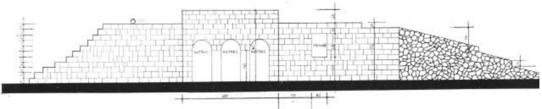
Fig. 4. Orašac, Maričevića Jaruga (Ravin de Maričević), élévation du monument érigé à la mémoire de la Première insurrection serbe (dessin de Mirjane Trebinjac, architecte, 1981, échelle: 1:50).
