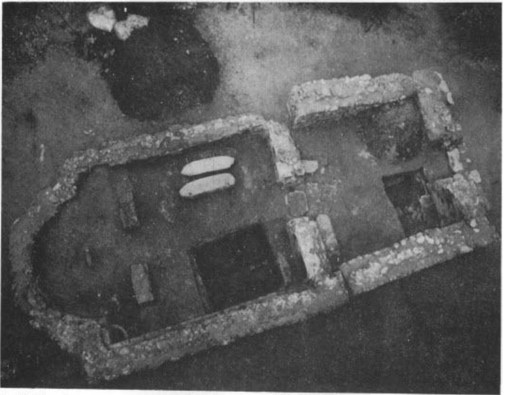
Fig. 10. Eglise et narthex avec les tombes ouvertes n° 1 à 4, après l'achèvement des travaux de fouille. Vue prise d'en haut.
