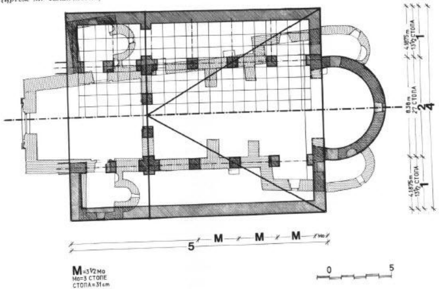
Сл. 12. Претпостављена основа старијег светилишта са анализом пропорцијских односа (цртеж М. Чанак-Медић)
