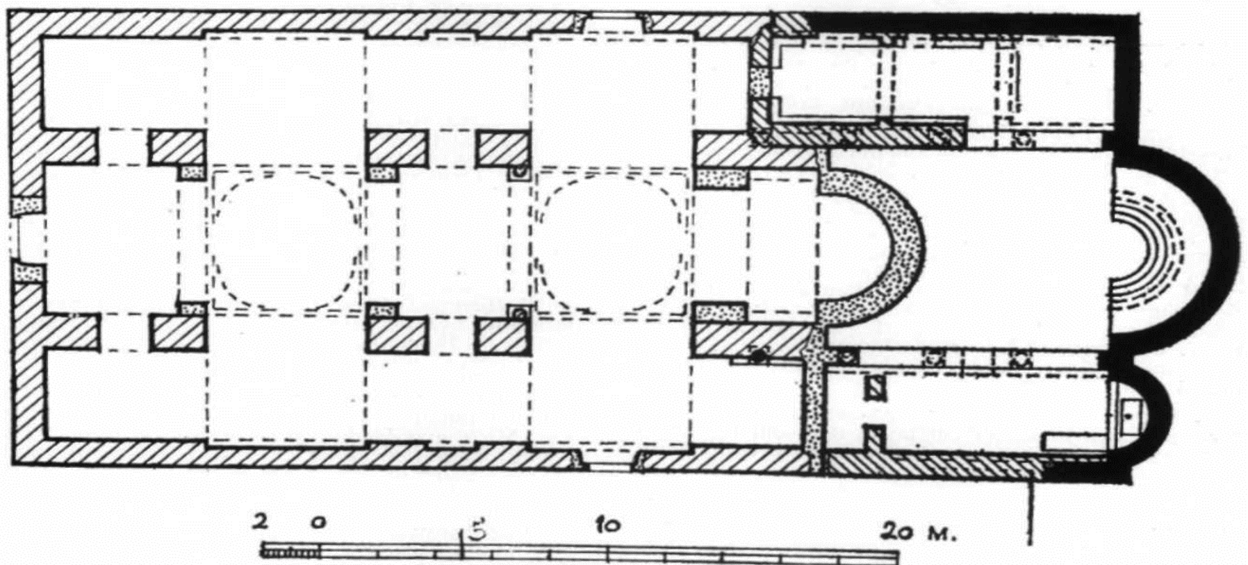
Сл. 2. Основа Светог Варнаве код Саламине на Кипру са остацима олтарског простора из V века, сачуваним изван постојеће цркве — обележено црним (према А. Н. S. Megaw)
