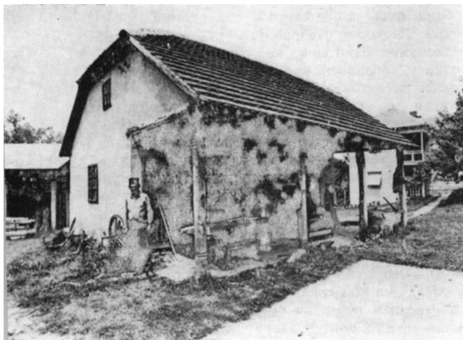
Сл. 20. Ковачница Витомира Вићентијевића, општи изглед са југоистока
