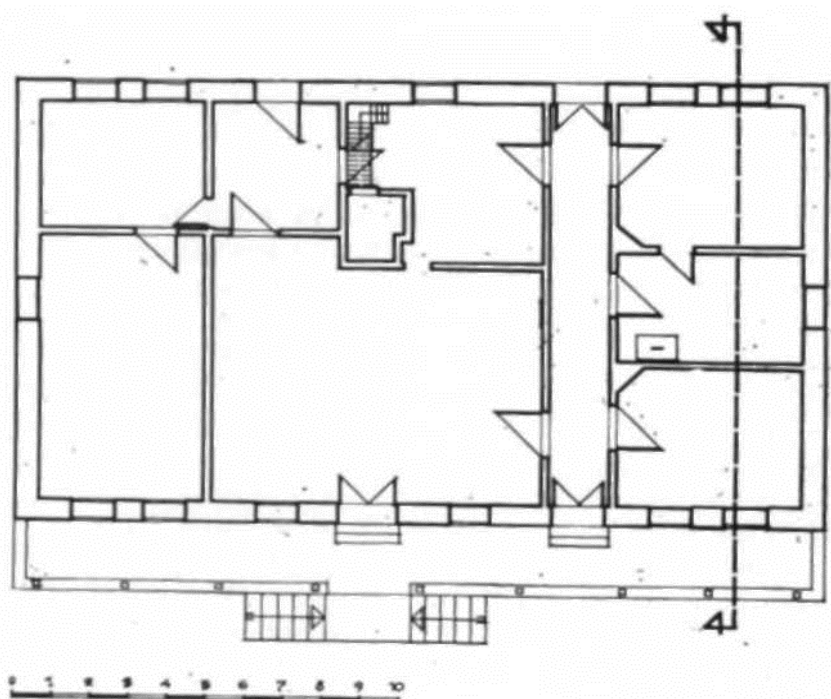
Цртеж 6. Механа Љубинковића, попречни пресек и основа Dessin 6. L'auberge des Ljubinković, coupe perpendiculaire et plan.
