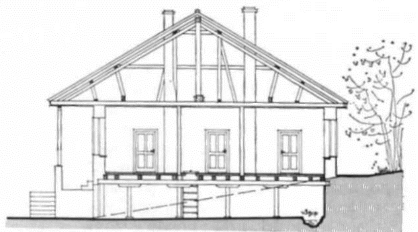
Цртеж 6. Механа Љубинковића, попречни пресек и основа Dessin 6. L'auberge des Ljubinković, coupe perpendiculaire et plan.
