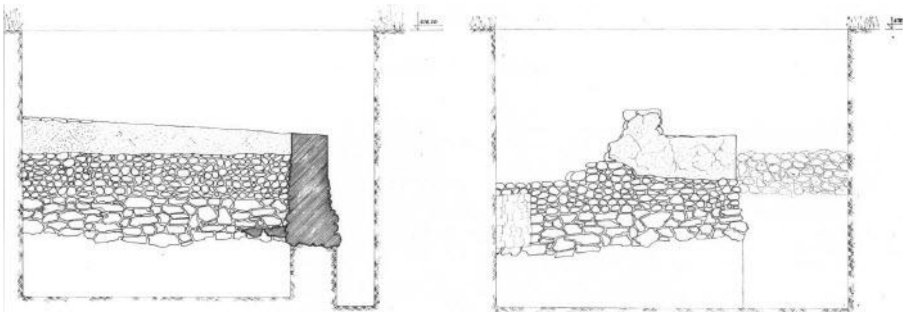
Сл. 8. а и б. Сонда V, зидови и темељи са малтерним везивом Fig. 8. a, б, Sonde V, murs et fondations liés avec du mortier
