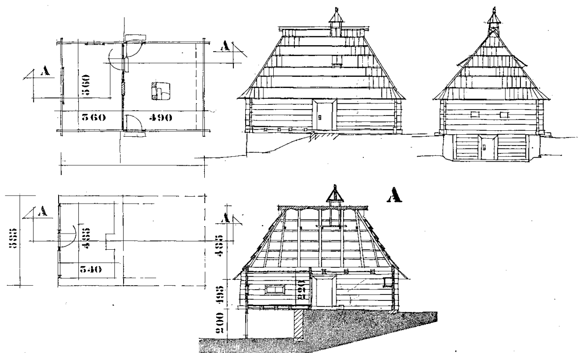
Сл. 4. Старија брвнара са Златибора, село Стубло, основе, изгледи и пресеци
