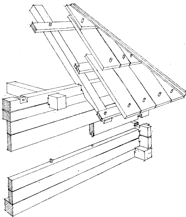
Сл. 13. Конструкција зида и крова брвнаре. Покривач од даичица „шиндре“
