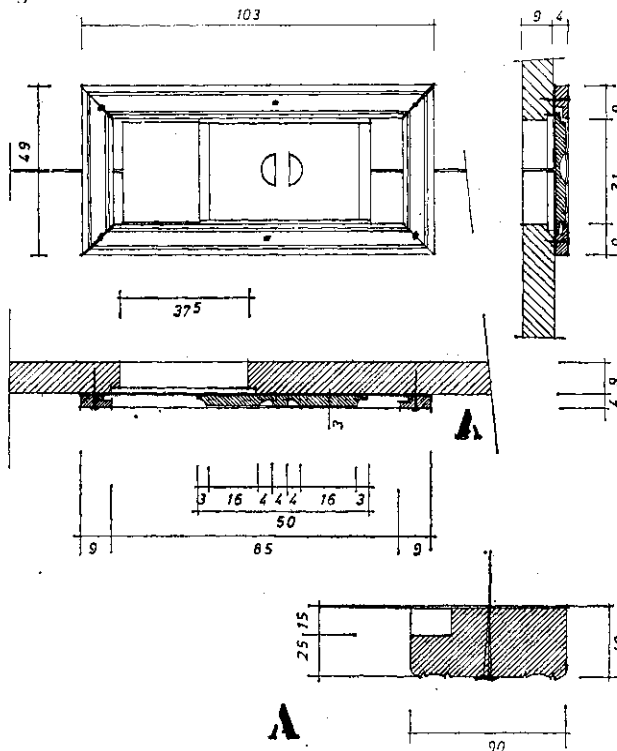
Сл. 14. Прозор на једној брвнари са Златибора. Село Стубло. Мали прозорски отвор затвара дрвени капак који клизи по посебно урађеном жљебу
