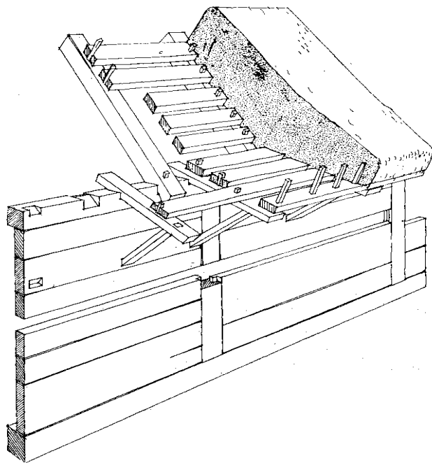
Сл. 12. Кровни покривач од сламе и зидови од талти низани у „диреке“. Рогови и „баскије“ учвршћени су дрвеним клиновима. За стреху се израђује посебна конструкција која држи први ред сламе
