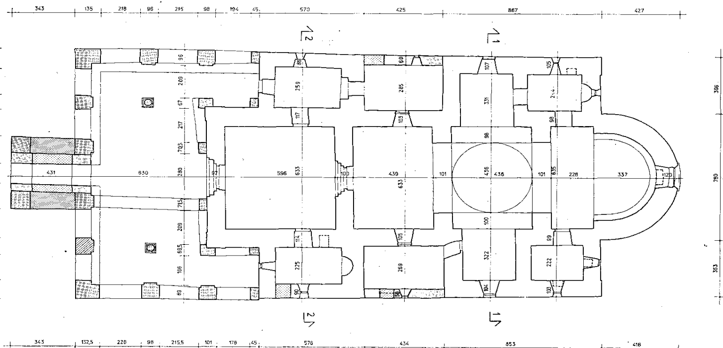
Сл. 6. Основа цркве
