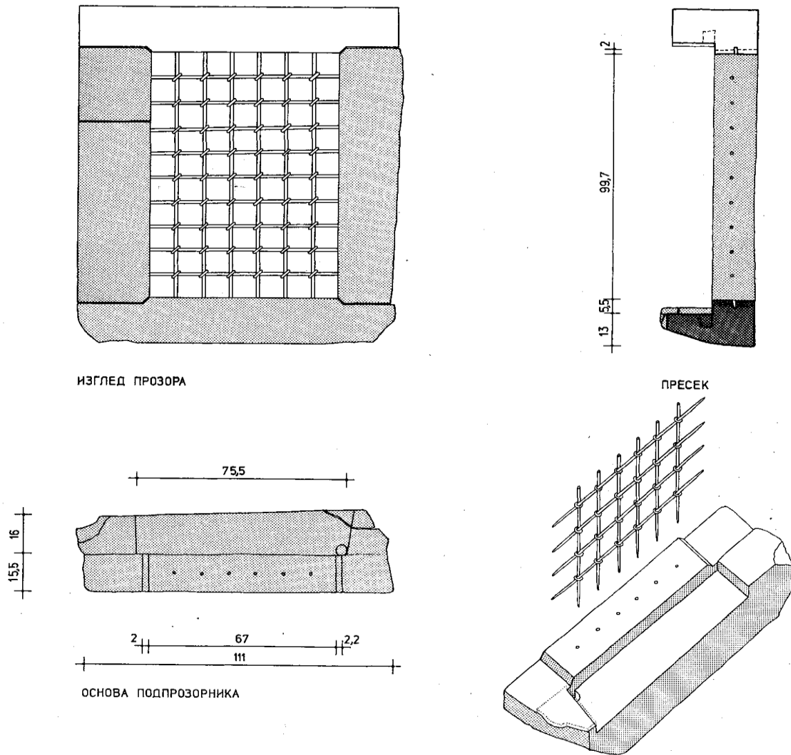
Сл. 19. Реконструкција прозора западне грађевине (II/4). Оригинални делови су затамљени.
