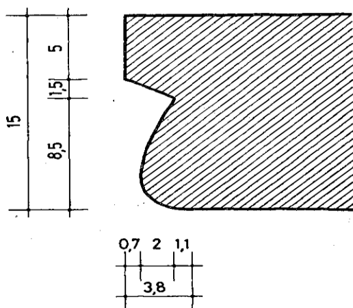
Сл. 9. Профили завршних венаца кубичног постоља (A) и апсиде (B) Fig. 9. Profils des bandes terminales de la base du tambour (A) et de l'abside (B)
