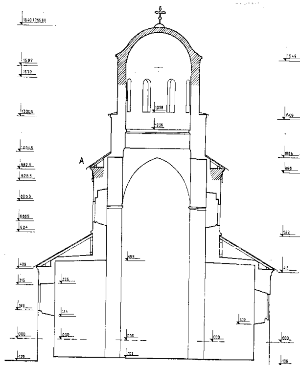
Сл. 7. Попречни пресек 1—1 Fig. 7. Coupe transversale 1—/
