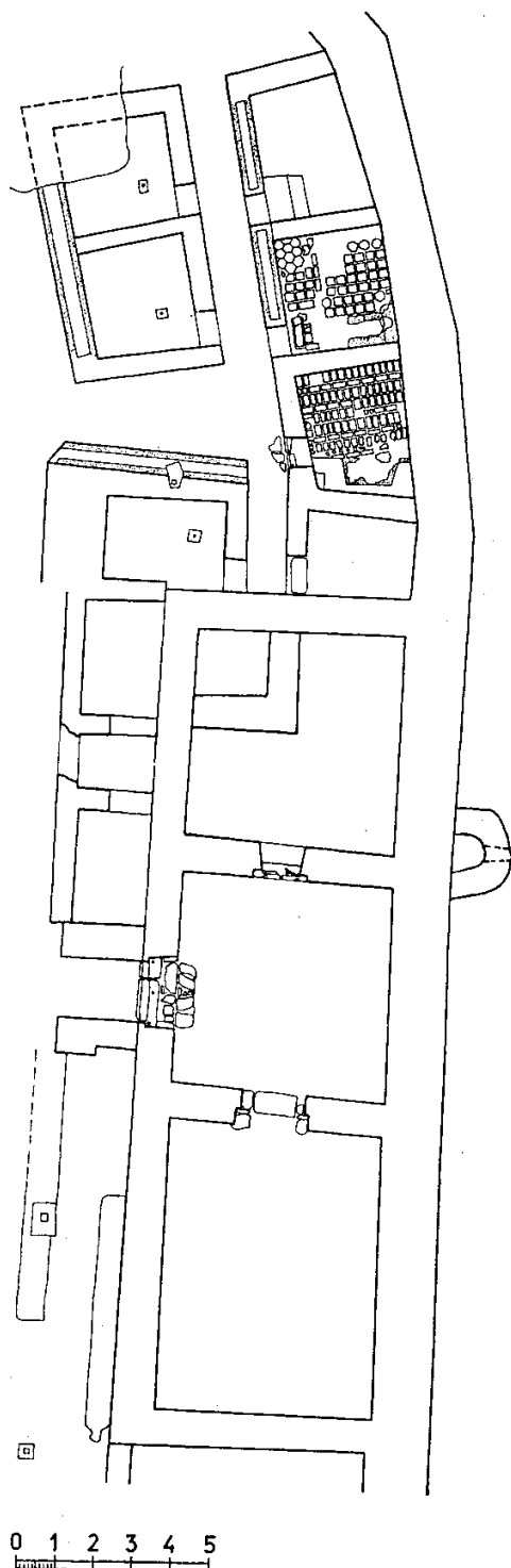
Сл. 25. Основа јужних грађевина Fig. 25. Plan des bâtiments méridionaux
