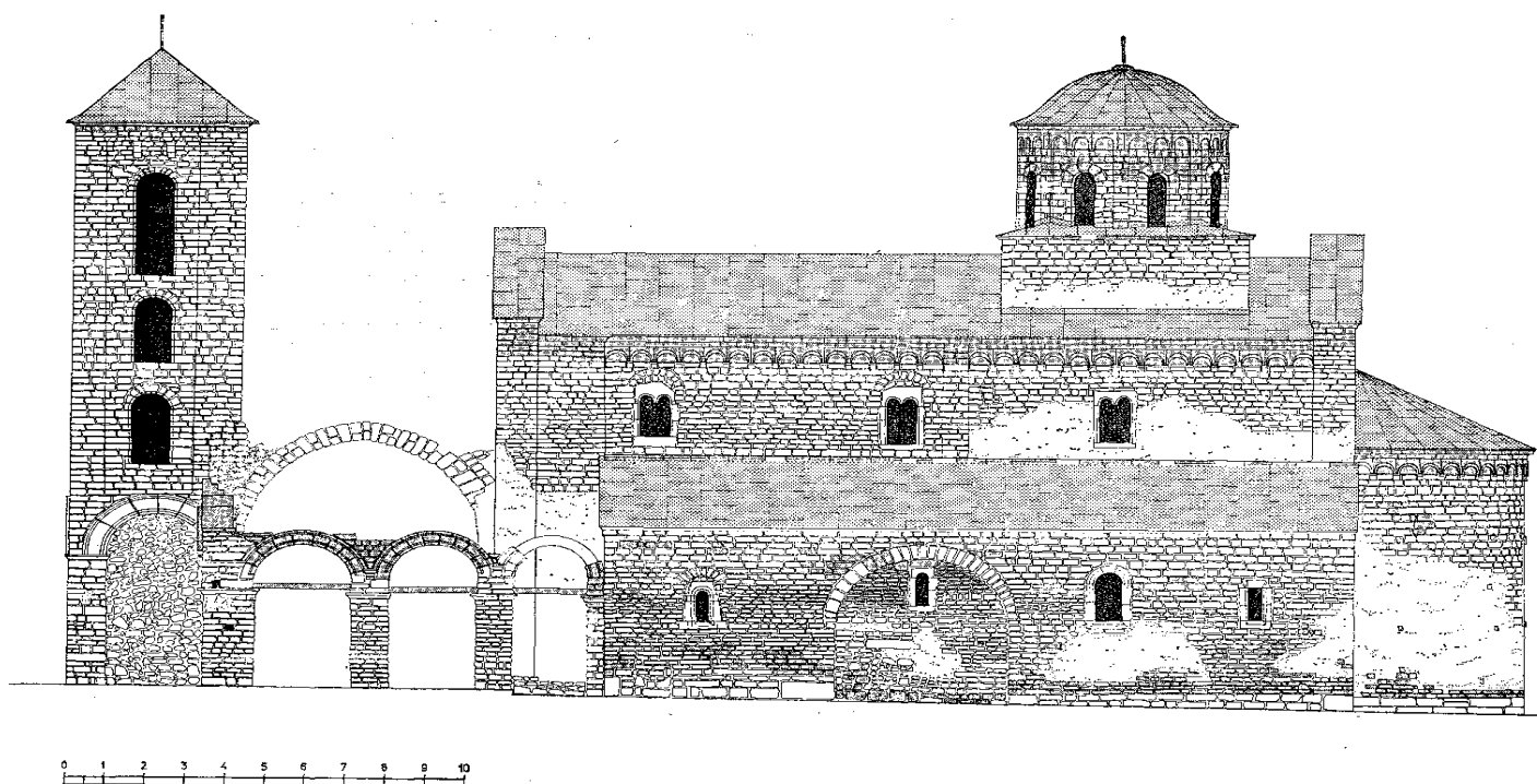
Fig. 14. L'église vue du sud, avec indication des parties restaurées ou échangées
