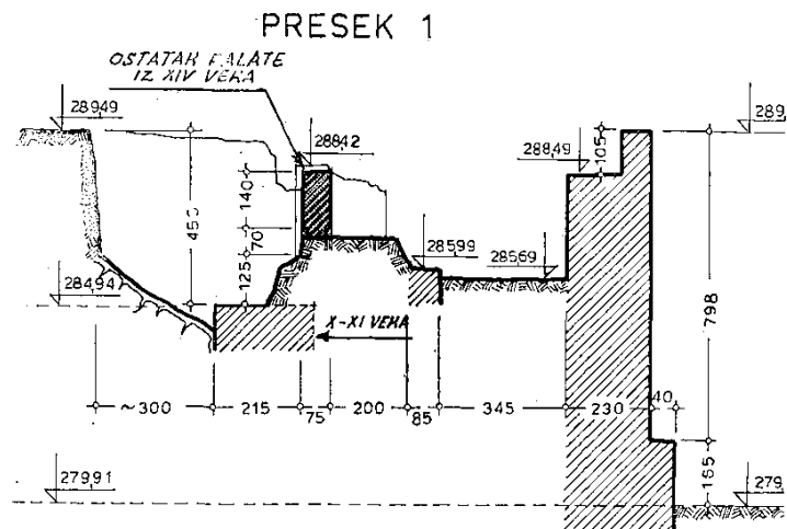
Сл. 3. Пресек 1—1 кроз преостале зидове средњовековног града у Скопљу који су приказани на плану — сл. 2. Из овог цртежа јасно се види њихов хронолошки однос
