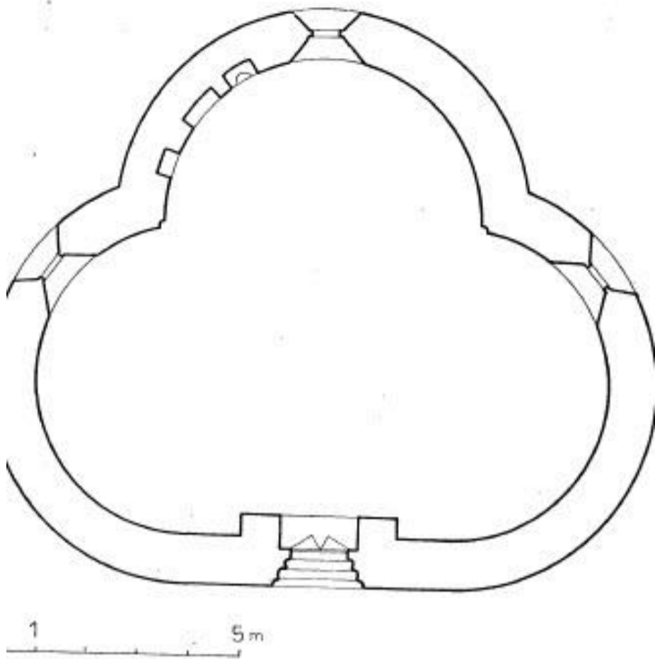
Сл. 3. Основа цркве светог Пантелејмона код села Торња (све цртеже урадио арх. др Војислав Матић коме дугоујем искрену захвалност) Fig. 3. Le plan de l'église Saint-Pantaléon près du village de Toranj (Tous les dessins ont été faits par l'architecte Vojislav Matić à qui nous exprimons ici notre gratitude sincère)
