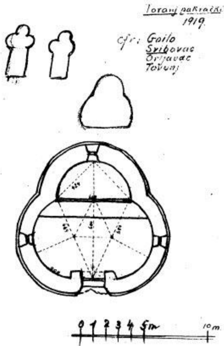
Сл. 19. Основа цркве Светог Пантелејмона са пресецима и упоредним основама сродних цркава. (Цртеж оловком 1919. г.) Fig. 19. Plan et coupes de l'église Saint-Pantaléon; plans comparés d'autres églises similaires (Dessin au crayon de 1919)
