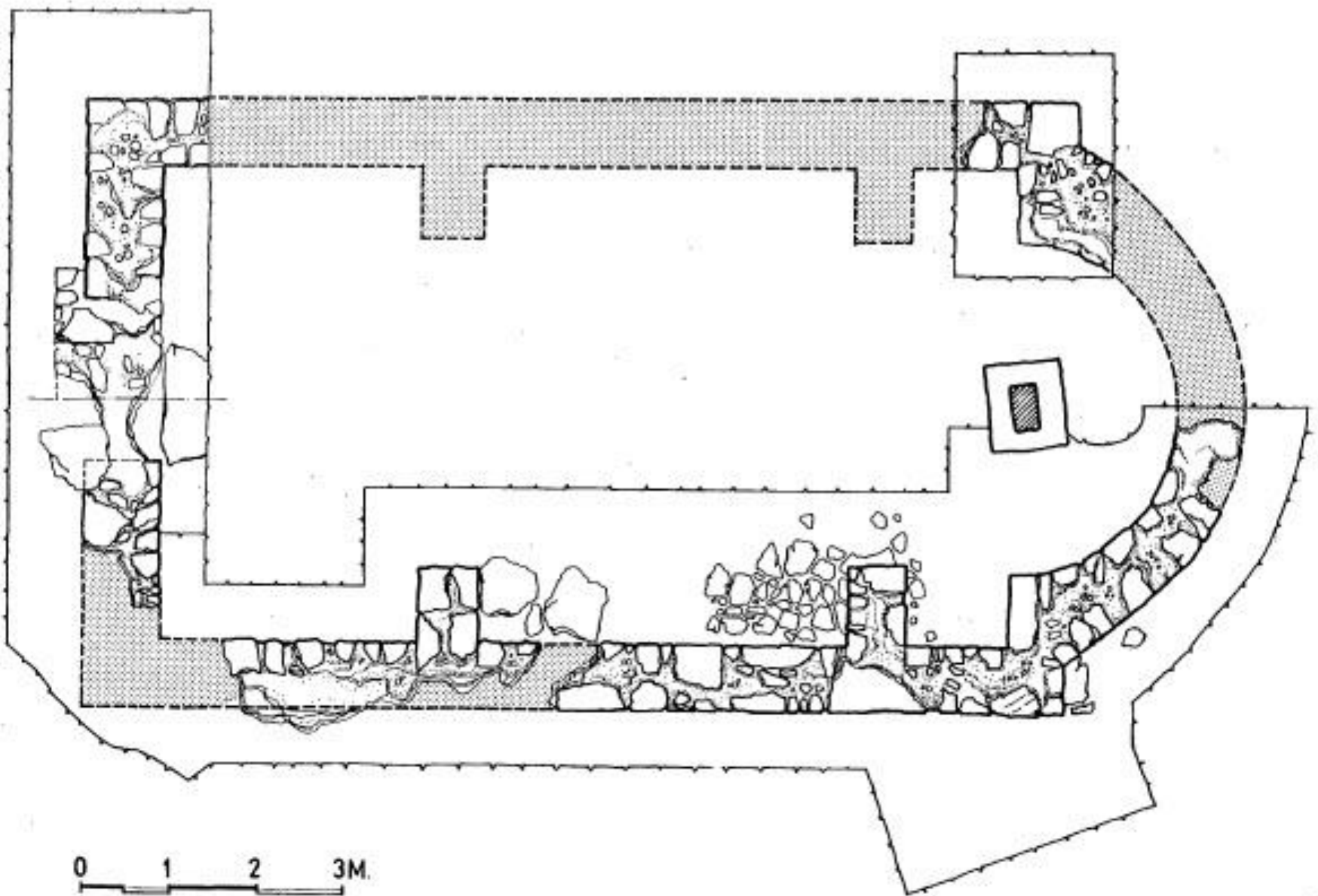
Сл. 3. Основа цркве
