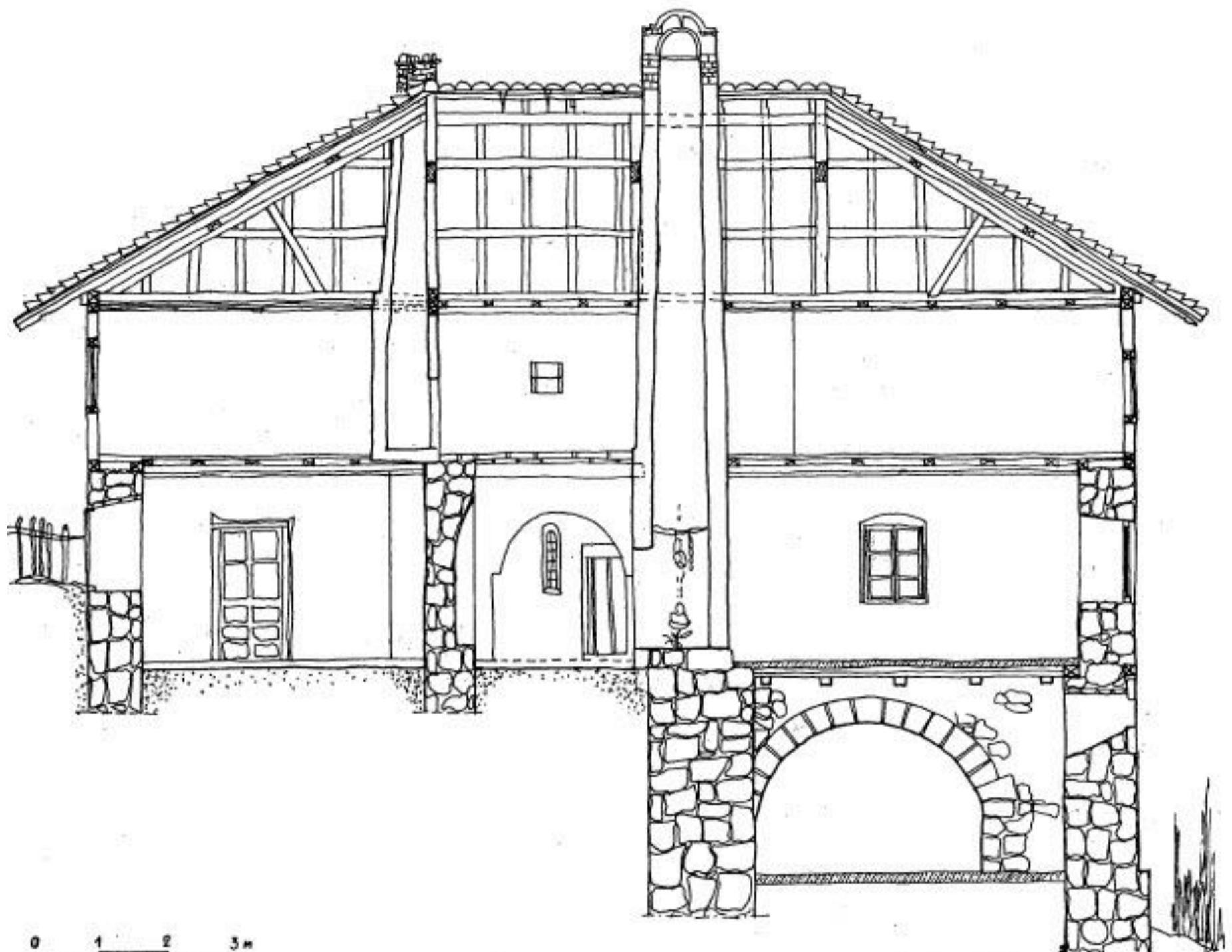
Fig. 8. La coupe transversale du bâtiment d'hébergement
