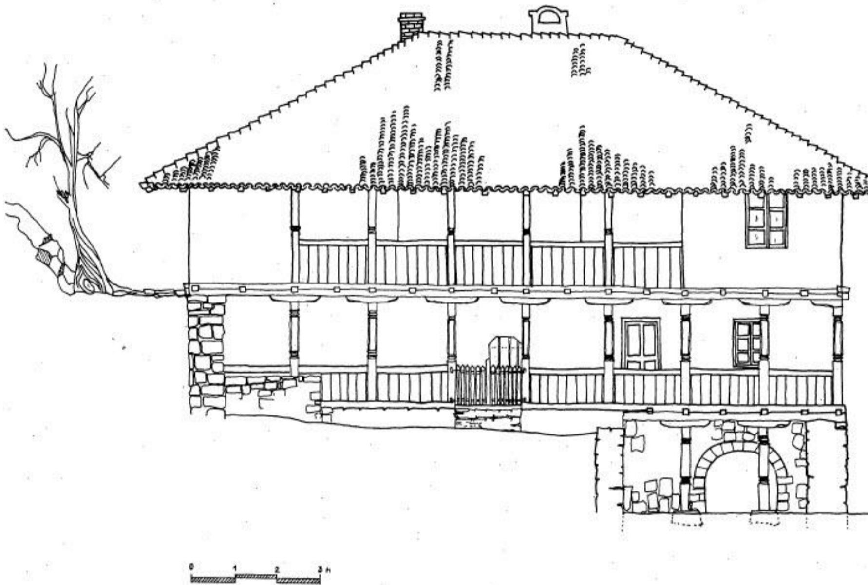
Сл. 9. Изглед реконструисаног конака. (Сви цртежи су арх. А. Гајића из документације Завода за заштиту споменика културе у Крагујевцу)
