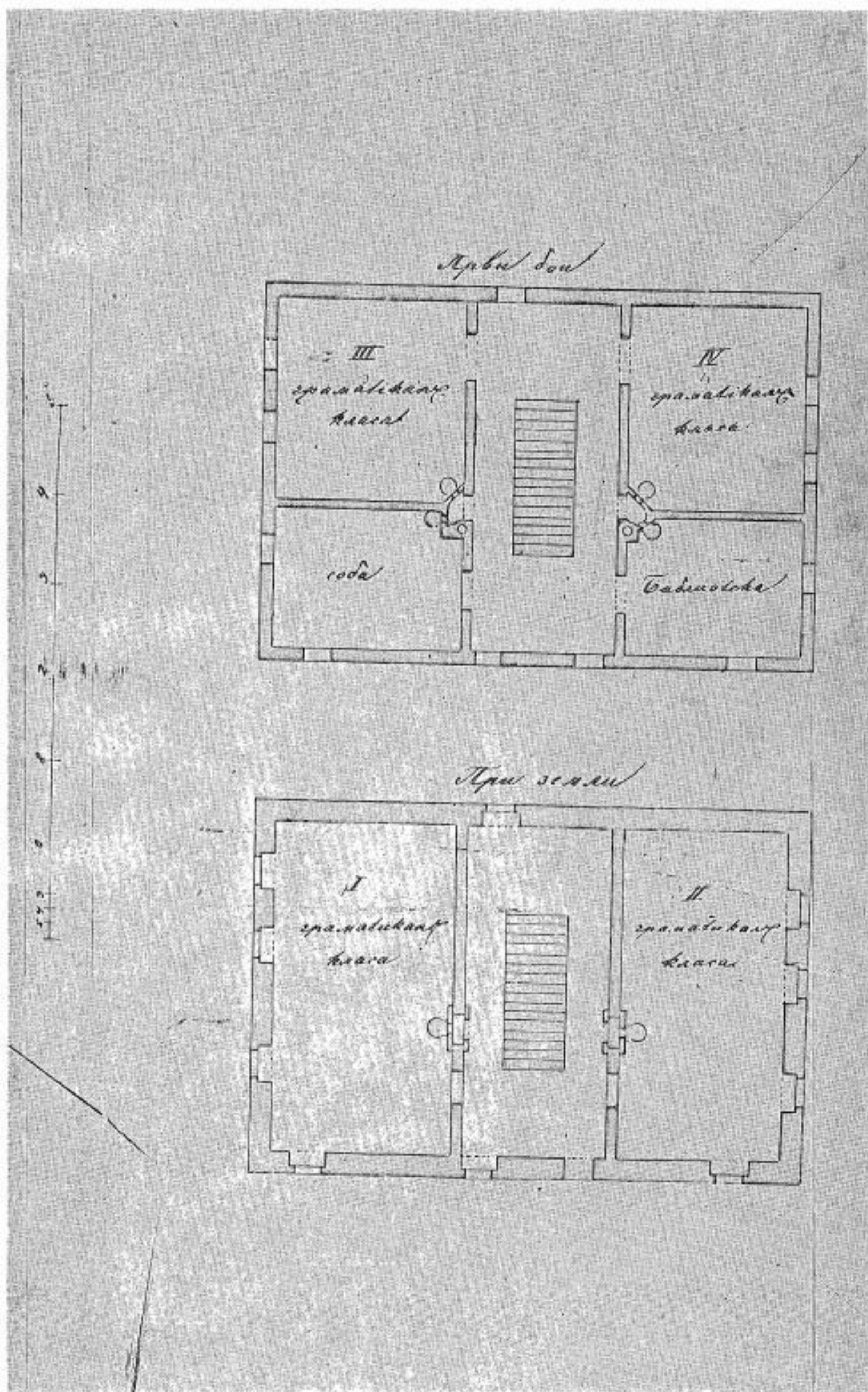
Сл. 6. Предлог за преуређење куће Јована Павловића за потребе Полушколазе шабачке
