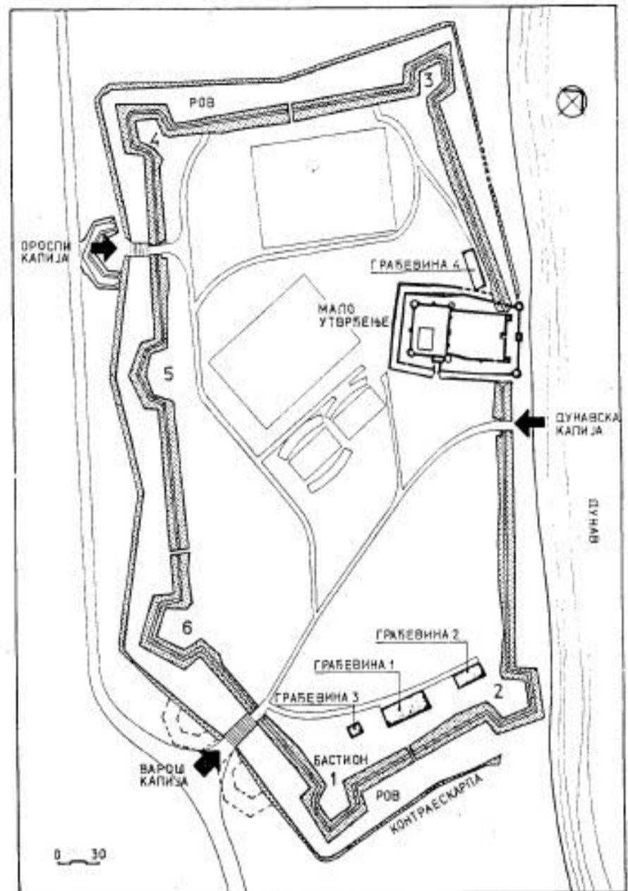
Сл. 14. Велико утврђење Фетислам, основа Fig. 14. Fétislam, la Grande forteresse, plan
