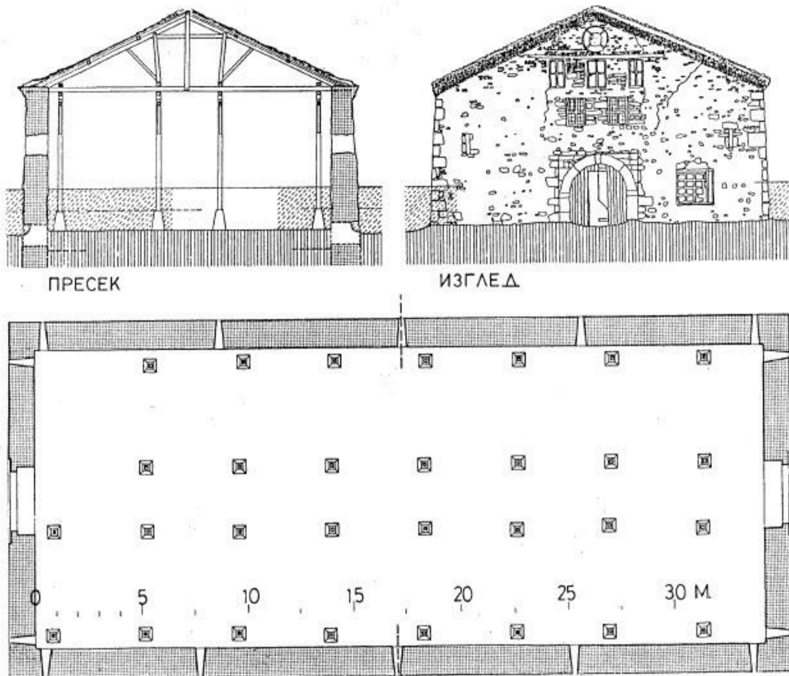
Сл. 21. Топхана — основа, пресек и изглед
