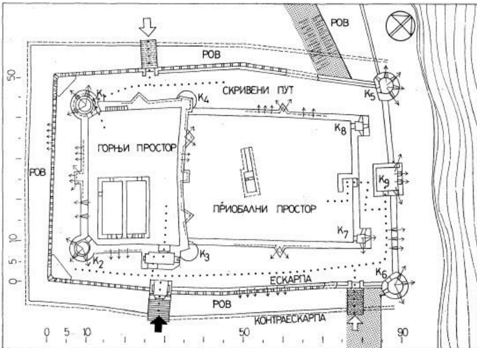
Fig. 1. Fétislam, la Petite fortification, plan — Analyse de la structure de la fortification
