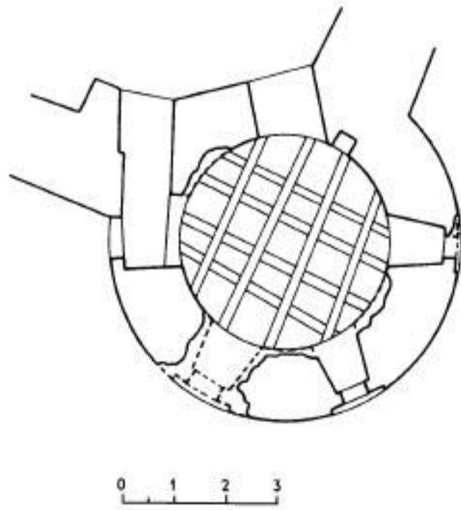
Сл. 2. Мало утврђење, кула K_1 — основа и пресек Fig. 2. La Petite fortification, tour K_1 — plan et coupe
