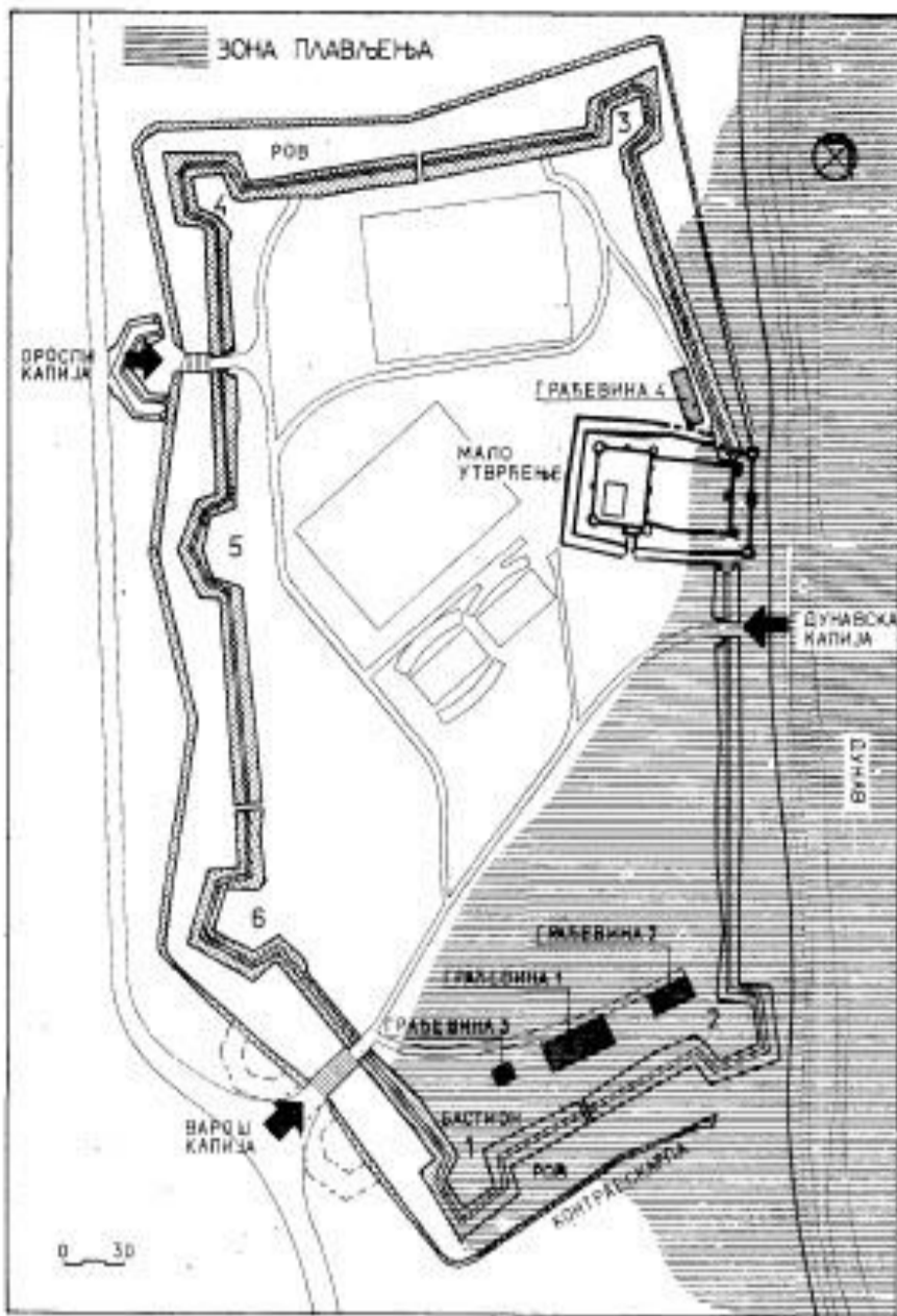
Сл. 22. Основа Великог града — угроженост успором Дунава
