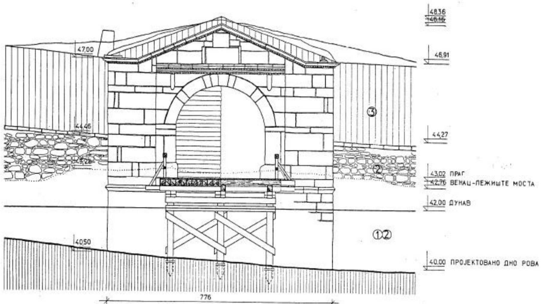
Сл. 17. Велико утврђење, Варош капија (реконструкција арх. Д. Тодоровић)
