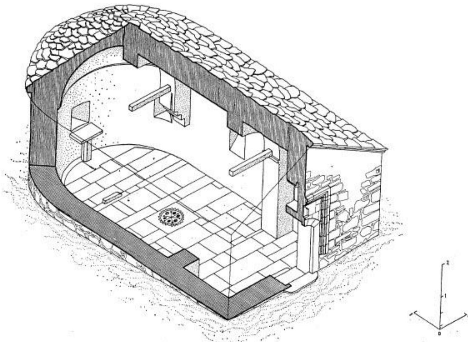
Сл. 8. Аксонометријски приказ првобитног конструктивног склопа ковачевске цркве
