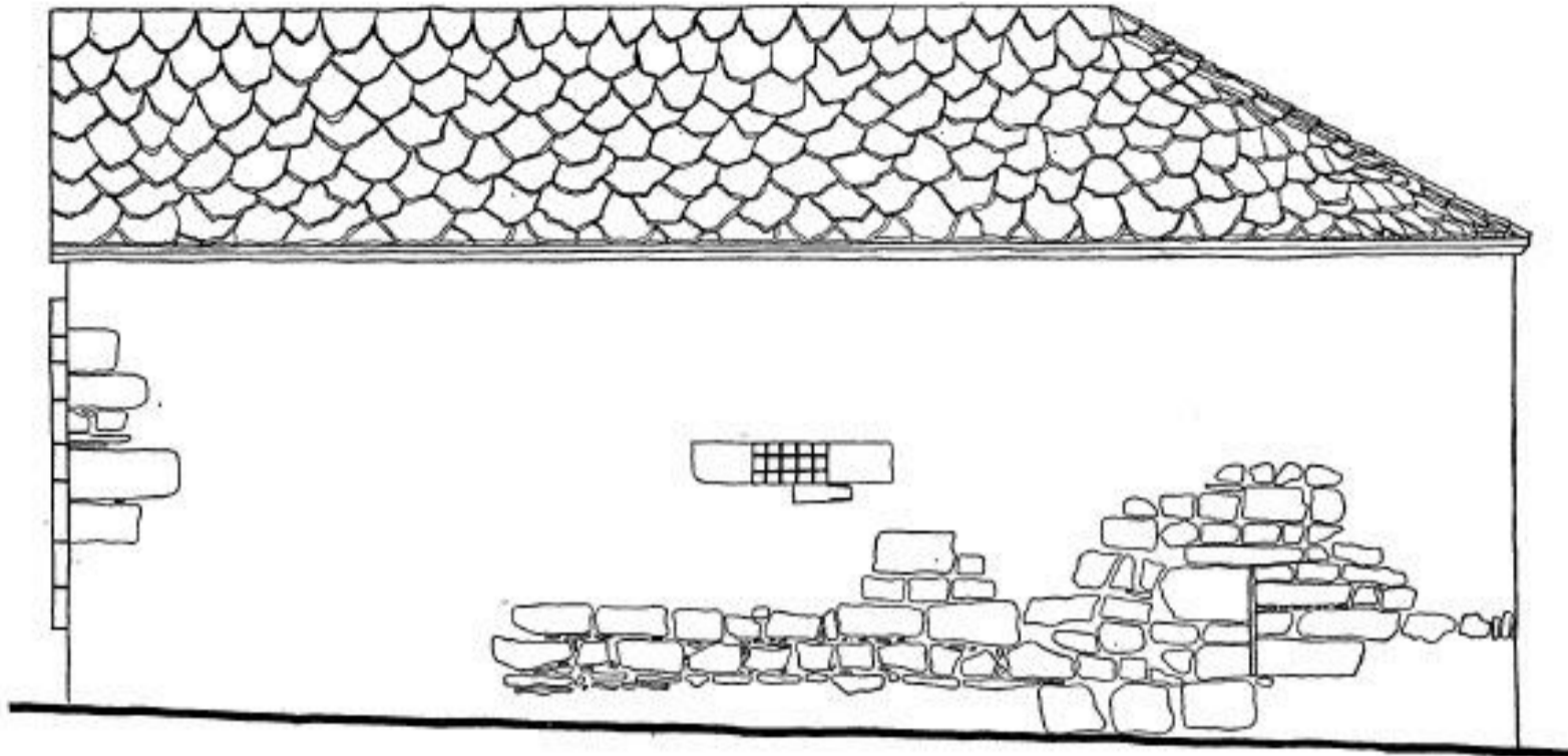
Сл. 6. Западни и јужни изглед цркве у Ковачеву и реконструкција некадашњег изгледа
