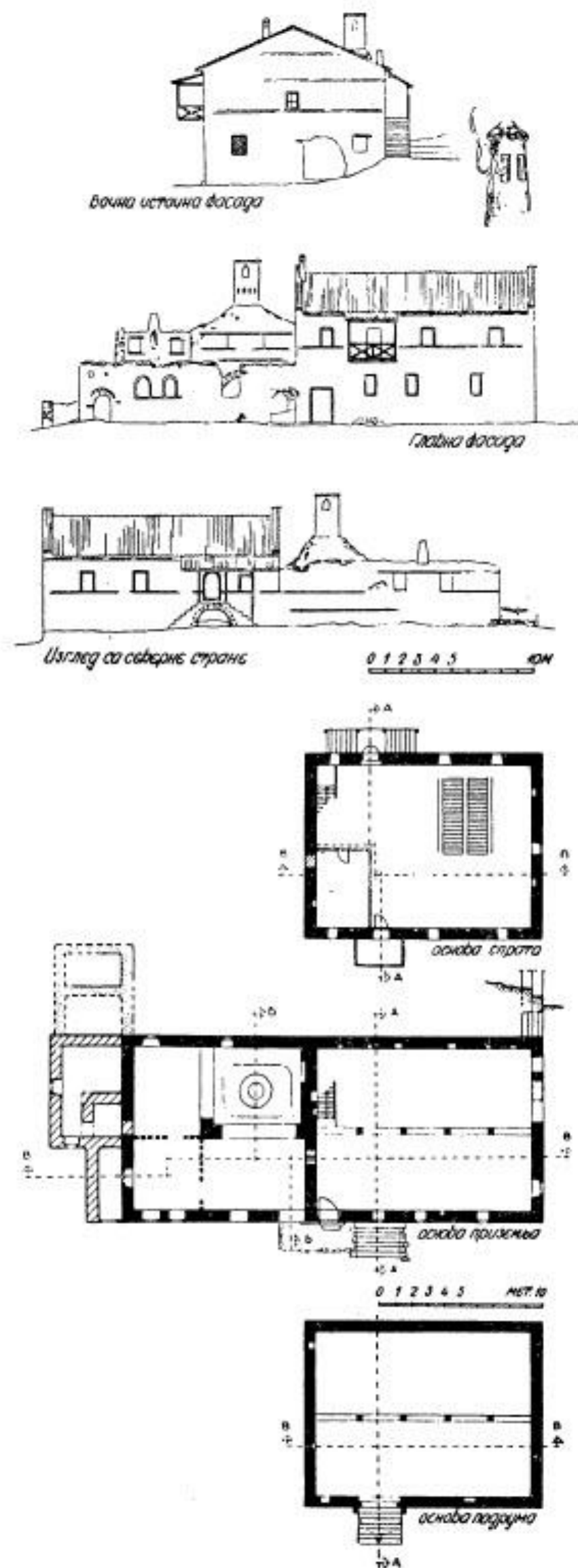
Сл. 17. Стари конак — стара трпезарија у Пећкој Патријаршији, стање пред рушење. Цртеж Б. Вуловића
