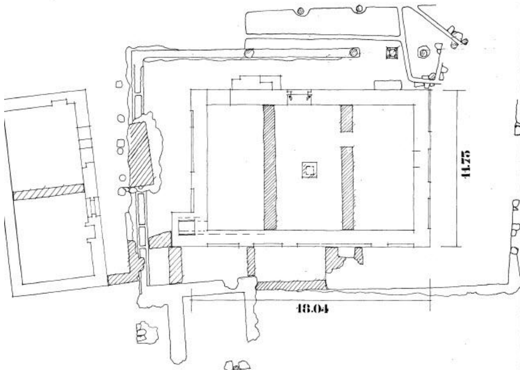
Fig. 5. Plan du palais mis au jour, comprenant le dessin des vestiges des murs dont la majeure partie date d'une époque postérieure
