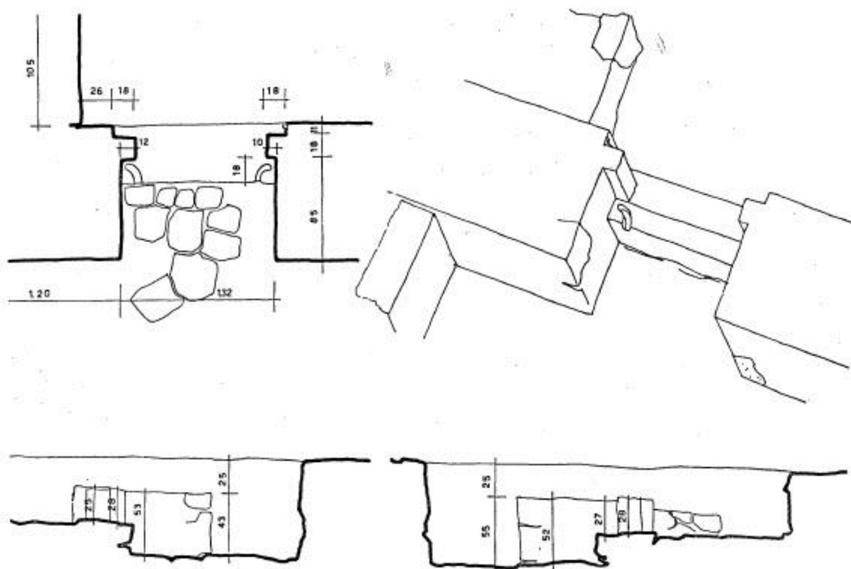
Fig. 7. Vestiges d'une porte dans le mur nord. Plan, aspects latéraux, axonométrie
