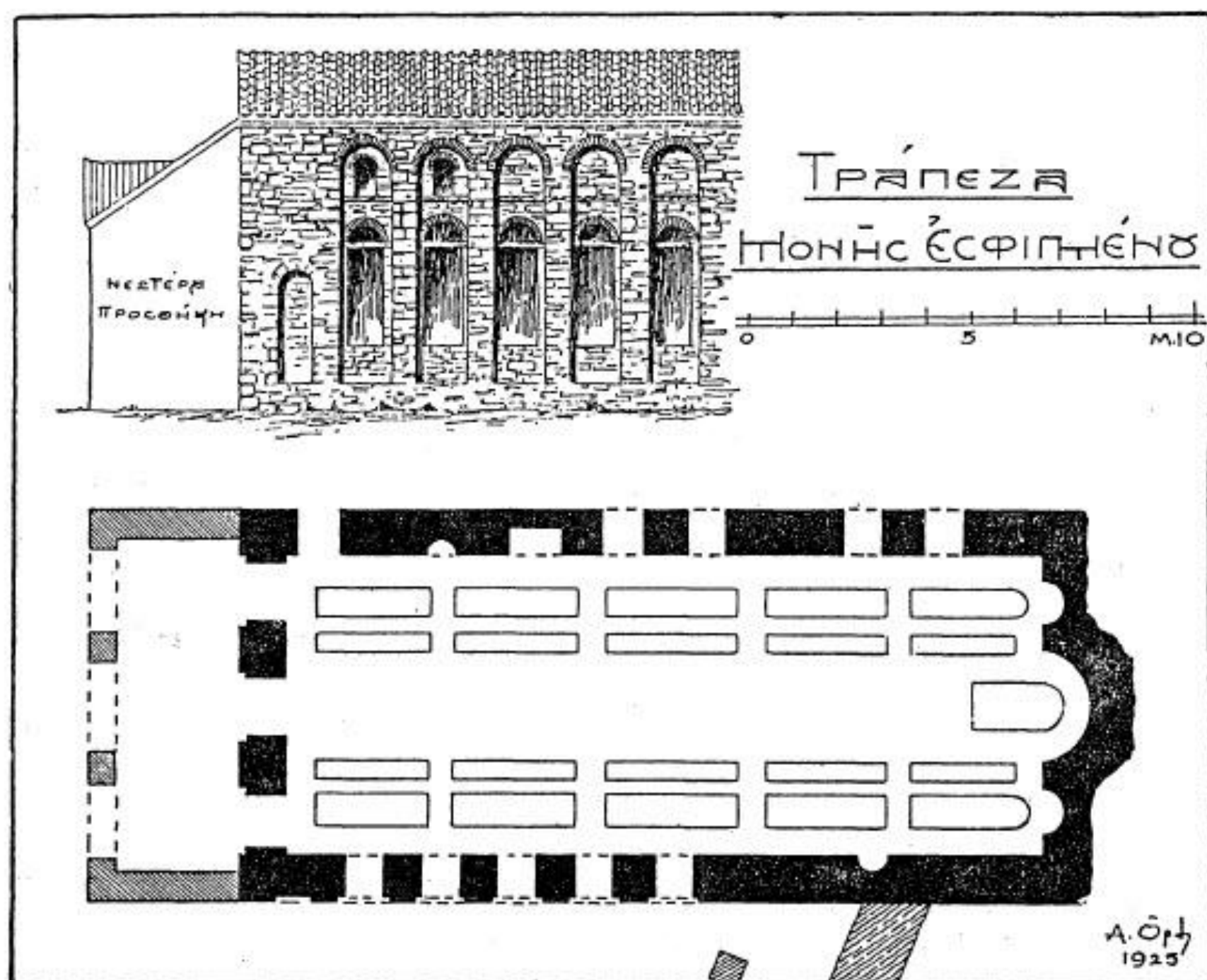
Fig. 15. Réfectoire du monastère d'Esphigmen. Reproduction du dessin d'A. K. Orlandos
