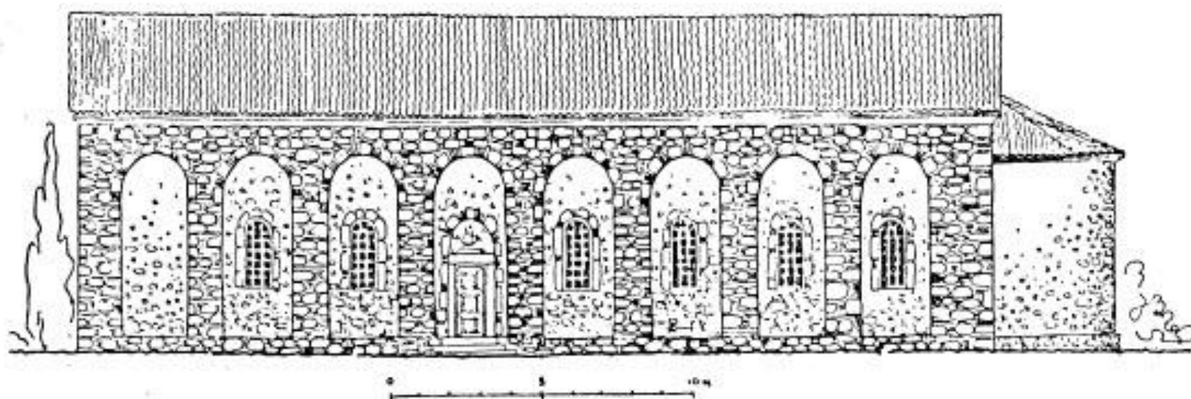
Fig. 14. Réfectoire du monastère de Dečani, reconstitution. Vue du sud. D'après S. Nenadović, réfectoire du protomaître Georges au monastère de Dečani
