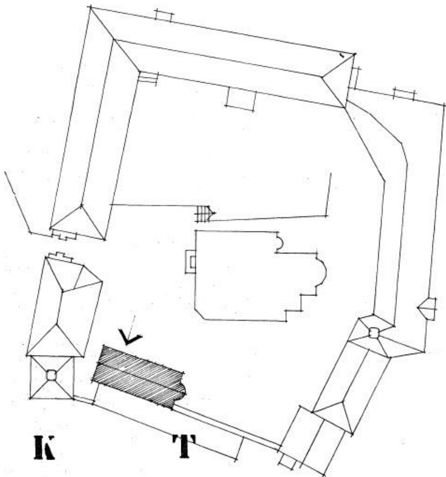
Fig. 10. Réfectoire du monastère de Treskavac, peut-être le seul réfectoire de notre pays où il subsiste une cuisine à foyer et tables de pierre originelles. Les dessins montrent, en plus de la situation, le bâtiment du réfectoire avec tables et bancs, le plan et la coupe de la cuisine, une porte donnant accès à la cuisine à foyer et une des tables. Seule une petite partie des tables, faites de blocs de pierre massifs, d'une longueur de 3,80 m, avait été achevée et décorée d'ornements; ceux-ci sont reproduits sur le dessin. Il convient de mentionner que dans le récent incendie tous les bâtiments d'hébergement accolés à l'église furent complètement brûlés, sauf le réfectoire en fut épargné
