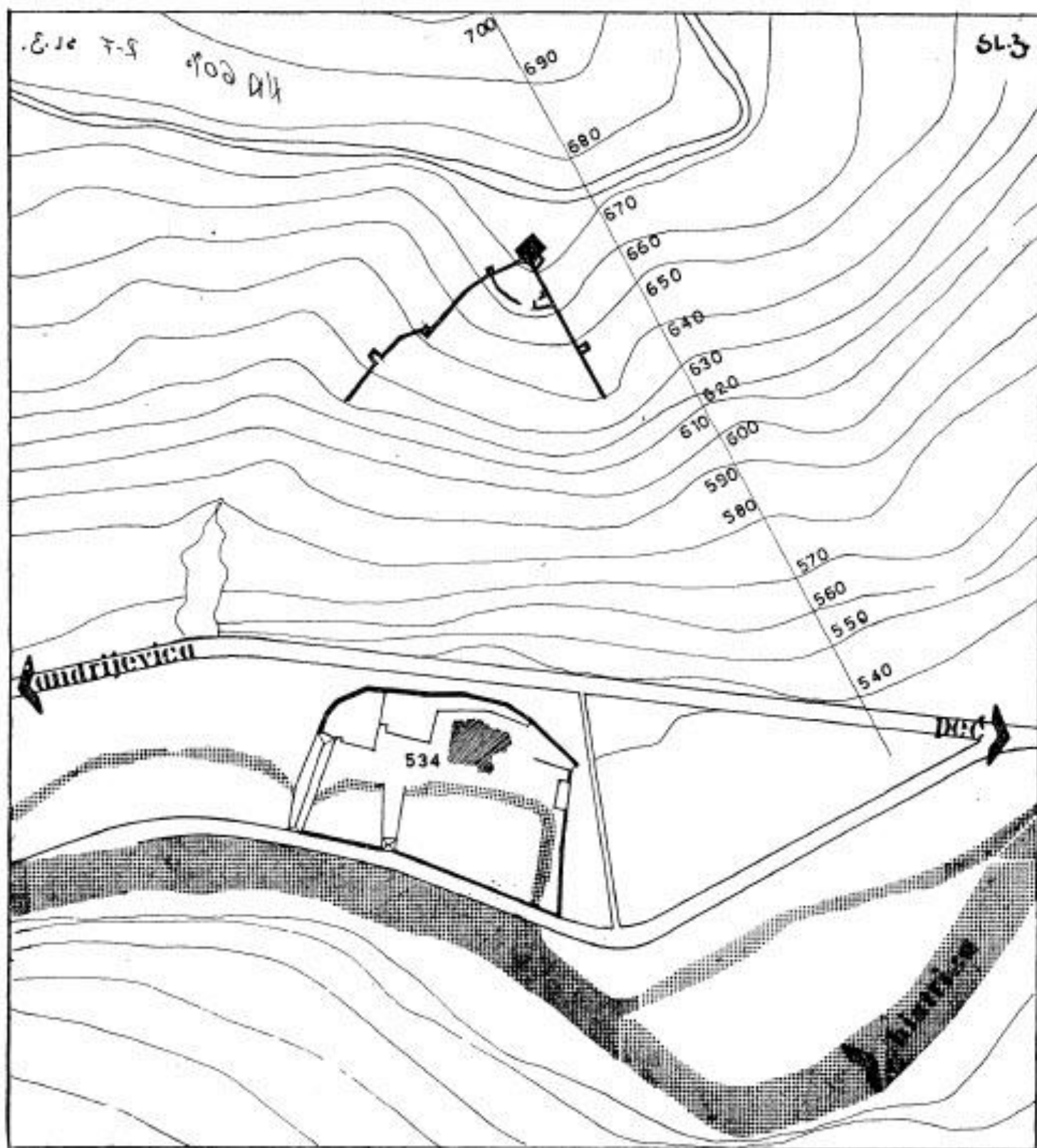
Сл. 3. Ситуациони план манастира са ближом околином и уцртаним остацима зидова утврђења који су откривени 1965—66. године
