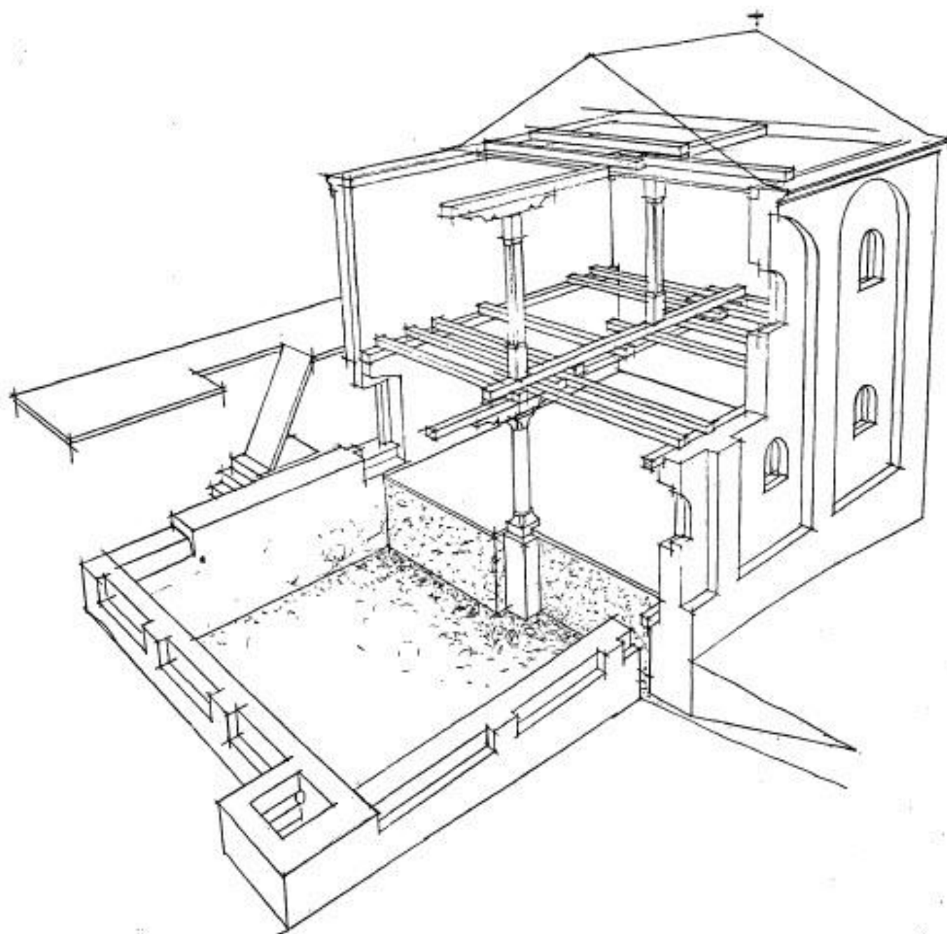
Сл. 8. Вероватни изглед и конструктивни склоп палате
