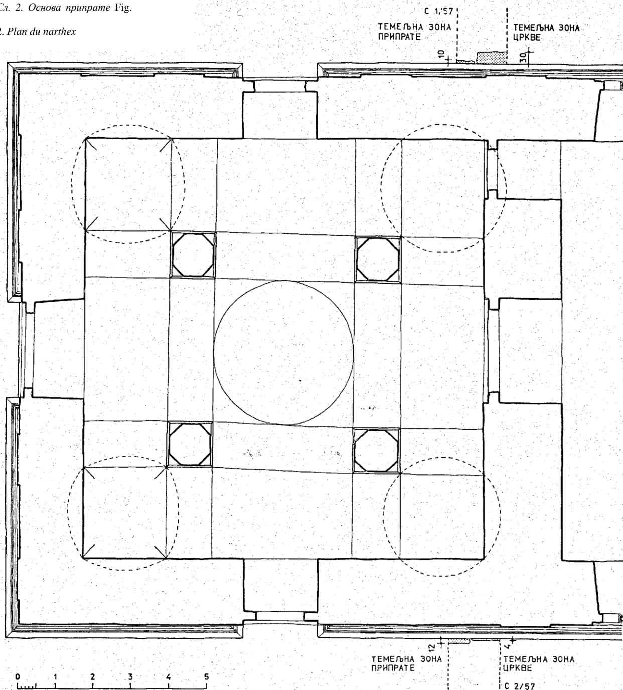
Сл. 2. Основа припрате Fig.
