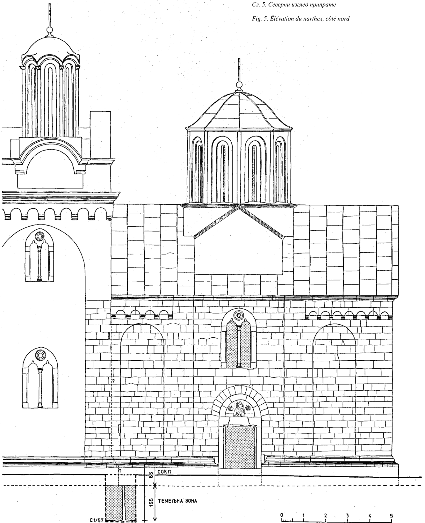
Сл. 5. Северни изглед припрате
