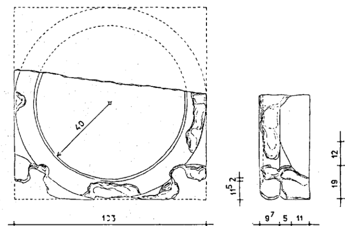
Сл. 8. Стопа стуба припрете (стопа из Смедерева снимила арх. Г. Симић)
