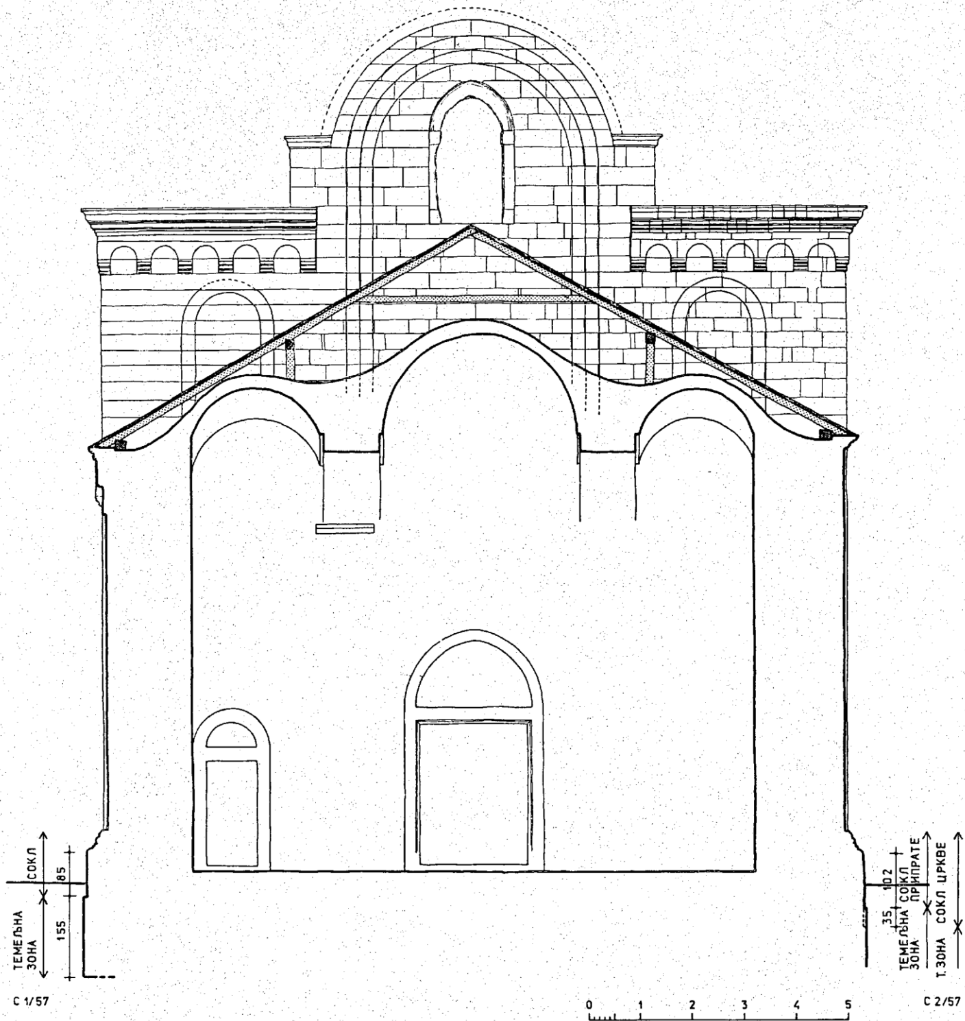
Сл. 4. Попречни пресек кроз источне сводове приправе
