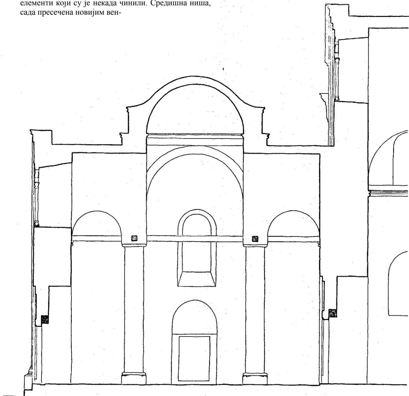
Fig. 10. Coupe longitudinale du narthex — reconstitution
