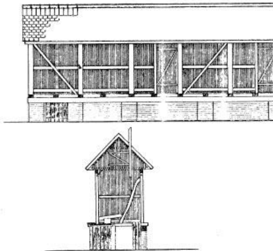
Сл. 17. Чардак — салаш Стрилић (В. Ковачевић)
