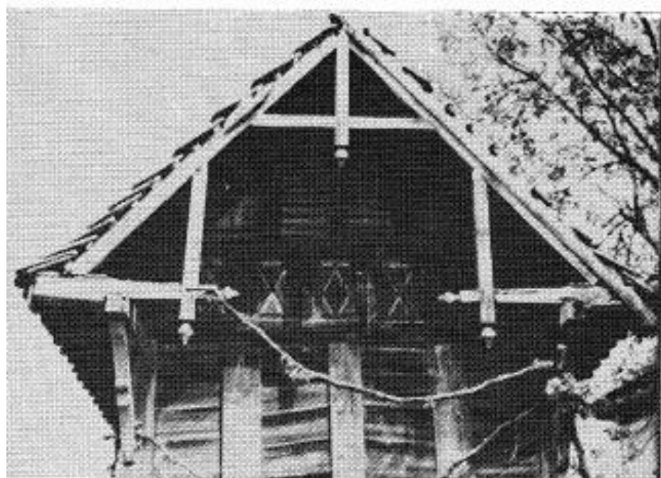
Сл. 8. Амбар, препуштена настрешница над забатом — Мартинци, Сремска 121
