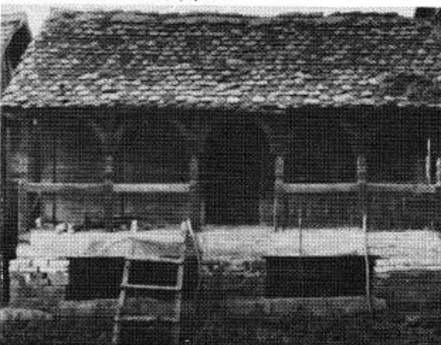
Сл. 12. Амбар са отвореним тремом — Шид, М. Пијаде 62, стуб трема са годином изградње зграде
