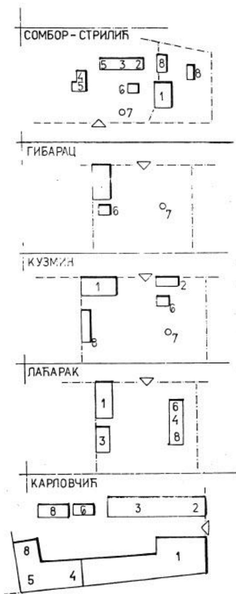
Fig. 1. Situation de l'ambar et du tchardak dans une propriété rurale (dessin dû à l'architecte Ilija Protić)
