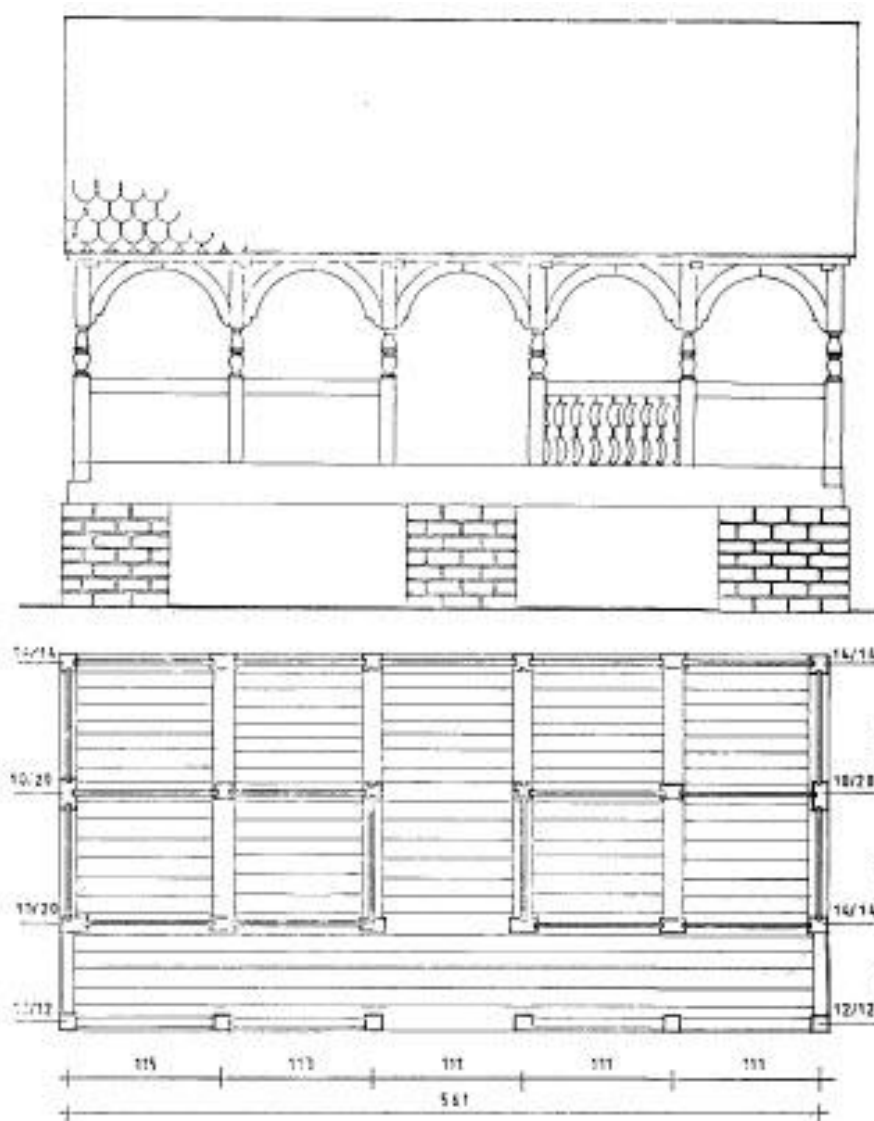
Сл. 5. Амбар са тремом на дужој страни — Карловчић (С. Темерински, В. Томашевић)
