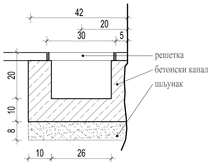
ПРЕСЕК А-А
