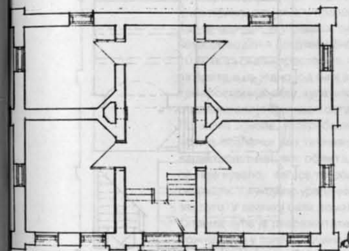
Слика 11. Мали Борак, конак Михаиловића: а) основа приземља, б) основа спрата в) пресек 2.2, г) улазни изглед
