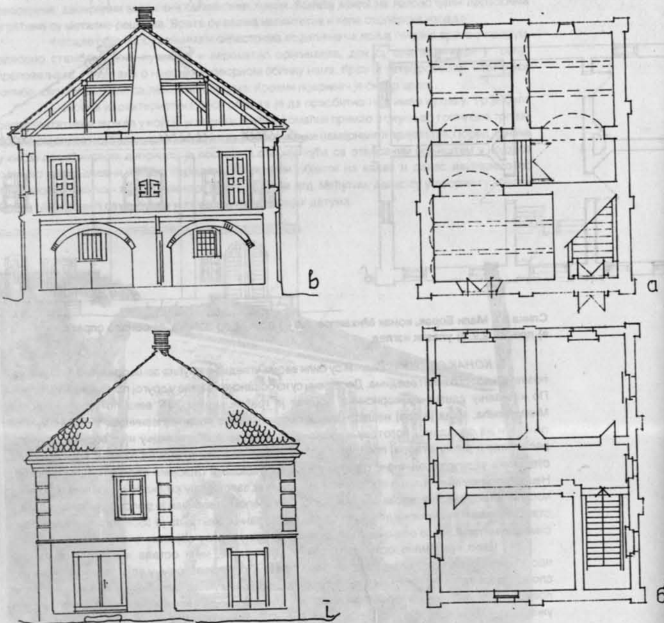
Слика 12. Мали Борак, конак Радића: а) основа приземља, б) основа спрата, в) пресек 1-1, г) улазни изглед
