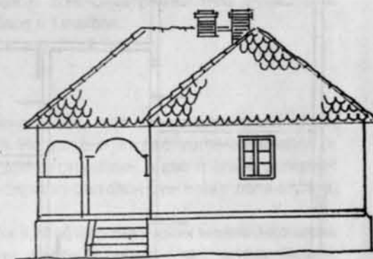
Слика 17. Велики Црњени, кућа Бабића: а) основа, б) улазни изглед
