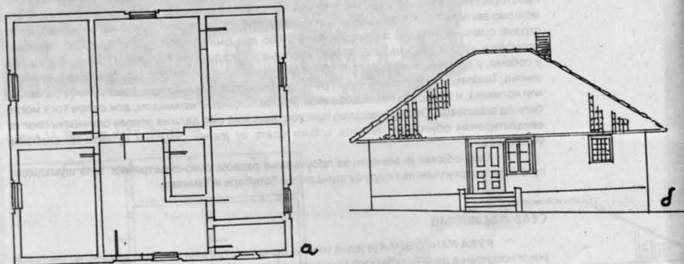
Слика 21. Јунковац, кућа Крцалића: а) основа, б) улазни изглед
