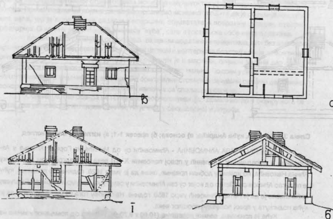
Слика 6. Каленић, кућа Аћимовића: а) основа; б) пресек 2-2; в) улазни изглед; г) бочни изглед
