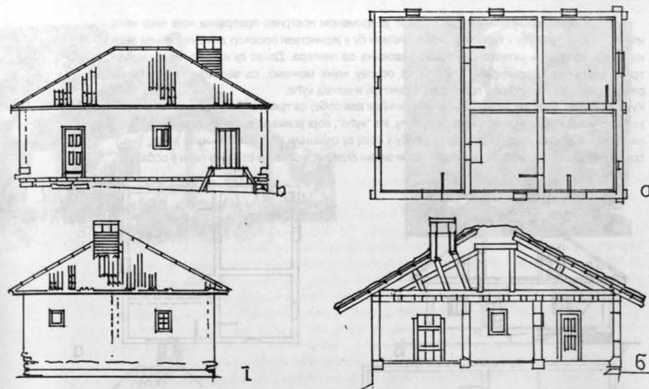
Слика 3. - Каленић, кућа Андрића: а) основа; б) пресек 1-1; в) изглед; г) бочни изглед
