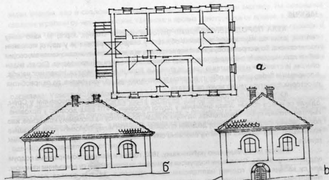
Слика 14. Јабучје, кућа Поповића: а) основа, б) продужени изглед, в) бочни изглед
