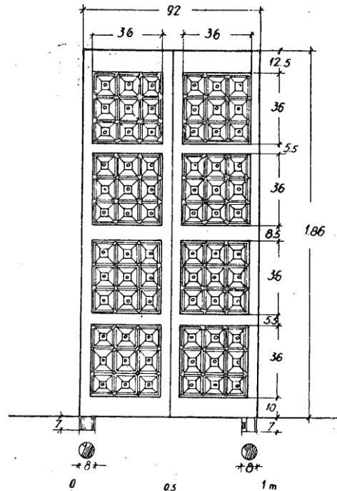
Сл. 5. Манастир Стјеник, стара дрвена улазна врата. — Fig. 5. Le monastère Stjenik, la vieille porte d'entrée en bois.
