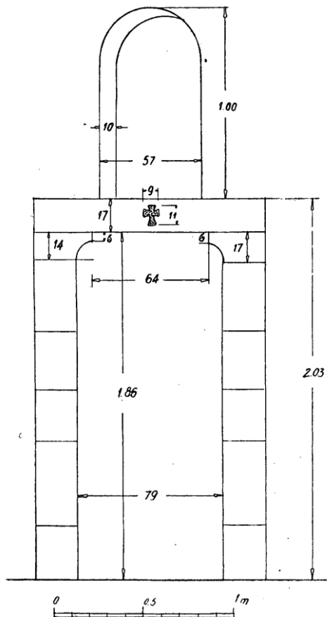
Сл. 4. Манастир Стјеник, главни улаз. Fig. 4. Le monastère Stjenik; entrée principale.
