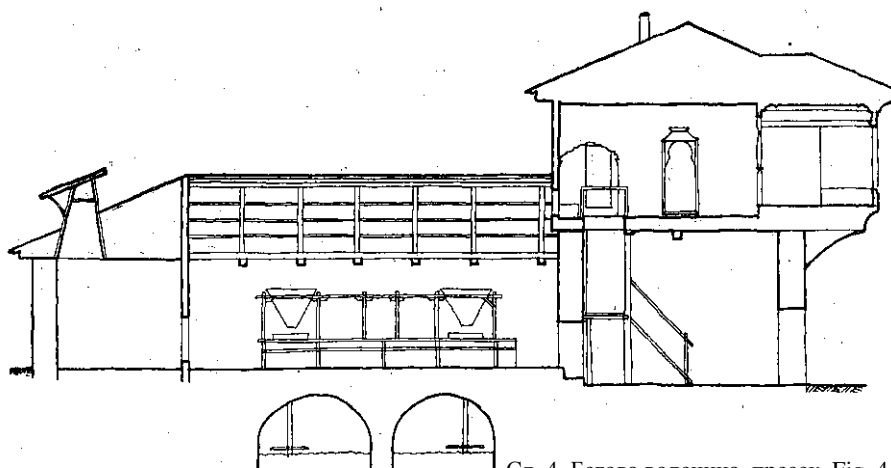
ПОДУЖНИ ПРЕСЕК
