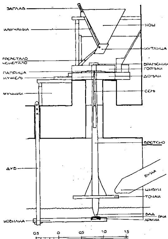
Сл. 7. Бегова воденица, скица млинског уређаја. — Fig. 7. Moulin de Bey, schéma des installations de meunerie.
