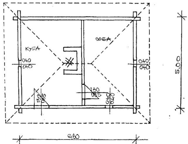
цртеж 1. Основа куће брвнаре у Коњуши
