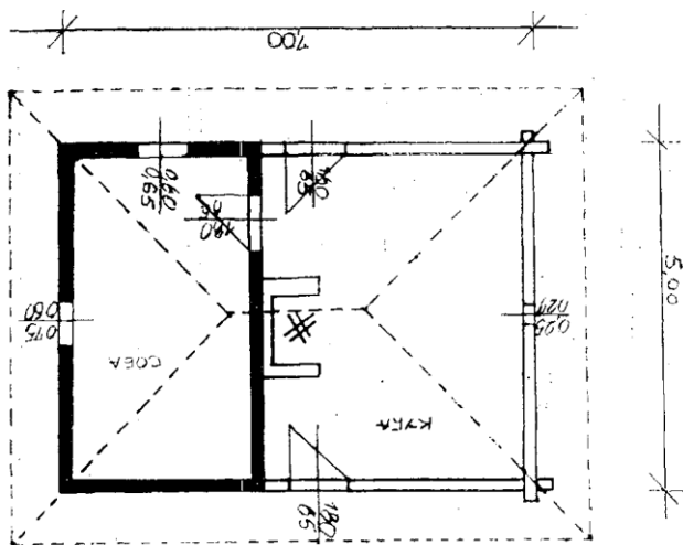
цртеж 2. Основа куће полубрвнаре у Лесковцу
