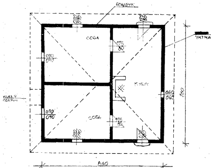
цртеж 4. Основа куће четмаре у Топоници
