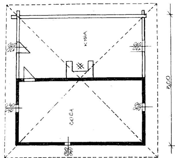
цртеж 3. Основа куће полубрвнаре у Гунцатима
