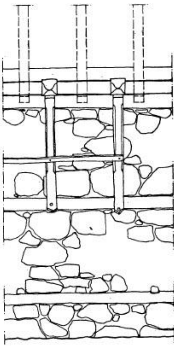
Fig. 6. Moulin à eau du monastère, — les bouts façonnés des colonnes et des poutres.
