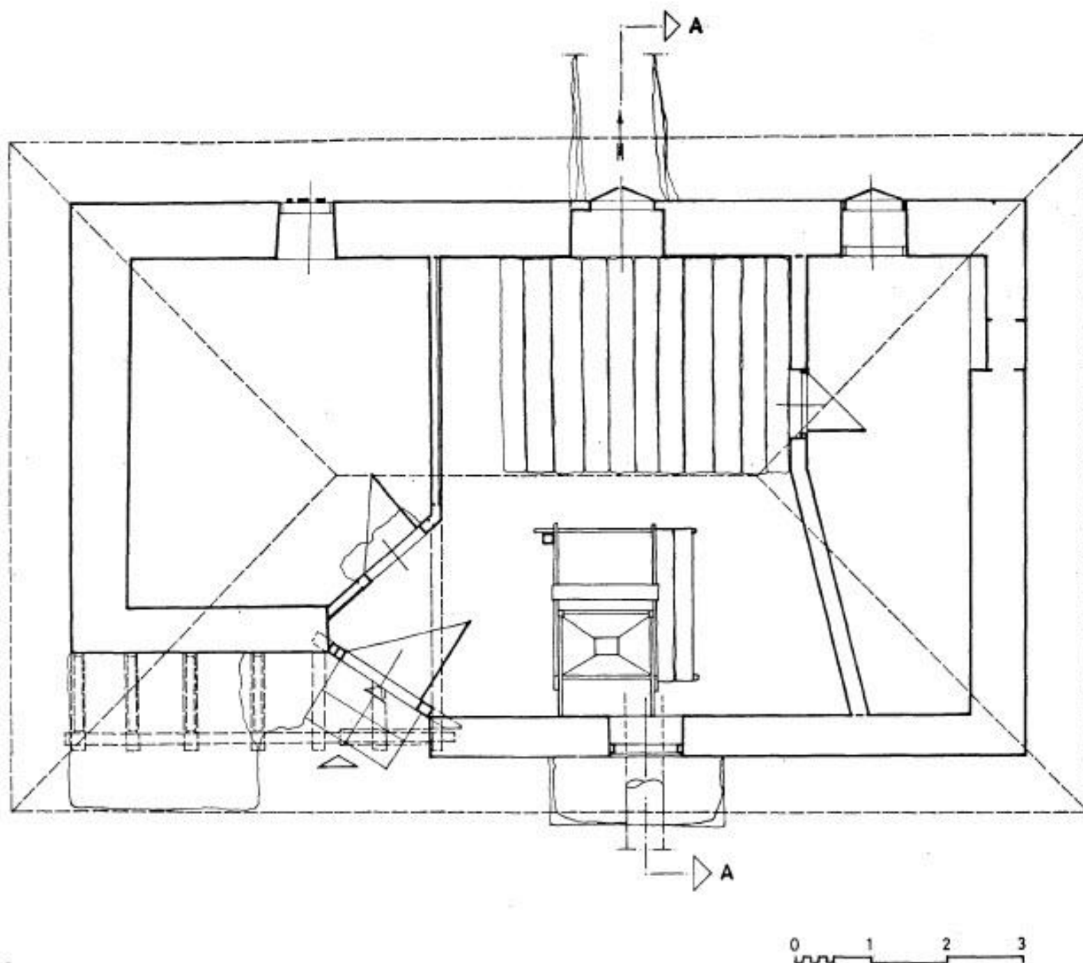
Сл. 7. Манастирска воденица — основа Fig. 7. Moulin à eau du monastère, — plan.
