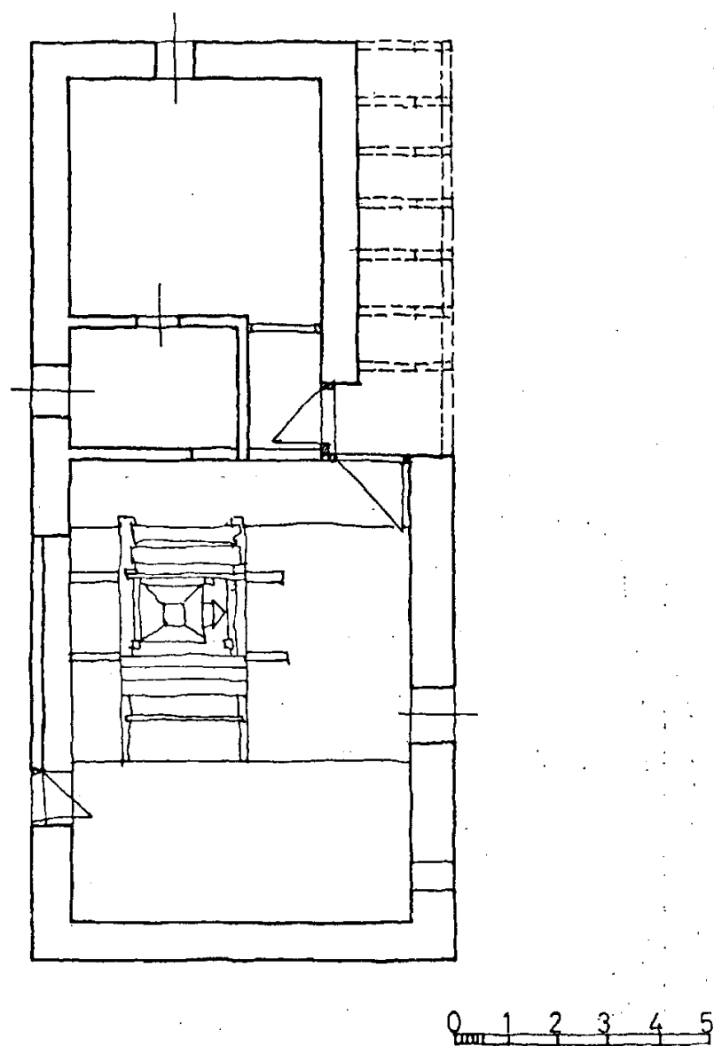
Сл. 11. Калајџијска воденица у Накривањском Чифлуку — основа Пример приземне воденице чију настрешницу носи група од седам извијених косника
