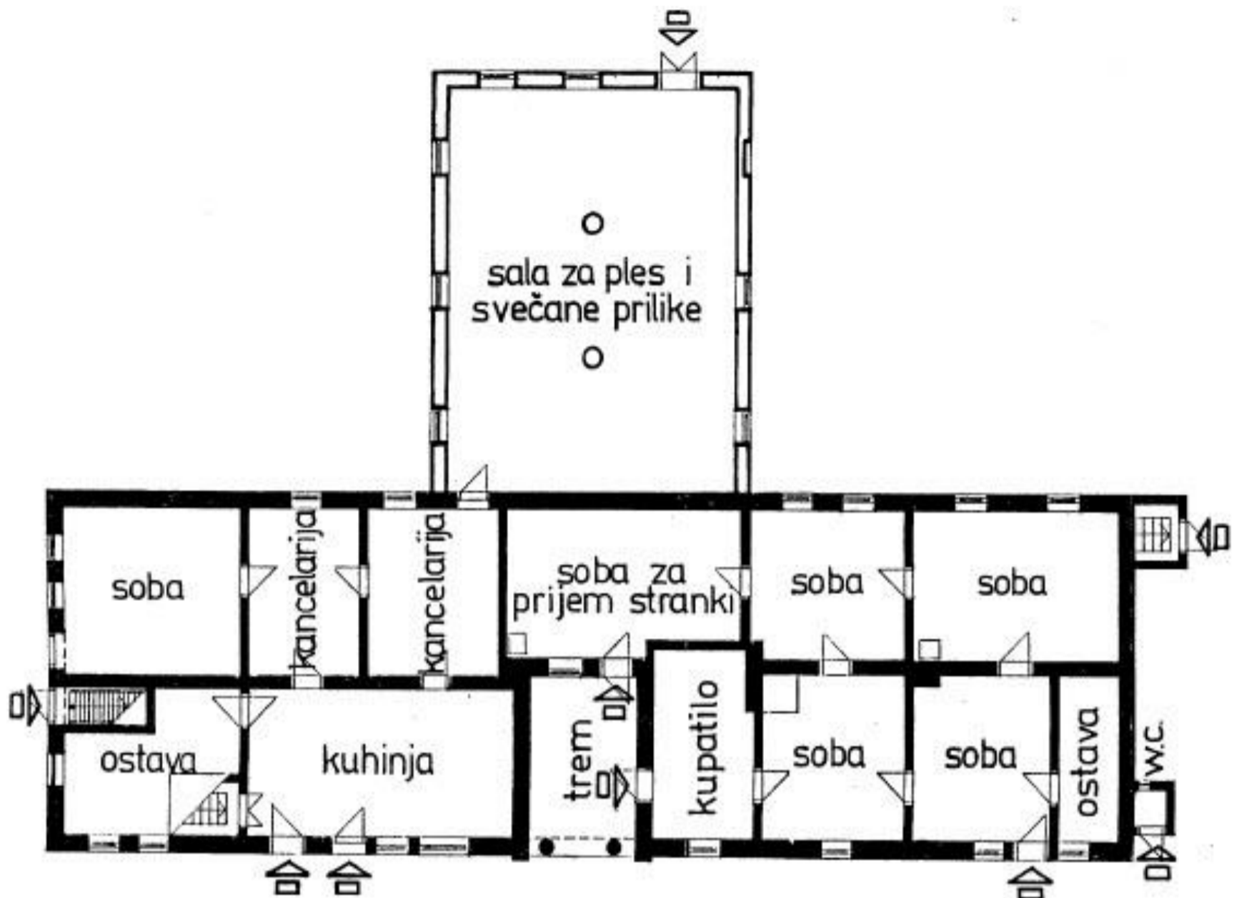
Сл. 1. Основа куће на мајуру Лелбах Буле (ПА „Зобнатица“ парцела бр. 2)
