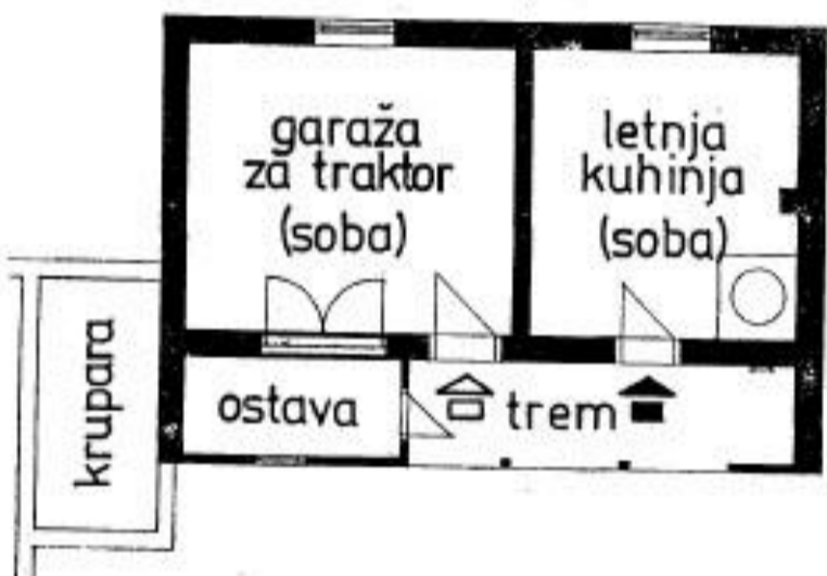
Сл. 7. Основа мале куће Јохана Мајера Fig. 7. Vue de la petite maison de Johannes Mayer
