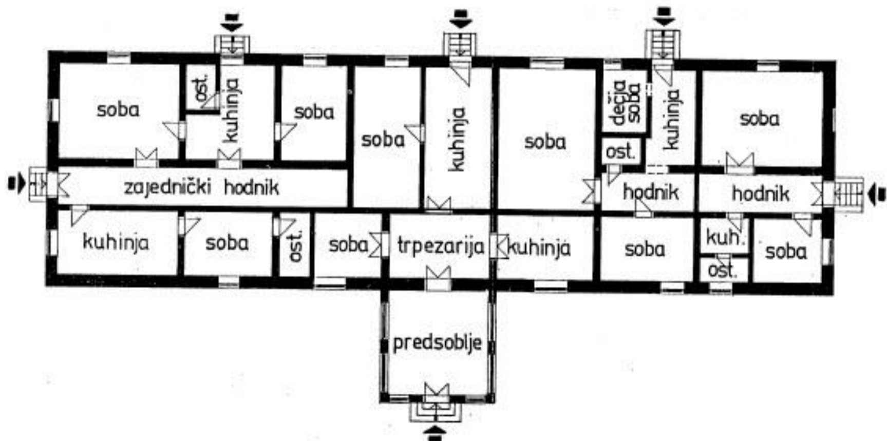
Сл. 3. Основа куће на мајуру Калмар Имреа (ПА „Зобнатица“ парцела бр. 4)
