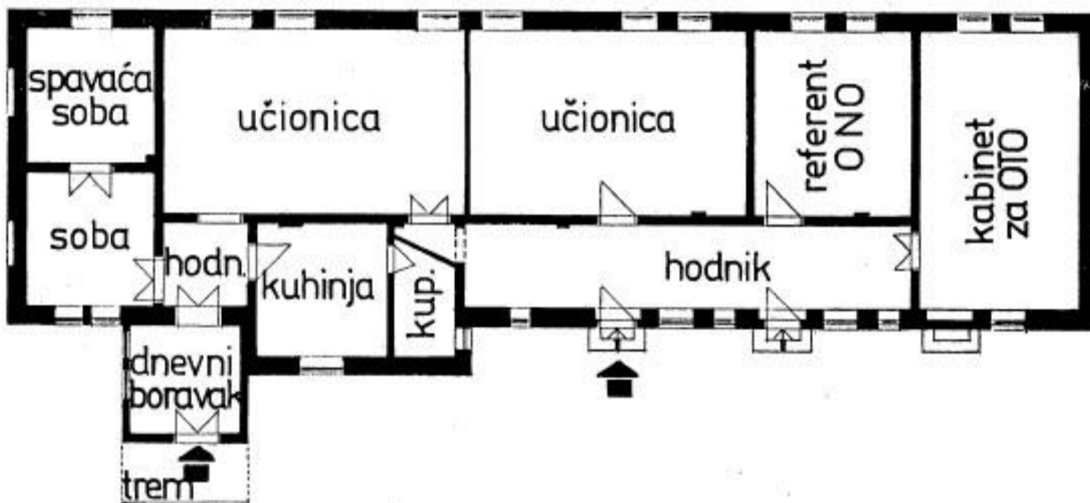
Сл. 9. Основа објекта у Хајдукову
