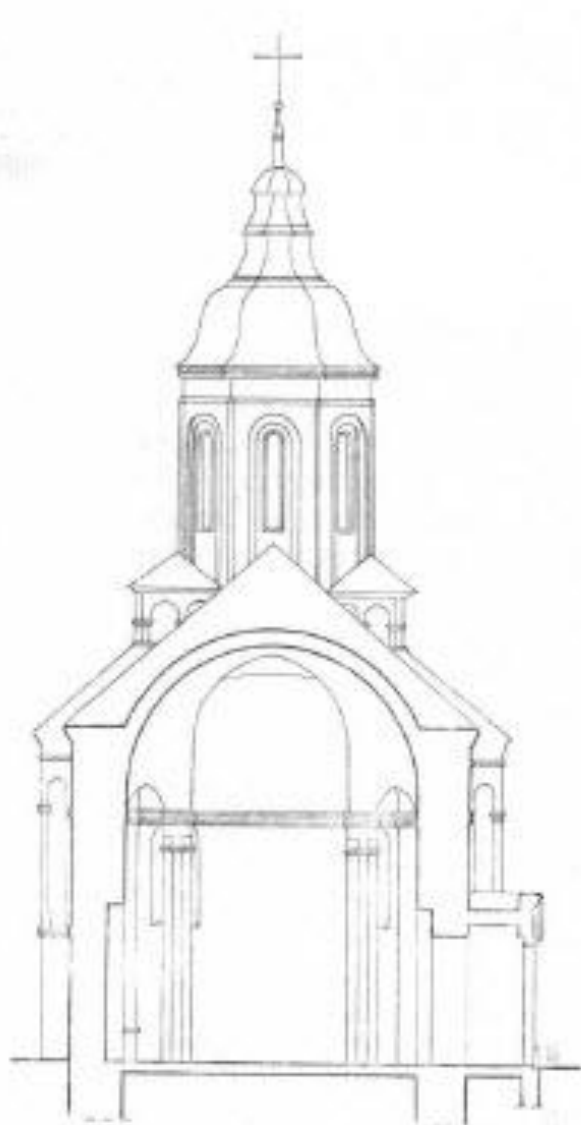
Цртеж 7. Подужни пресек (запад—исток) Горње цркве у Сремским Карловцима (данашње стање) Dessin 7. Section longitudinale (ouest-est) de l'église (état actuel).
