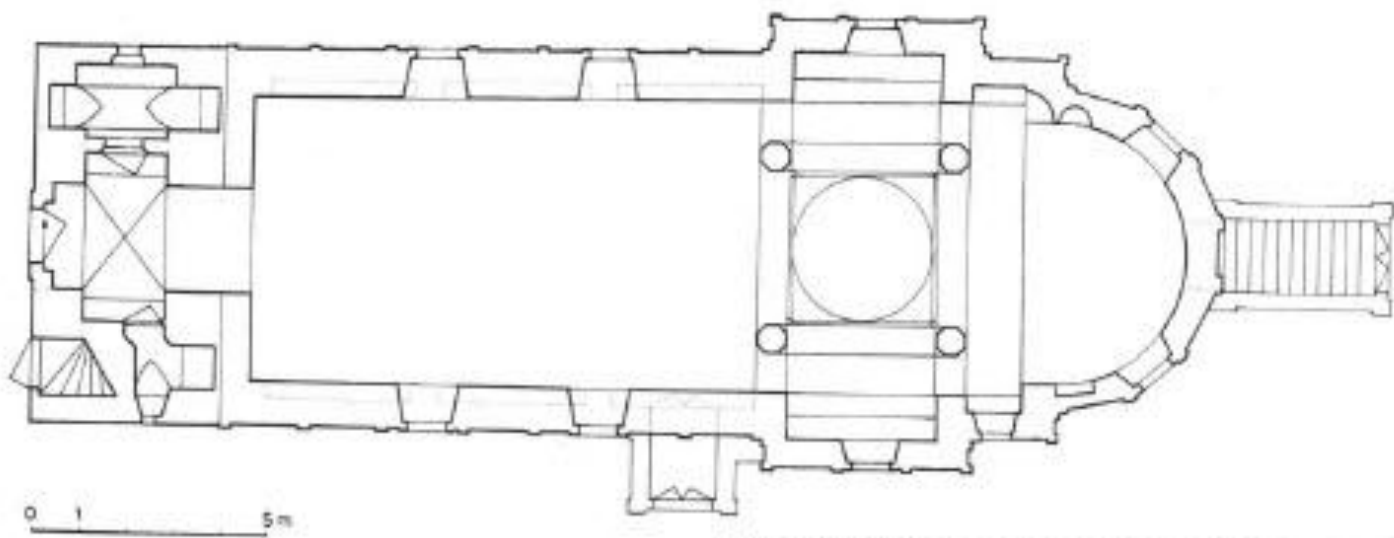
Цртеж 4. Основа Горње цркве у Сремским Карловцима (данашње стање)
