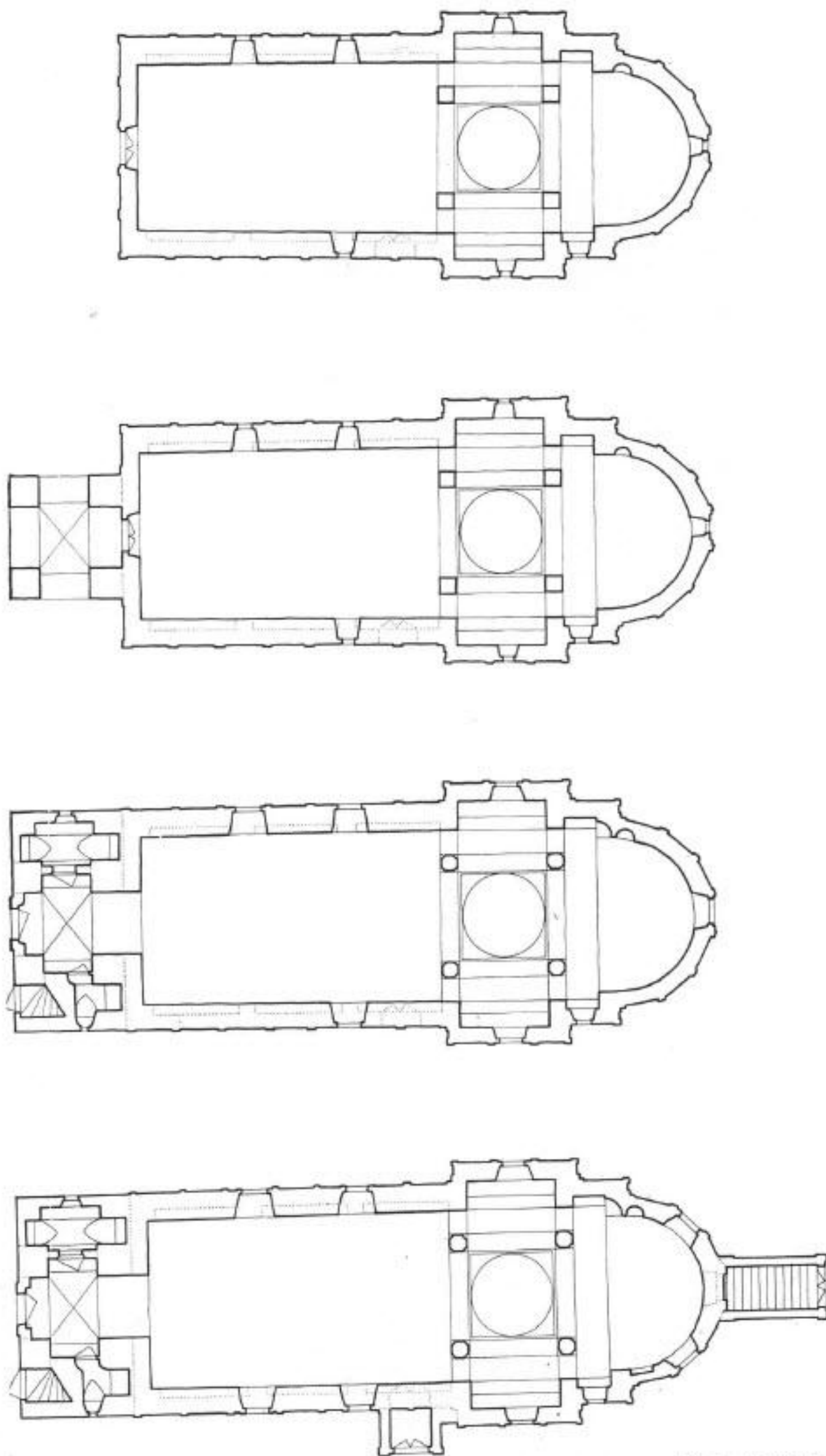
Цртеж 17. Упоредна табла основа Горње цркве у Сремским Карловцима: а) од времена настанка до почетка XVIII века, б) од 1718—31. до 1746. год., в) од 1746. до 1898. год. и г) од 1898. год. до данас.
