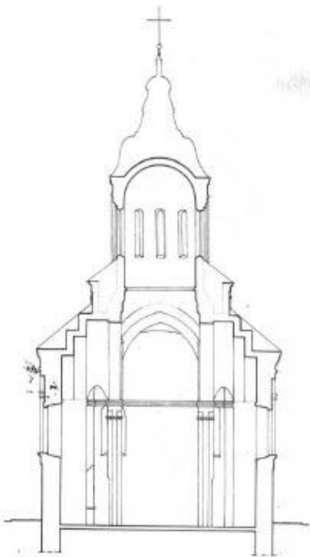
Цртеж 6. Попречни пресек (кроз припрату) Горње цркве у Сремским Карловцима (данашње стање) Dessin 6. Section transversale de l'église coupant le narthex (état actuel)
