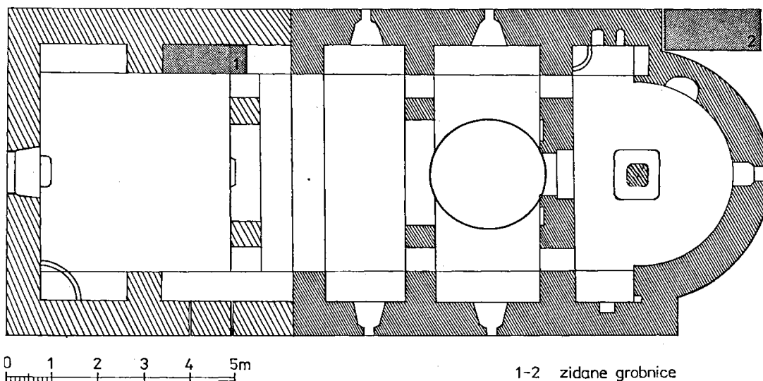
Цртеж 1. Црква манастира Подмалинско, основа
