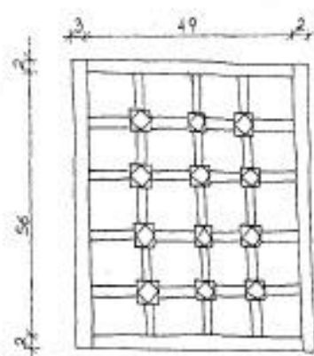
ПРОЗОР НА ИСТОЧАНОМ ЗИДУ СА ДРВЕНОМ МРЕЖОМ
