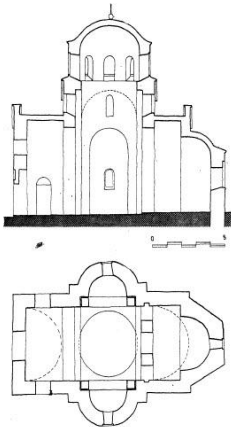
Сл. 4. Идеална реконструкција основе и пресека Богородице Топличке после њене средњовековне обнове
