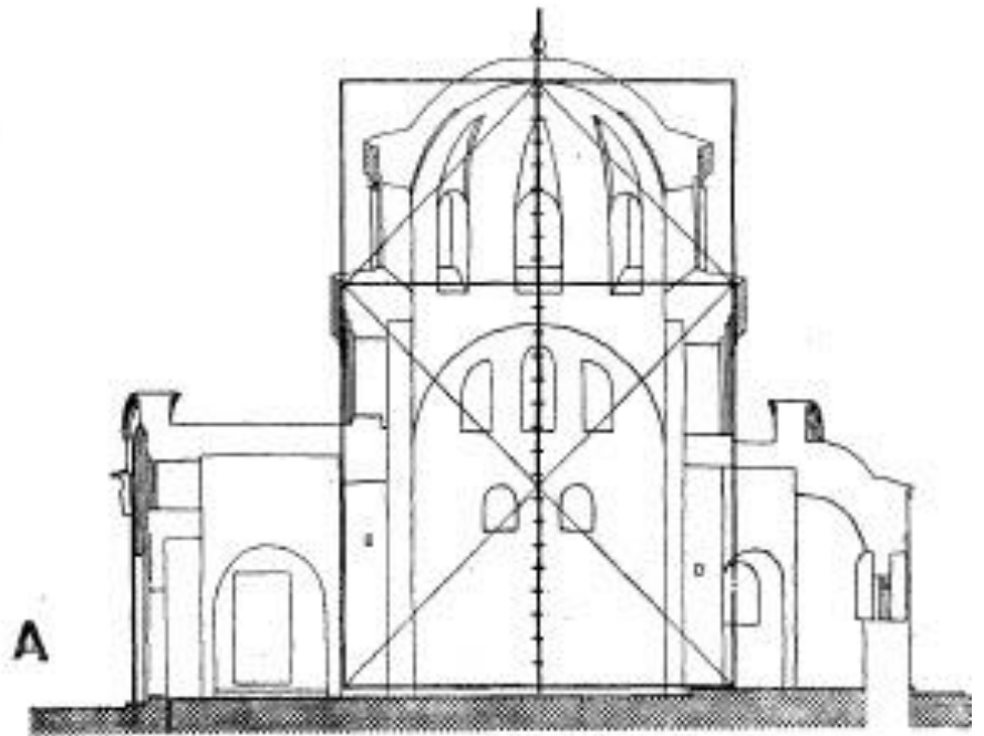
Сл. 5. Сразмере куполних делова трију најстаријих Немањиних задужбина (А. Свети Никола Топлички; В. Света Богородица Топличка; С. Свети Ђорђе у Расу)
