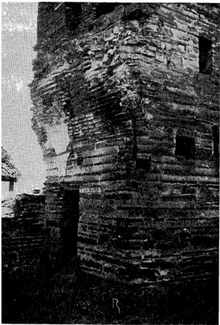
Сл. 7. Начин покривања малтером сваког другог уученог реда од опека, детаљ са јужне куле Светог Николе, снимак Б. Бошковића Fig. 7. La manière d'étaler le mortier sur chacun des rangs en retrait alternant avec des rangs en saillie; détail de la tour méridionale. Vue prise par Đ. Bošković
