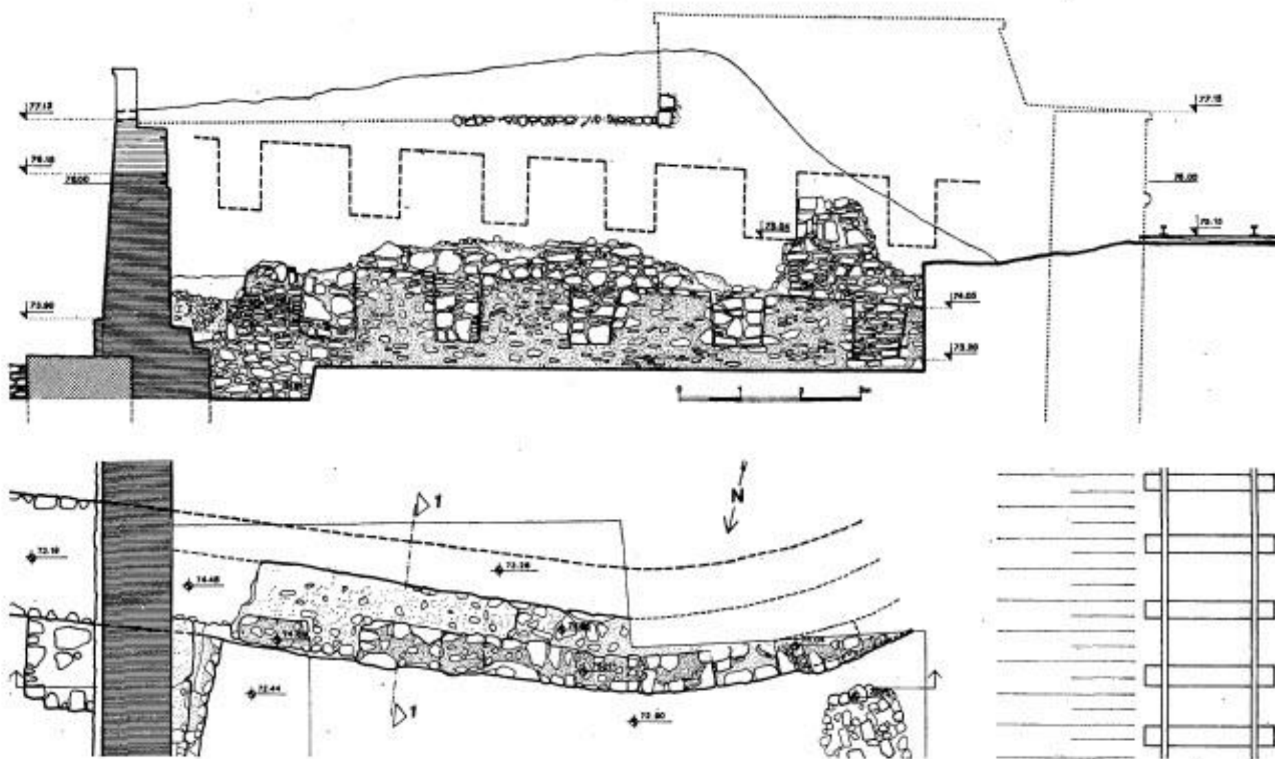
Сл. 12. Северни бедем савског пристаништа у Западном подграђу (сонда 5/82) — основа и изглед београда са пресеком кроз Приобални бедем
