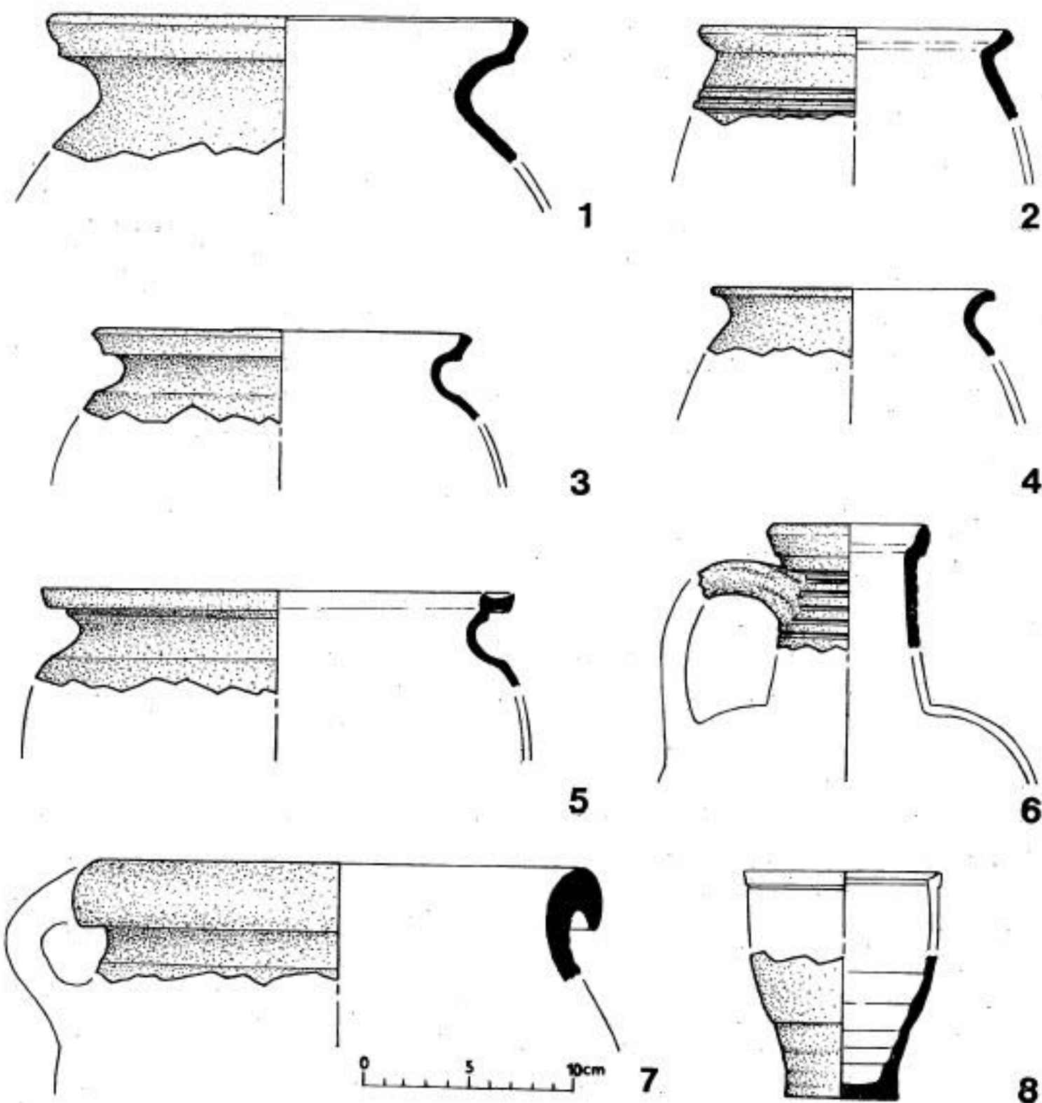
Сл. 6. Налази керамике из насипног слоја у простору А сонде 2/82 (цртежи Ј. Шарп)
