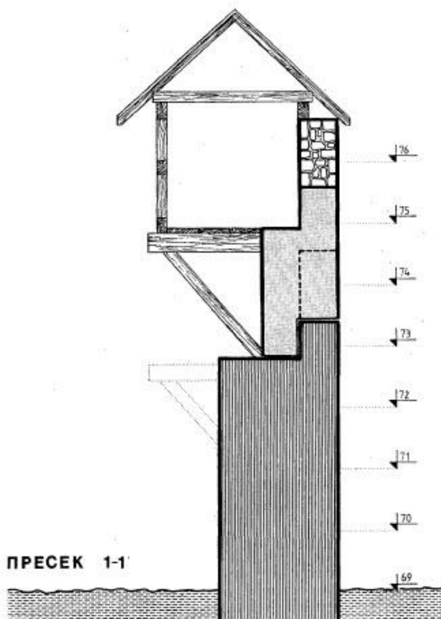
Сл. 13. Северни бедем савског пристаништа у западном подграђу — реституција пресека са старијом и млађом фазом Fig. 13. Muraille septentrionale du port de la Save dans le Faubourg occidental — restitution de la coupe comportant la phase ancienne et la phase moins ancienne
