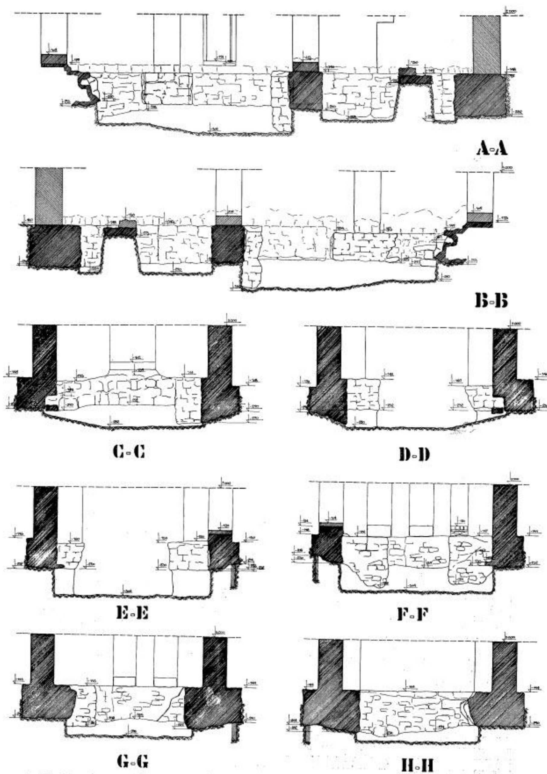
Fig. 7b. Coupes des fondations
