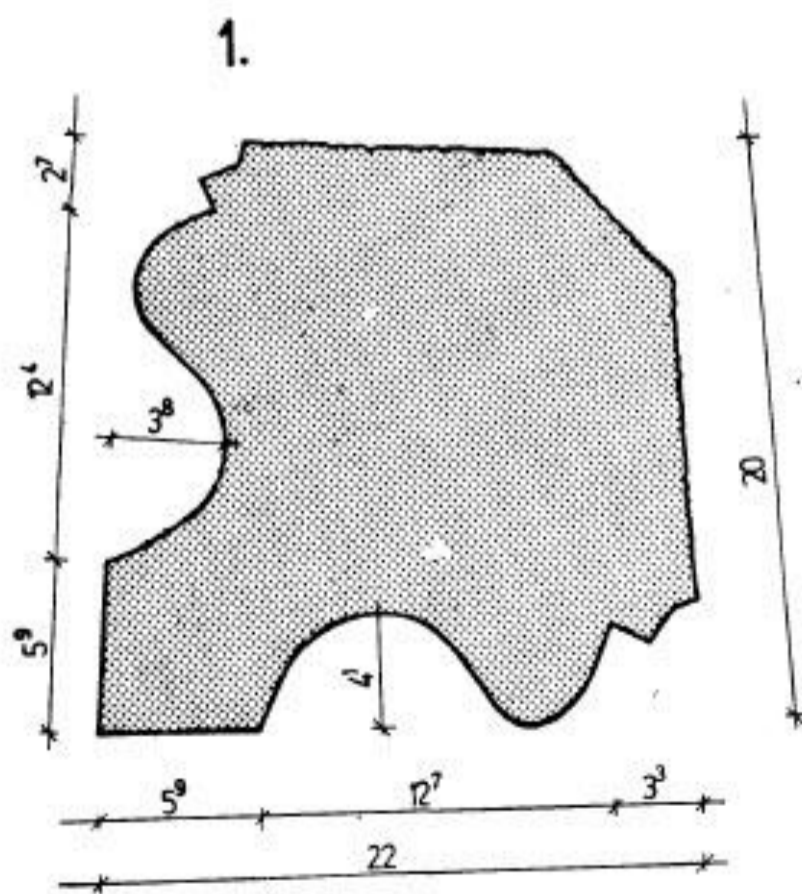
Сл. 4. Могући изглед саркофага светог Саве и детаљ профила
