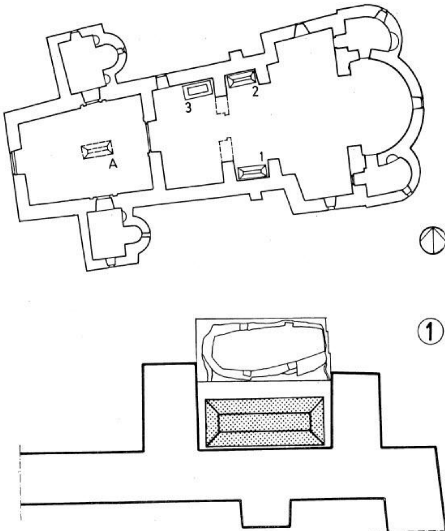
Fig. 5. Position présumée du sarcophage du roi Vladislav dans l'église du monastère de Mileševa et détail du caveau de ce roi. 1. Sarcophage du roi Vladislav, 2. Sarcophage d'un parent du roi Vladislav, 3. Châsse de Saint Sava, A. Sarcophage de Saint Sava
