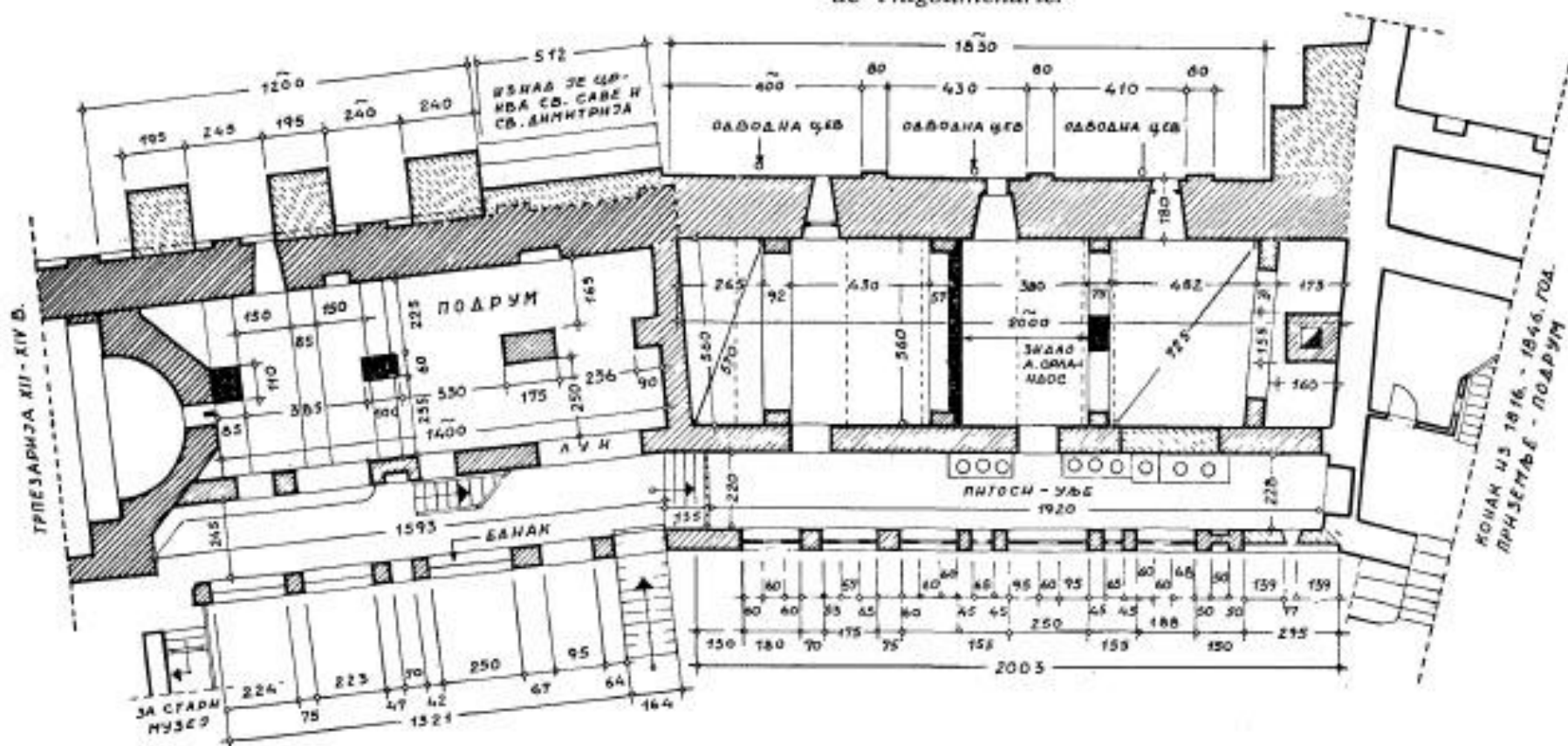
Fig. 5. Plan de la cave de la partie sud de l'igouménarie au monastère de Hilandar et de la boulangerie située dans la cave de la partie nord de l'igouménarie.
