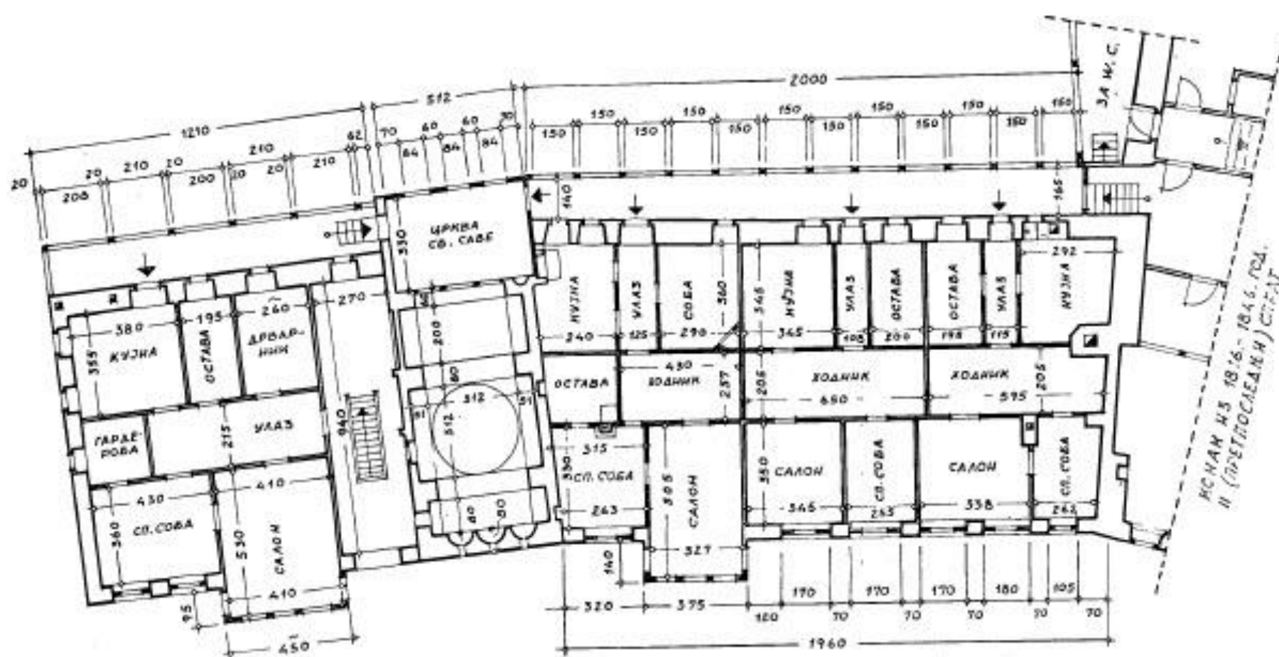
Fig. 9. Plan du quatrième étage de l'igouménarie au monastère de Chilandar
