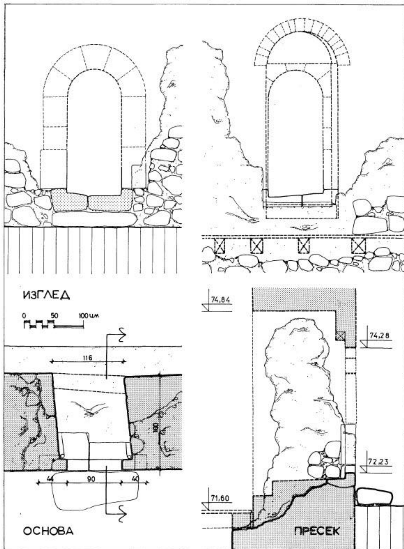
Fig. 8. Vestiges originaux du portail donnant accès au rez-de-chaussée du palais et la reconstitution de l'aspect présumé
