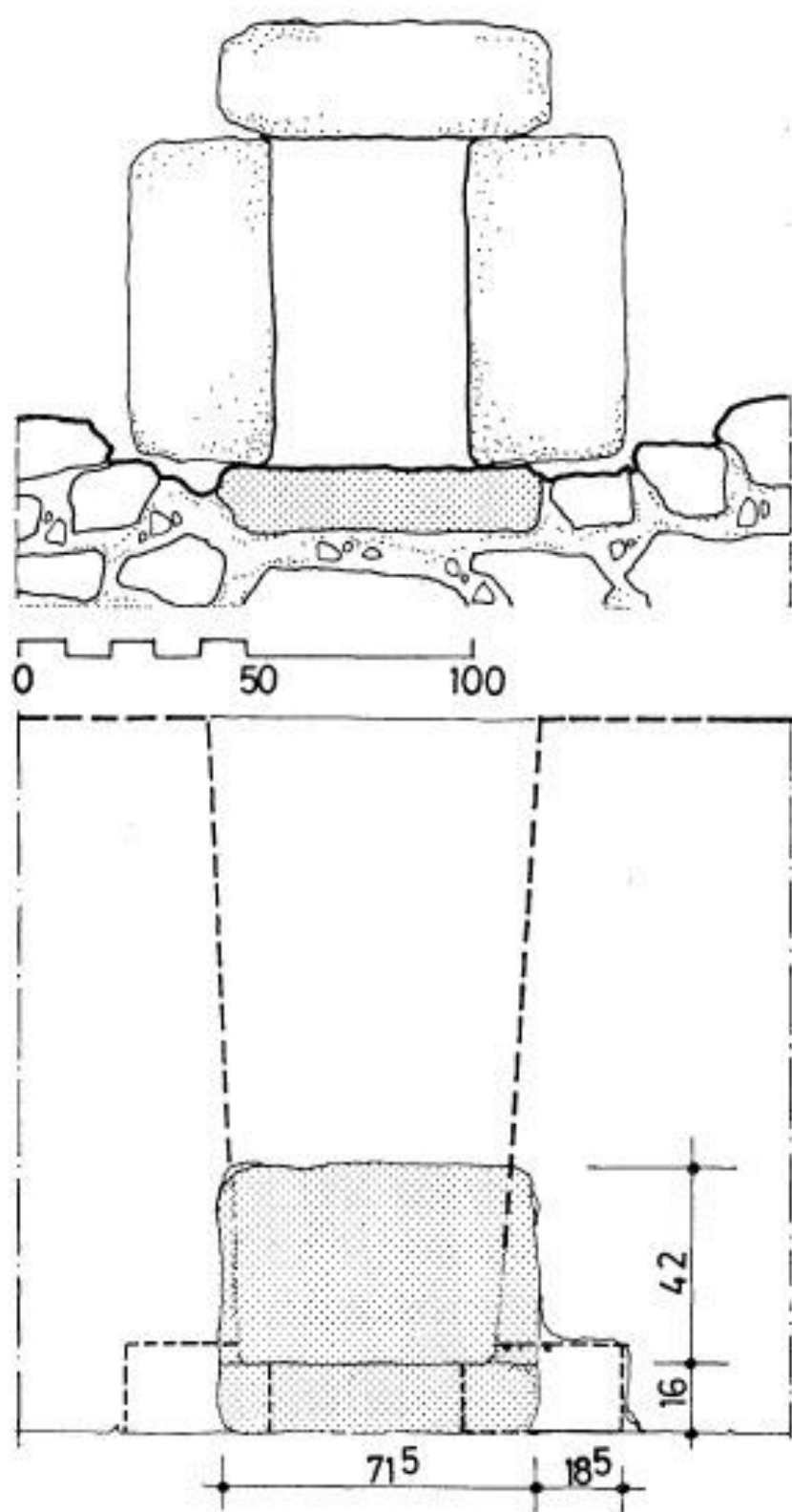
Сл. 9. Остаци каменог оквира прозора у приземљу грађевине и претпостављени првобитни изглед
