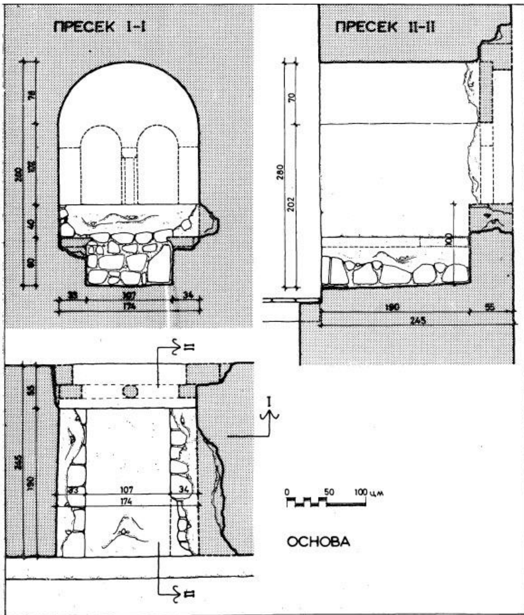
Fig. 10. Niche munie de fenêtre au rez-de-chaussée du palais et reconstitution de l'aspect primitif
