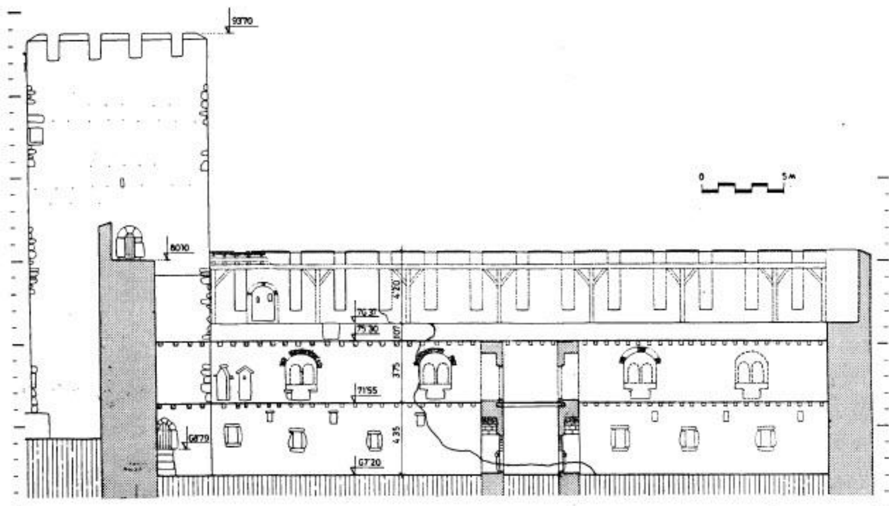
Fig. 13. Coupe transversale du palais et reconstitution de la construction primitive
