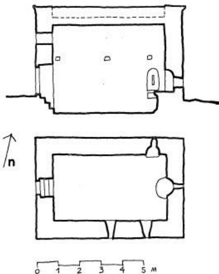
Сл. 23. Коритник, црква Св. арханђела Михаила, основа и подужни пресек
