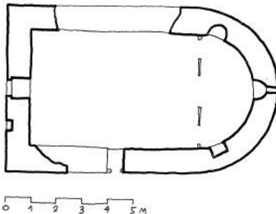
Сл. 38. Средња Река, основа цркве
