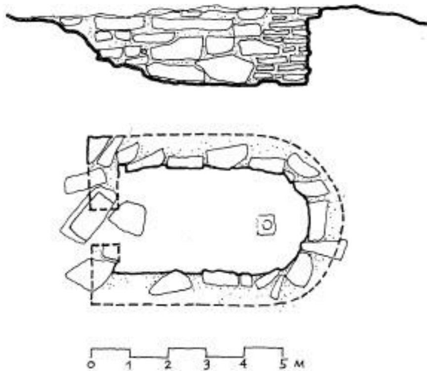
Сл. 30. Палеж, Горња црква, основа и подужни пресек
