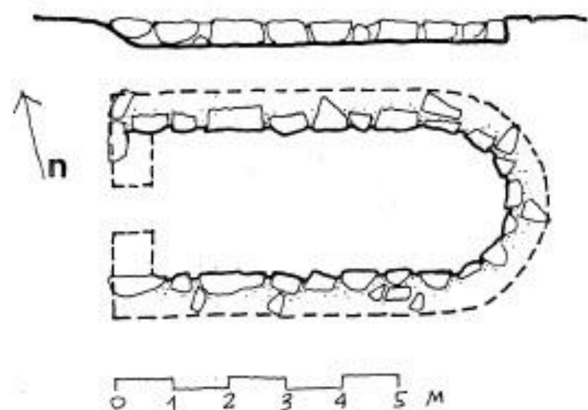
Сл. 3. Белобраћа, основа и подужни пресек цркве
