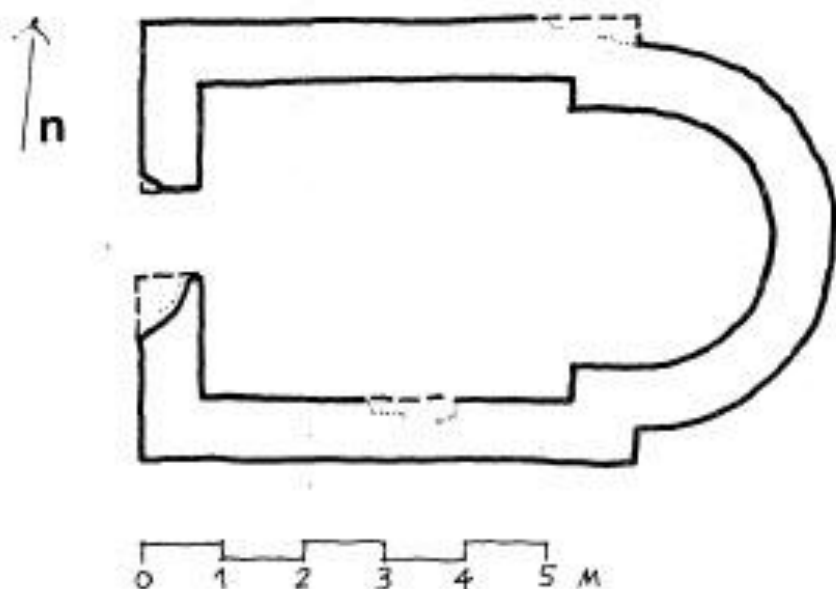
Сл. 2. Бажалице, основа цркве
