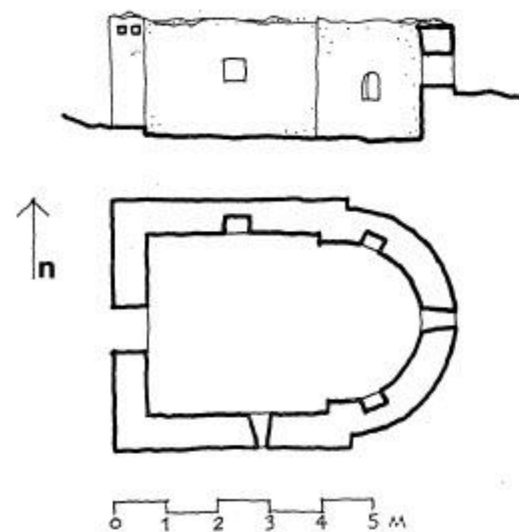
Сл. 25. Косурићи, црква Св. Катарине, основа и подужни пресек
