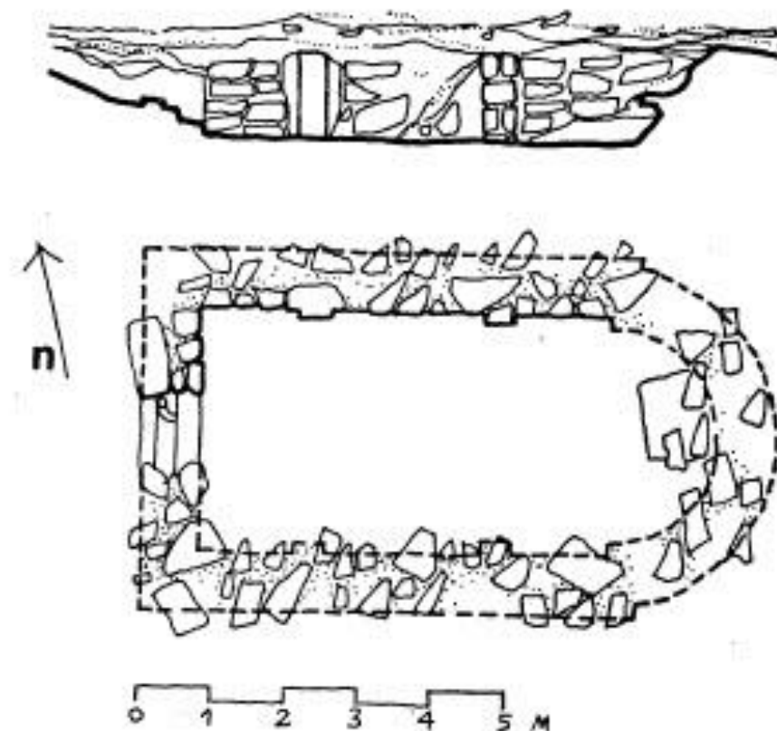
Сл. 17. Доњи Перишићи, црква Св. Спиридона, основа и подужни пресек
