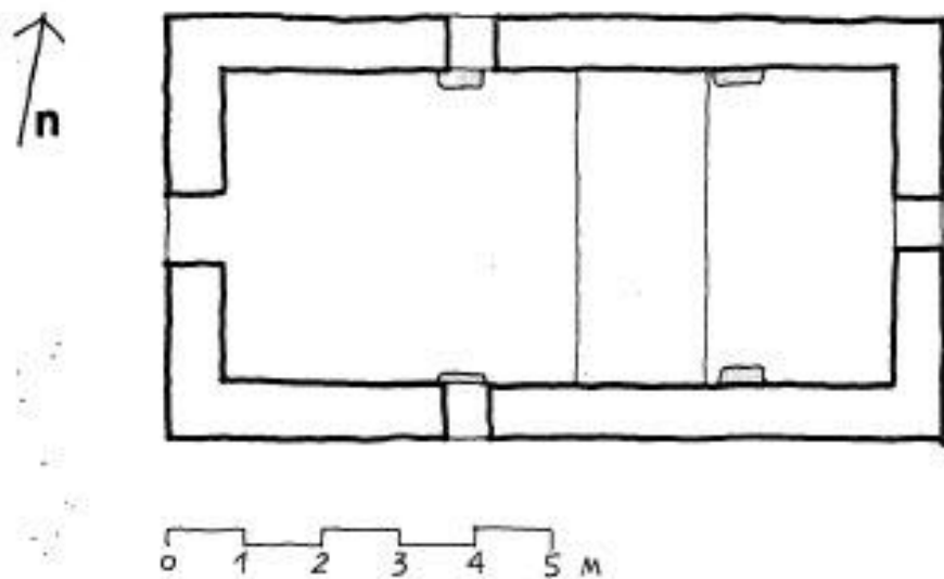
Сл. 21. Карадак, црква Св. Ане, основа
