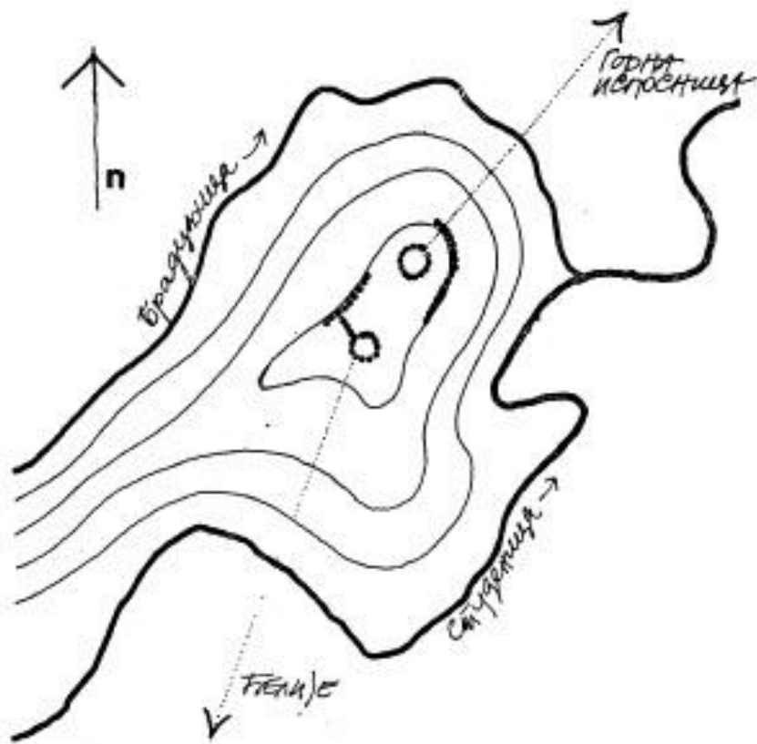
Сл. 47. Придворица, Јеринин град, ситуациона скица утврђења
