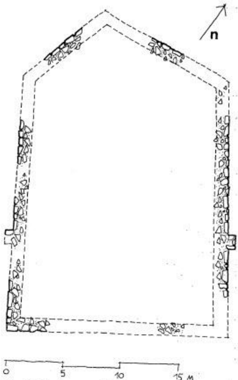
Сл. 49. Придворица, Ђелије, основа беодема
