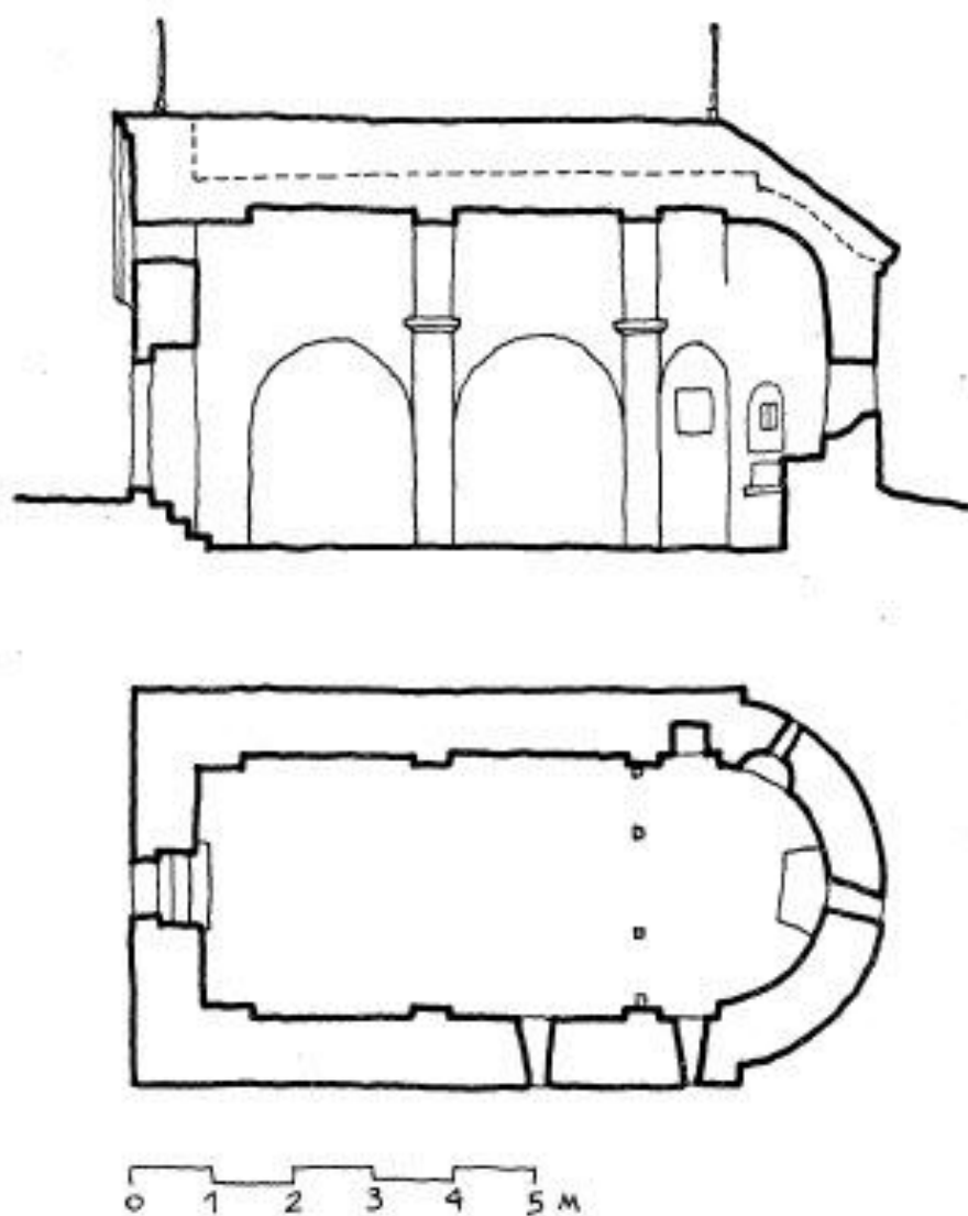
Сл. 28. Остатија, црква Св. Кузмана и Дамјана, основа и подужни пресек
