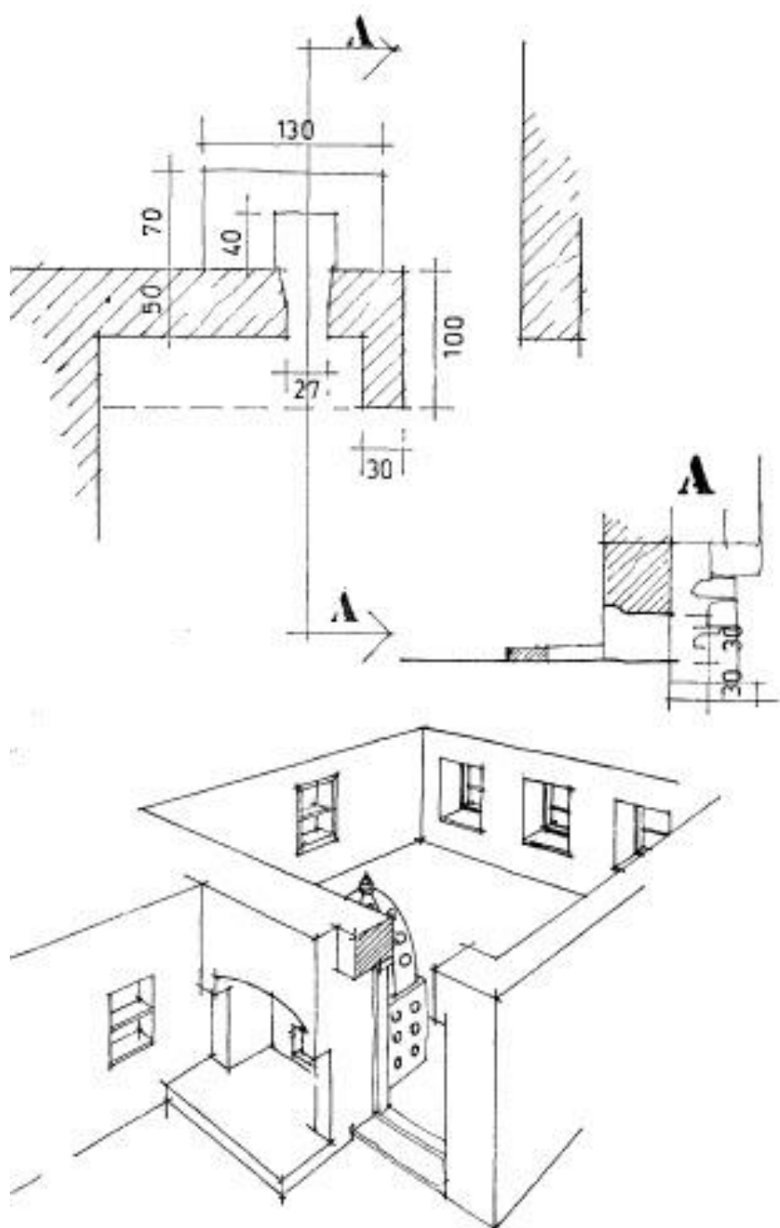
Сл. 16. Основа и пресек ложишта пећи откопане у рушевинама конака манастира Милешева
