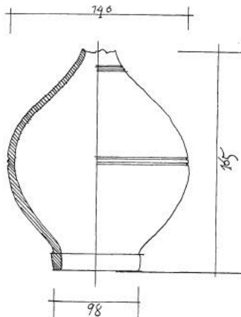
Сл. 10. Завршни лонац са пећи откривене у рушевинама конака манастира Милешево, XVII век
