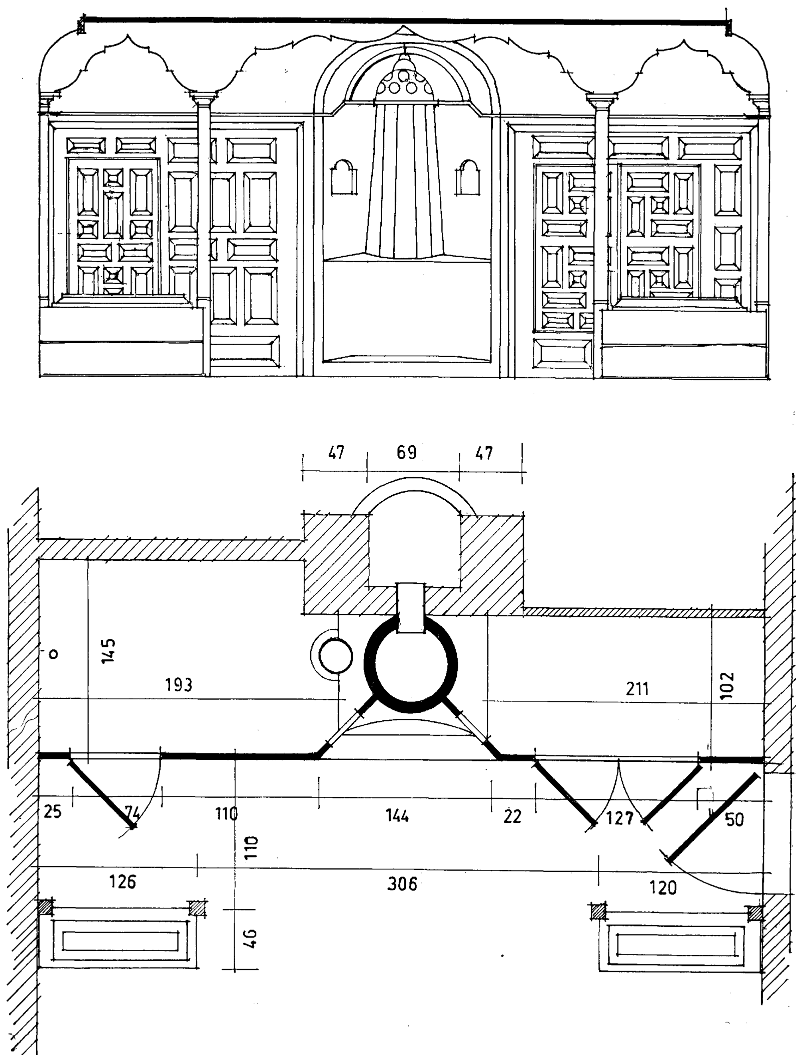
Сл. 24. Новије решење улаза у собу — пећ, купатило и плакар за постељину
