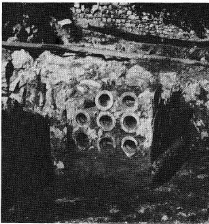
Сл. 15. Остаци пећи из коначи манастира Сопоћани, пре 1689. године, фото О. Кандић
